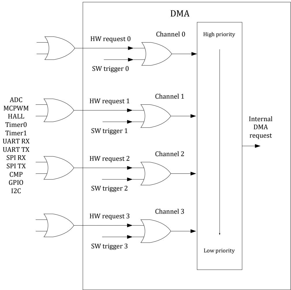
图 17-6 DMA 通道优先级
