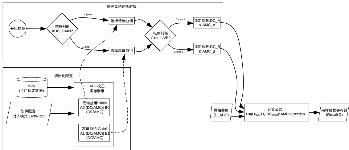
图 12-3 ADC 校正处理流程图
