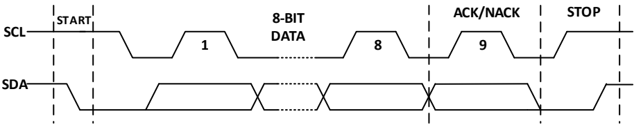
图 9-2 基本 I2C 传输时序图
