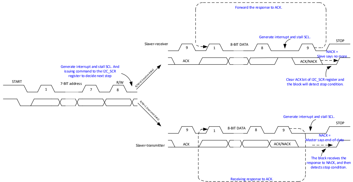
图 9-5 从模式传输示意图
