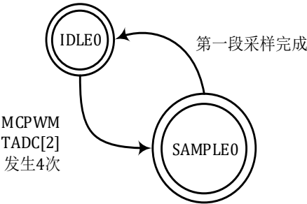
图 12-6 ADC 单段采样状态转移图
