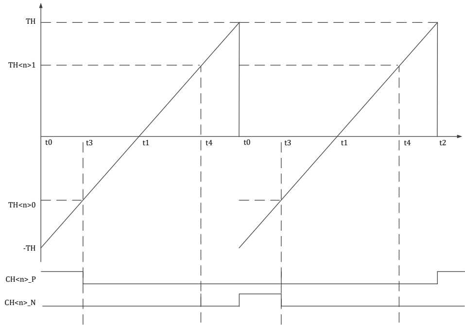
图 14-11MCPWM 时序 TH<n>0 和 TH<n>1 边沿对齐推挽模式
