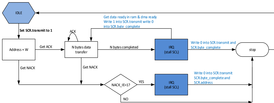
图 9-11 主模式下多字节发送示意图
