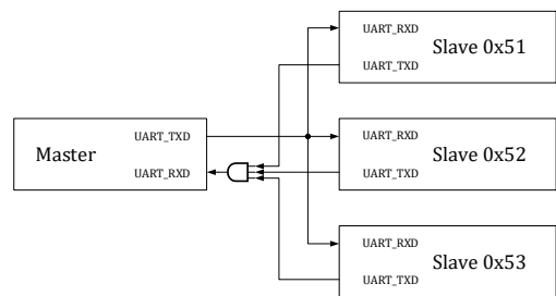
图 16-5 UART 多机通讯示例
