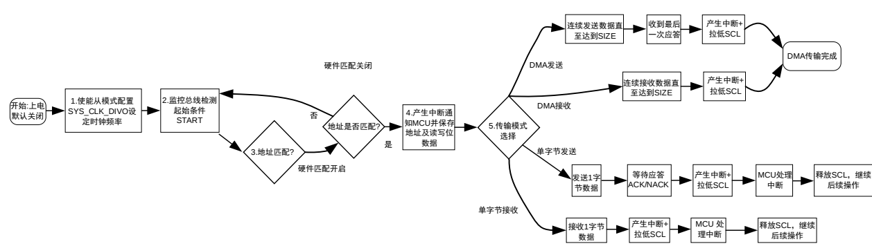
图 9-4 I2C 从模式工作流程图
