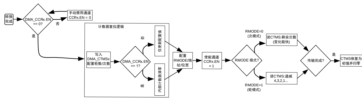
图 17-7 DMA 操作逻辑流程图
