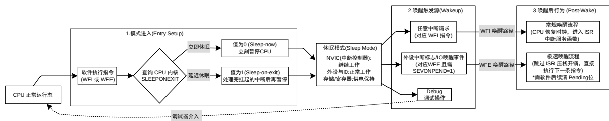
图 20-2 常规休眠模式进入与唤醒流程图
