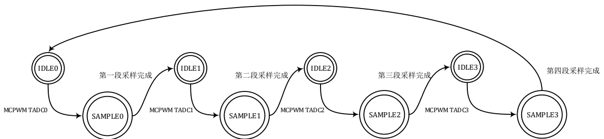
图 12-8 ADC 四段采样状态转移图
