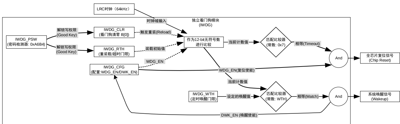
图 19-2 IWDG 工作原理和信号流向
