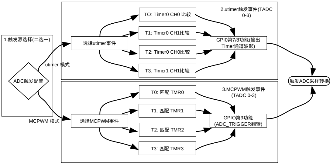
图 12-5 ADC 触发源选择与调试逻辑流程图
