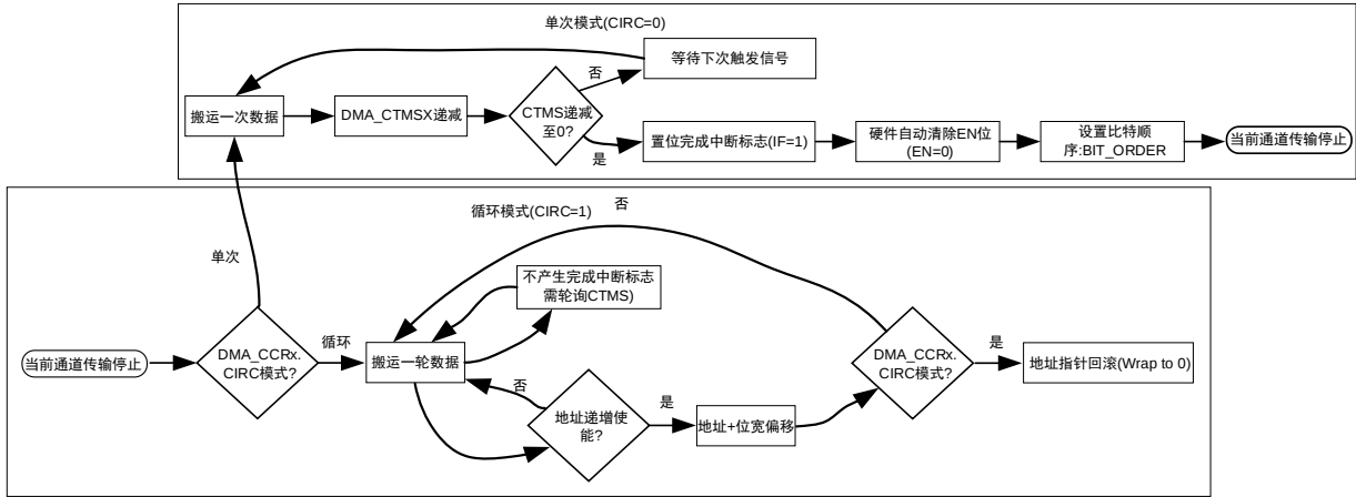
图 17-5 DMA 的循环模式和单次模式的逻辑流程图
