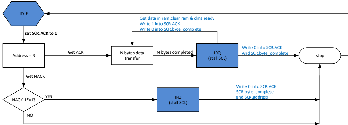
图 9-12 主模式下多字节接收示意图
