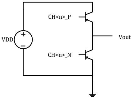
图 14-12MCPWM IO 控制示意图
