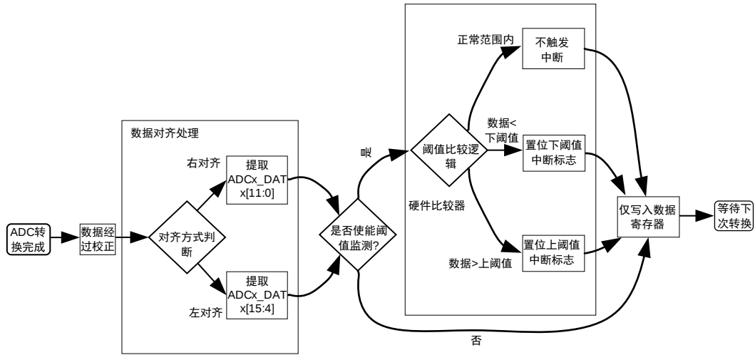
图 12-4 ADC 阈值比较流程图
