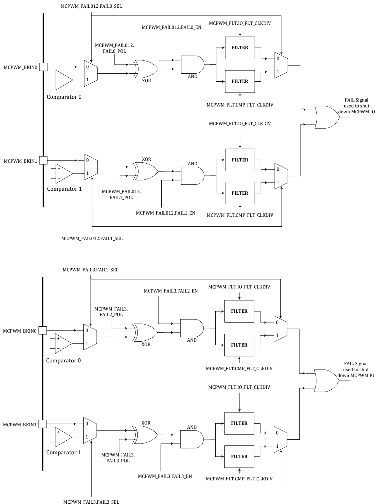
图 14-5 MCPWM FAIL 逻辑示意图
