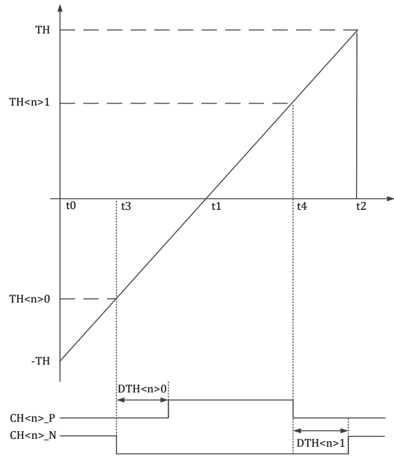
图 14-8MCPWM 时序 TH_{<n>0} 和 TH_{<n>1} -中心对齐模式
