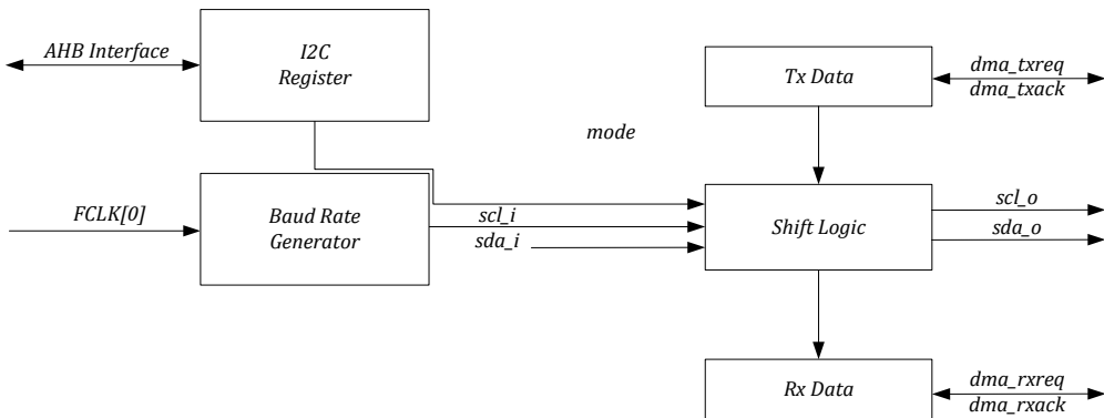
图 9-1I2C 模块顶层功能框图
