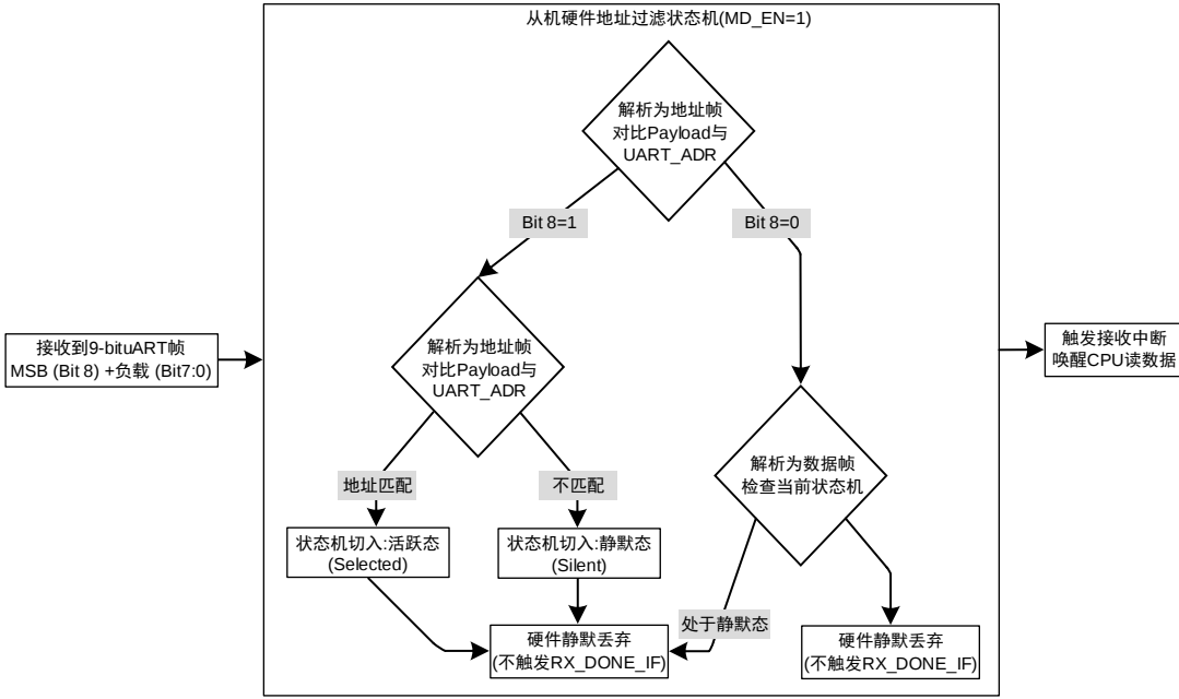
图 16-4 从机 9-bit UART 地址帧过滤状态机处理流程
