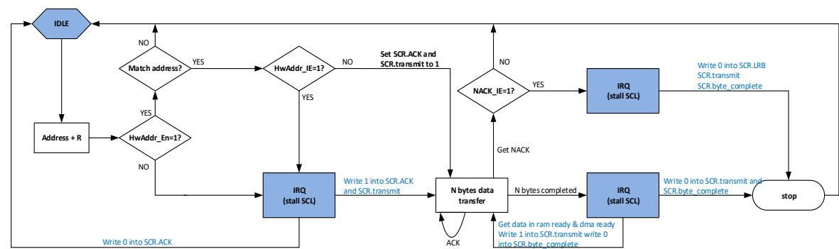
图 9-7 从模式下多字节发送示意图
