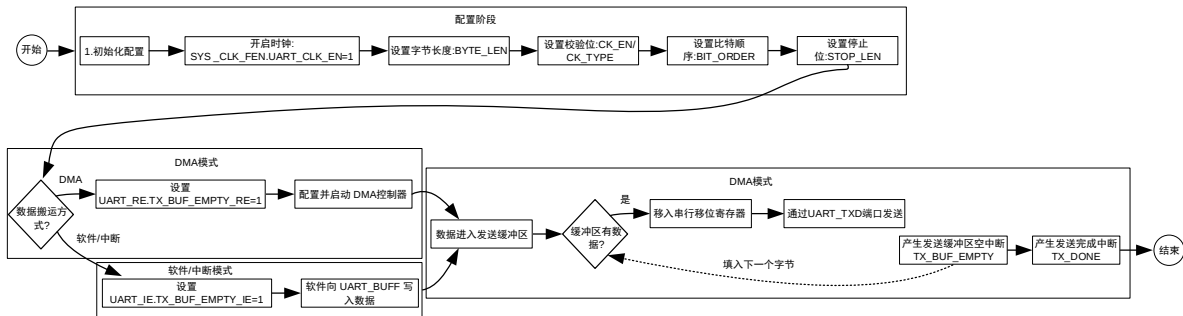
图 16-1 UART 发送流程和硬件机制
