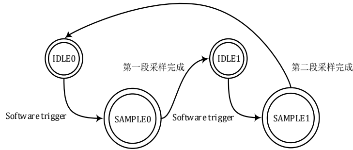
图 12-7 ADC 两段采样状态转移图
