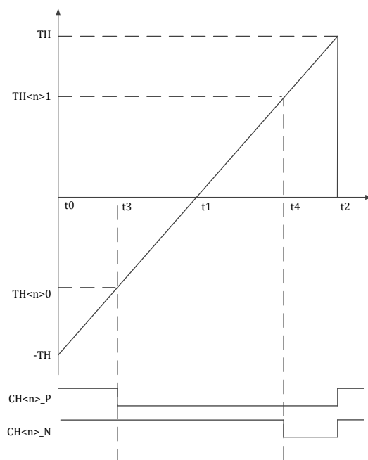
图 14-10MCPWM 时序边沿对齐模式
