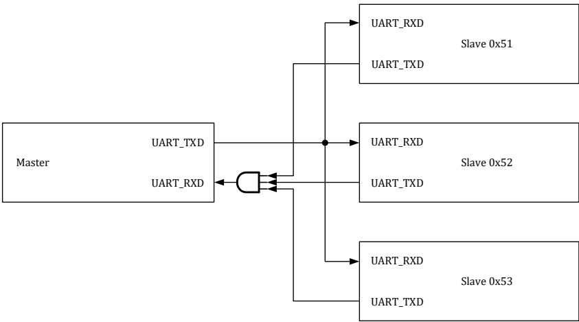
图 16-3 UART 多机通讯互联拓扑
