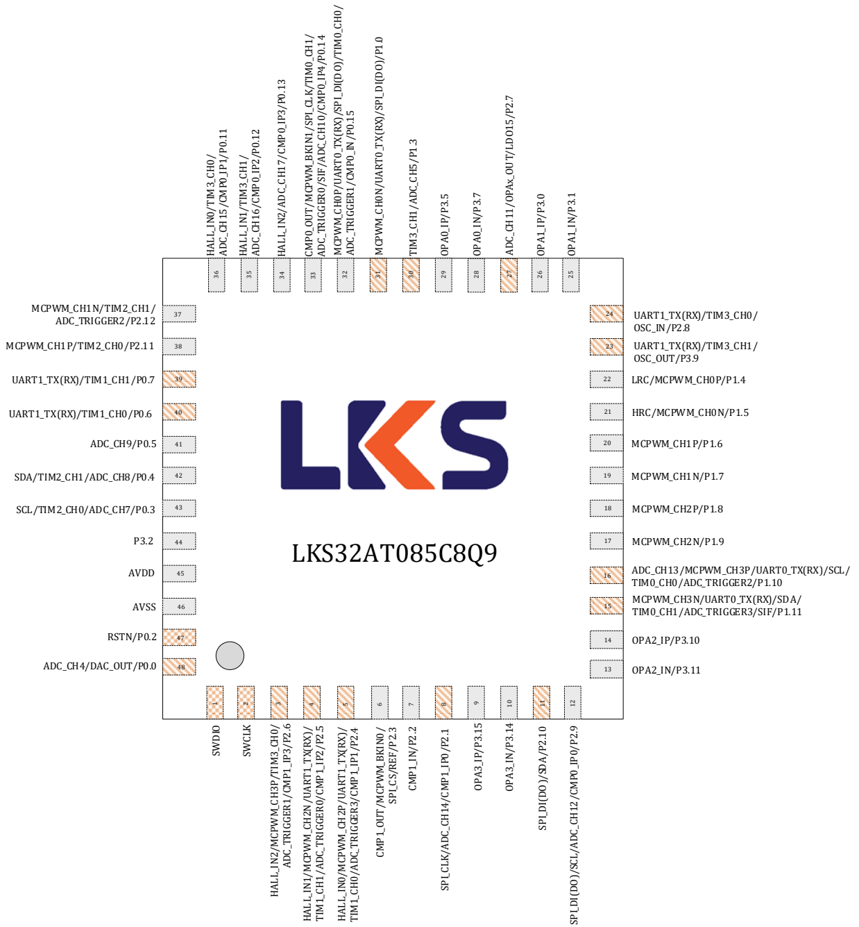
图 2-1 LKS32AT085C8Q9(B)管脚分布图
