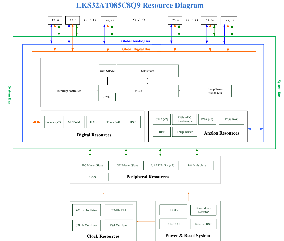
图 1-1 LKS32AT085C8Q9 系统资源框图
