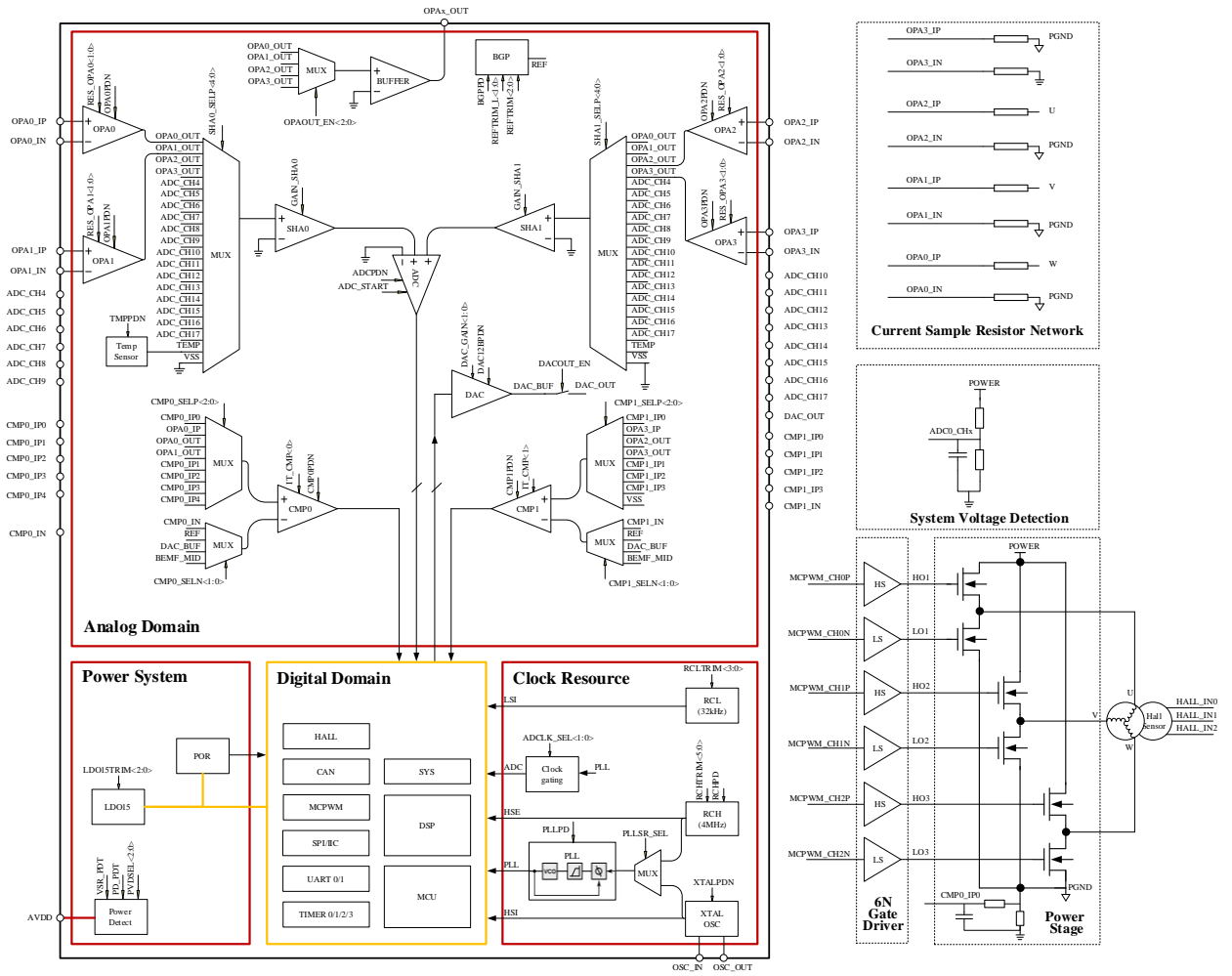
图 1-2 LKS32AT085 矢量正弦控制系统简化原理图
