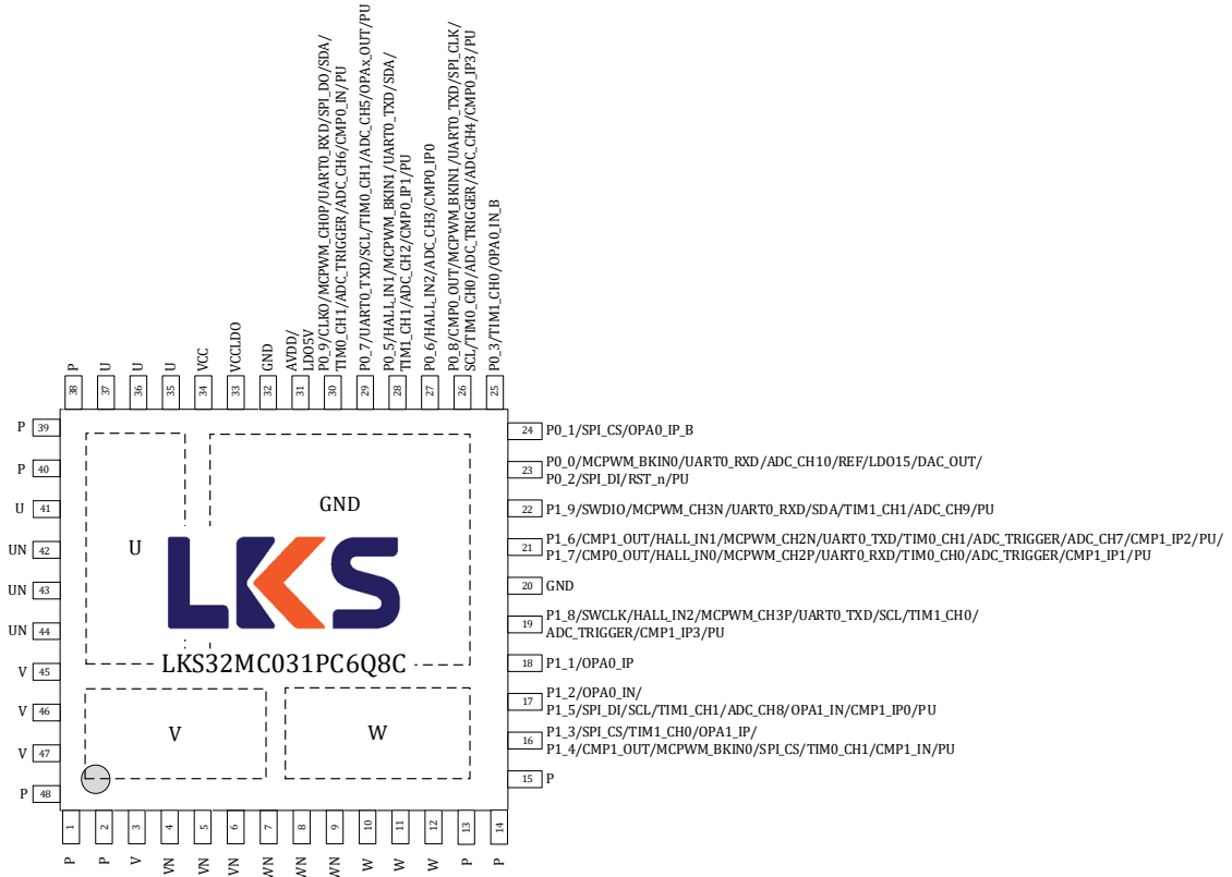
图 3-1 LKS32MC031PC6Q8C 管脚分布图
