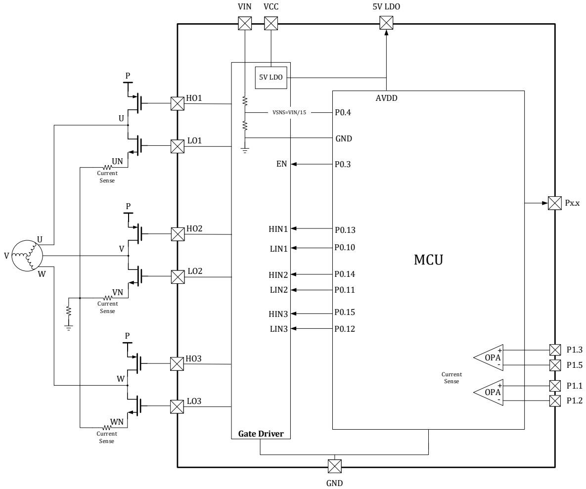
图 3-16 LKS32MC037FM6S8B(C)预驱连接示意图
