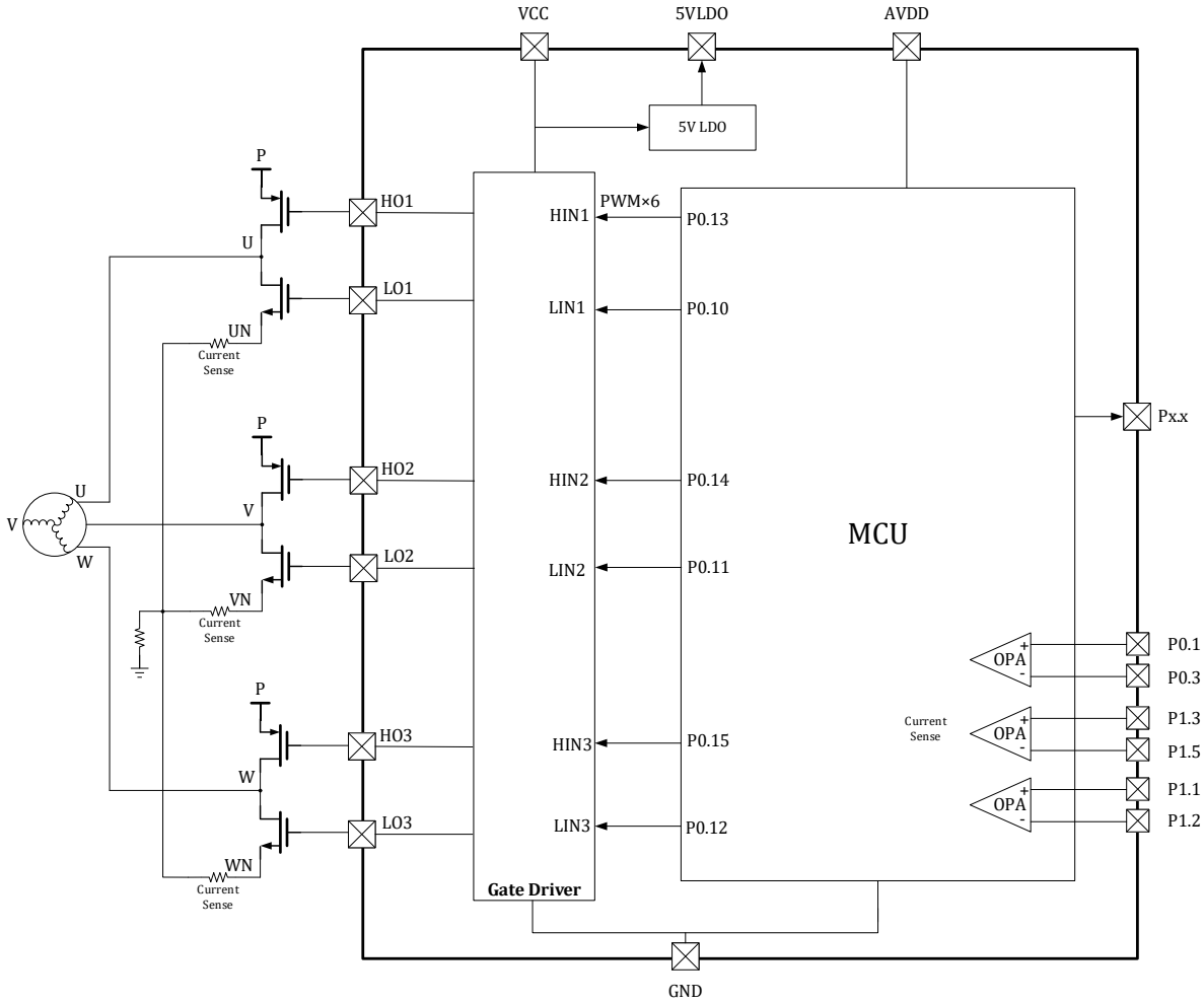
图 3- 24 LKS32MC039D2K6Q8C 预驱连接示意图
