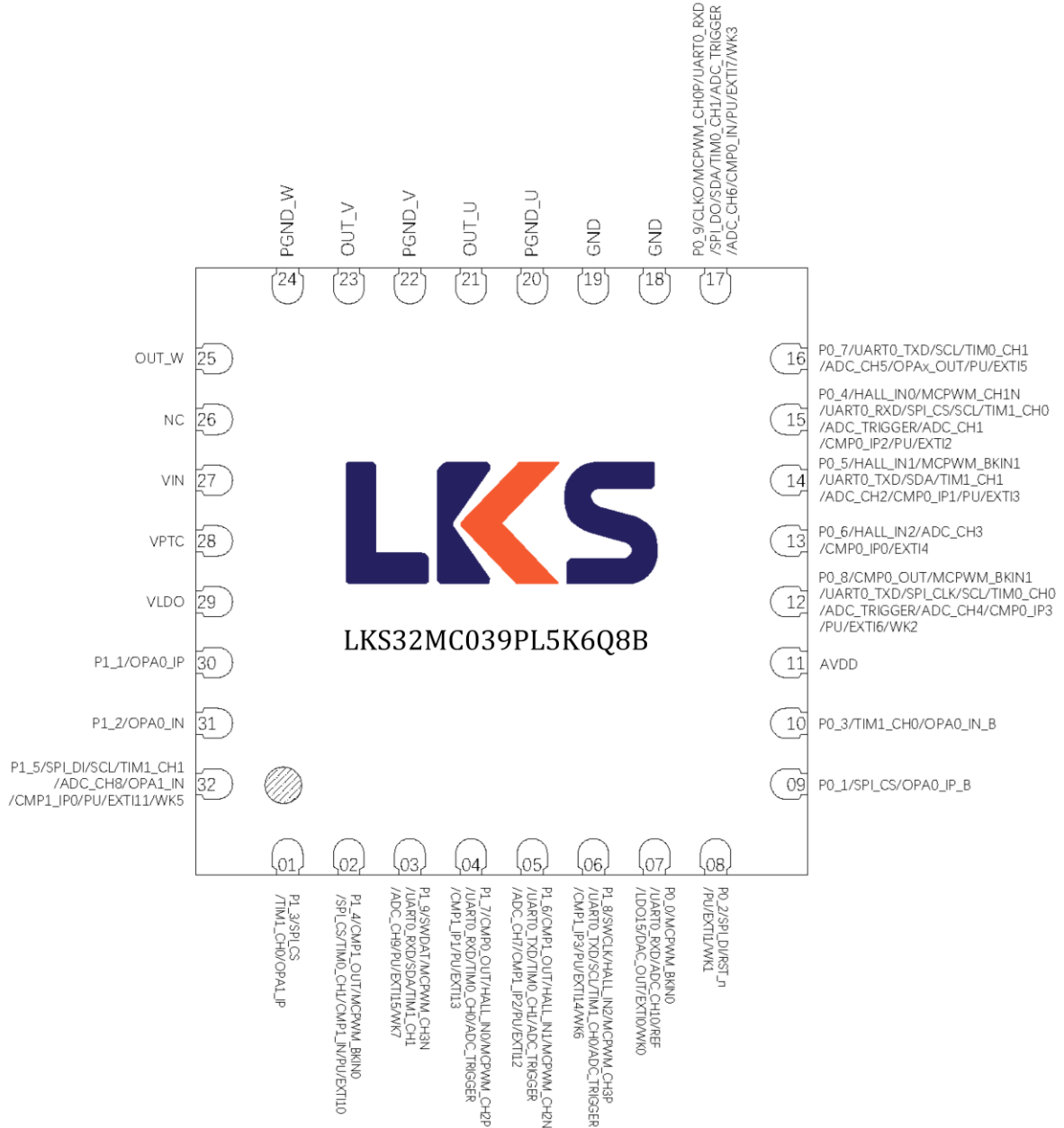
图 3- 25 LKS32MC039PL5K6Q8B(C)管脚分布图
