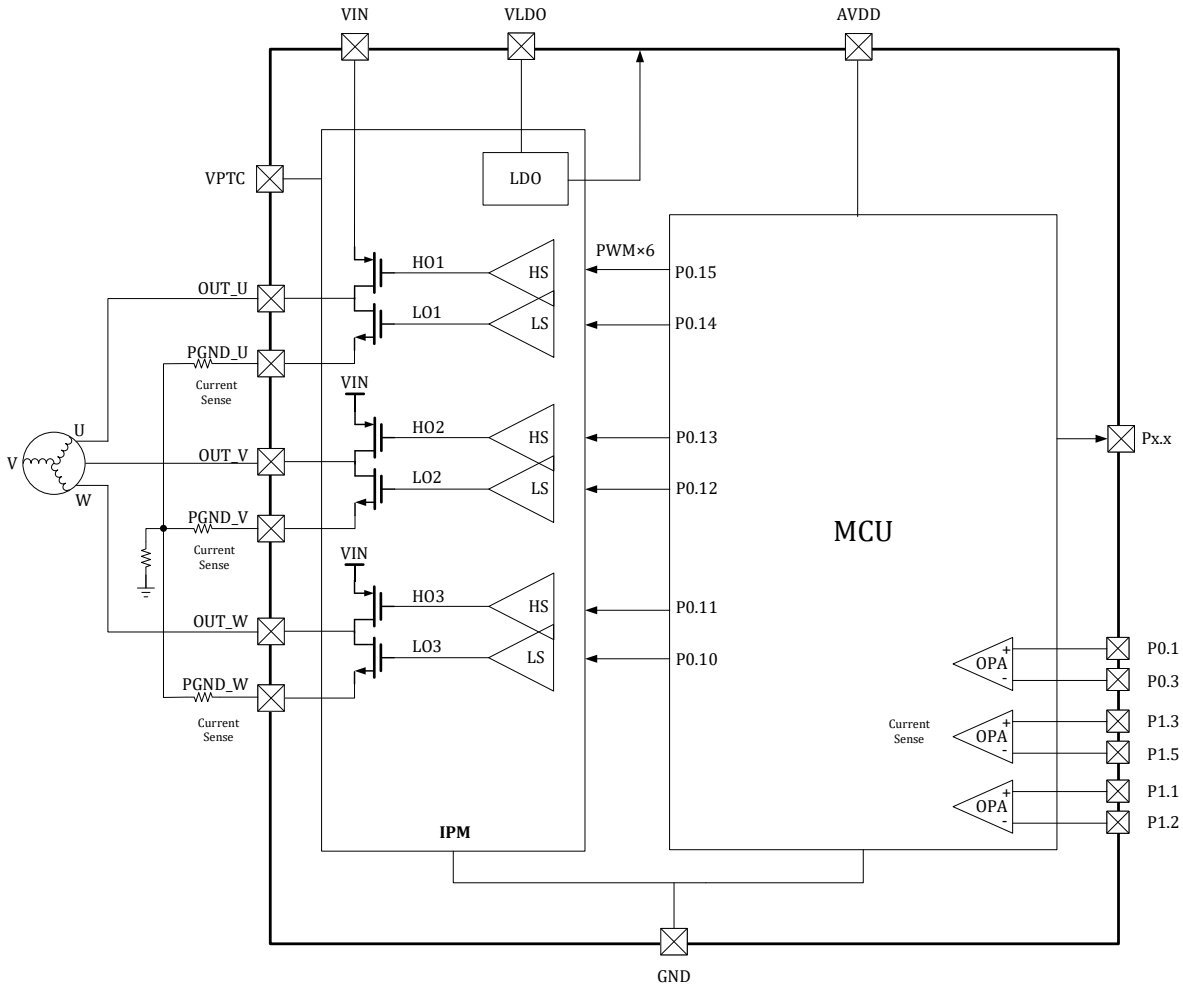
图 3- 26 LKS32MC039PL5K6Q8B(C) IPM 连接示意图
