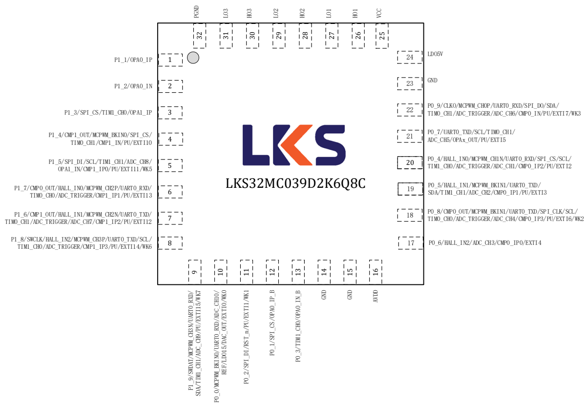
图 3- 23 LKS32MC039D2K6Q8C 管脚分布图
