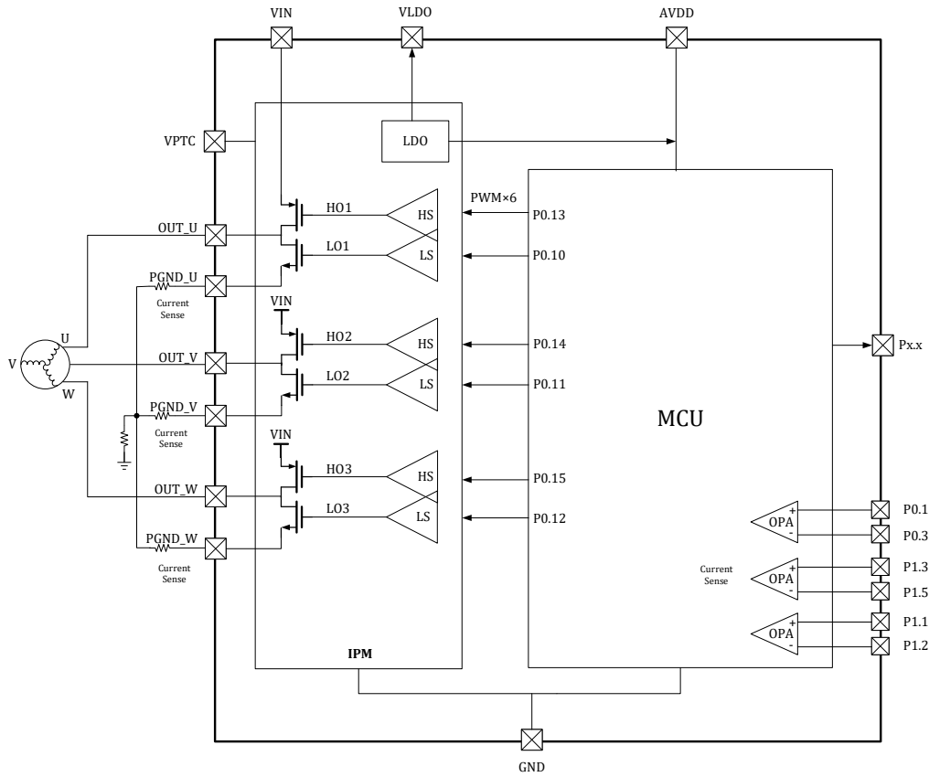
图 3- 28 LKS32MC039PL3K6Q8B IPM 连接示意图
