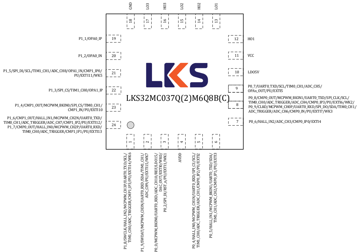
图 3- 19 LKS32MC037Q(2)M6Q8B(C)管脚分布图
