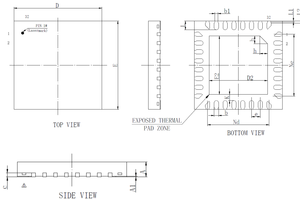
图 4-7 LKS32MC039PL3K6Q8C 封装图示
