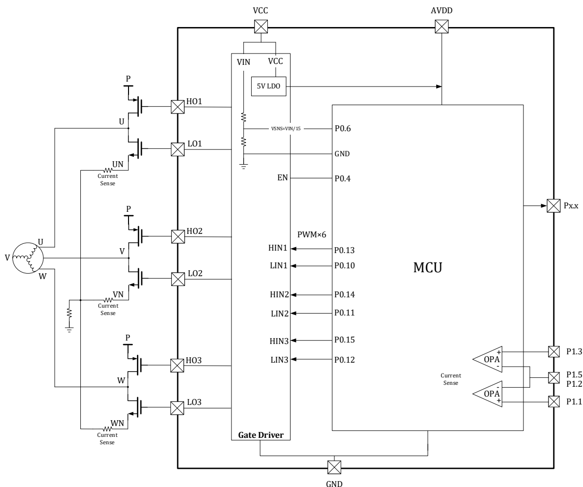
图 3-10 LKS32MC035EL6S8B(C)预驱连接示意图
