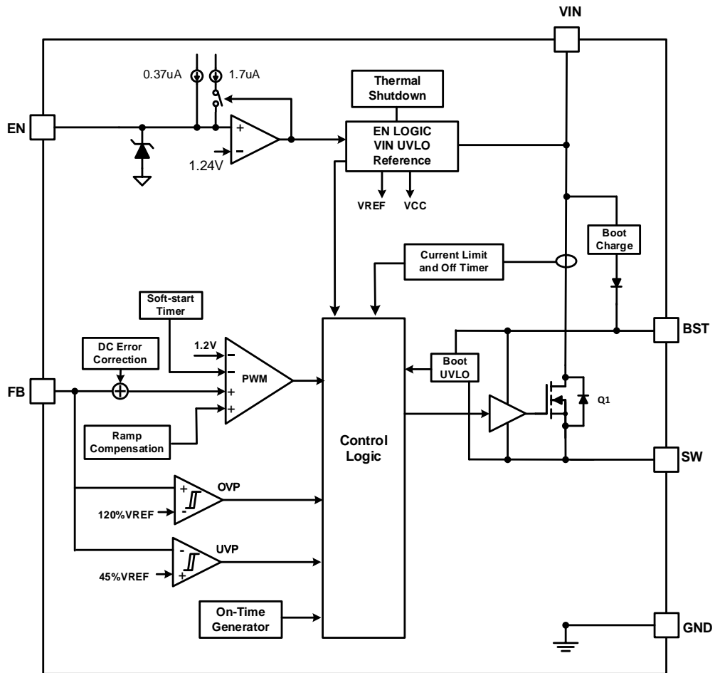
图 22-1 内部功能框图
