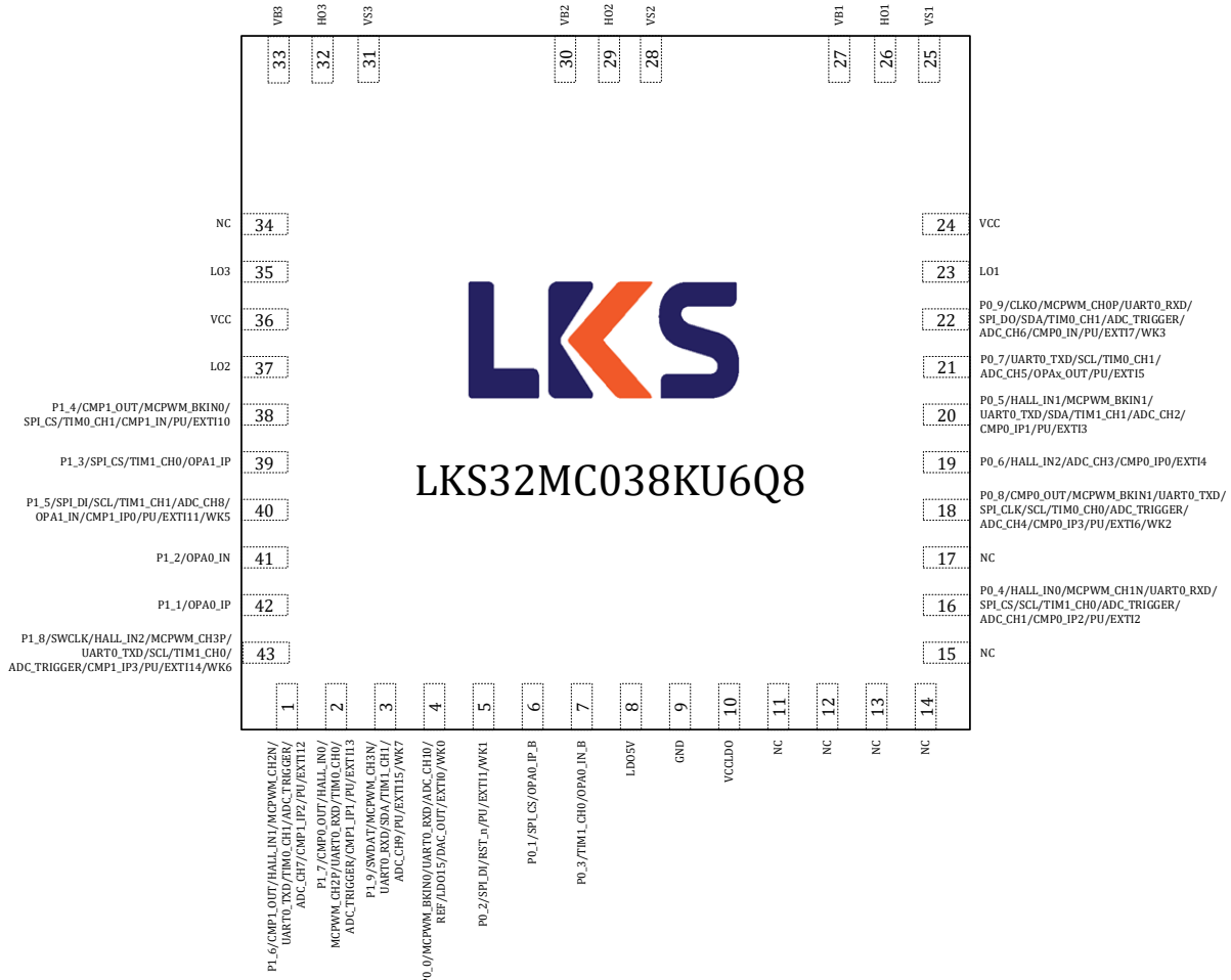
图 3-19 LKS32MC038KU6Q8B(C)管脚分布图
