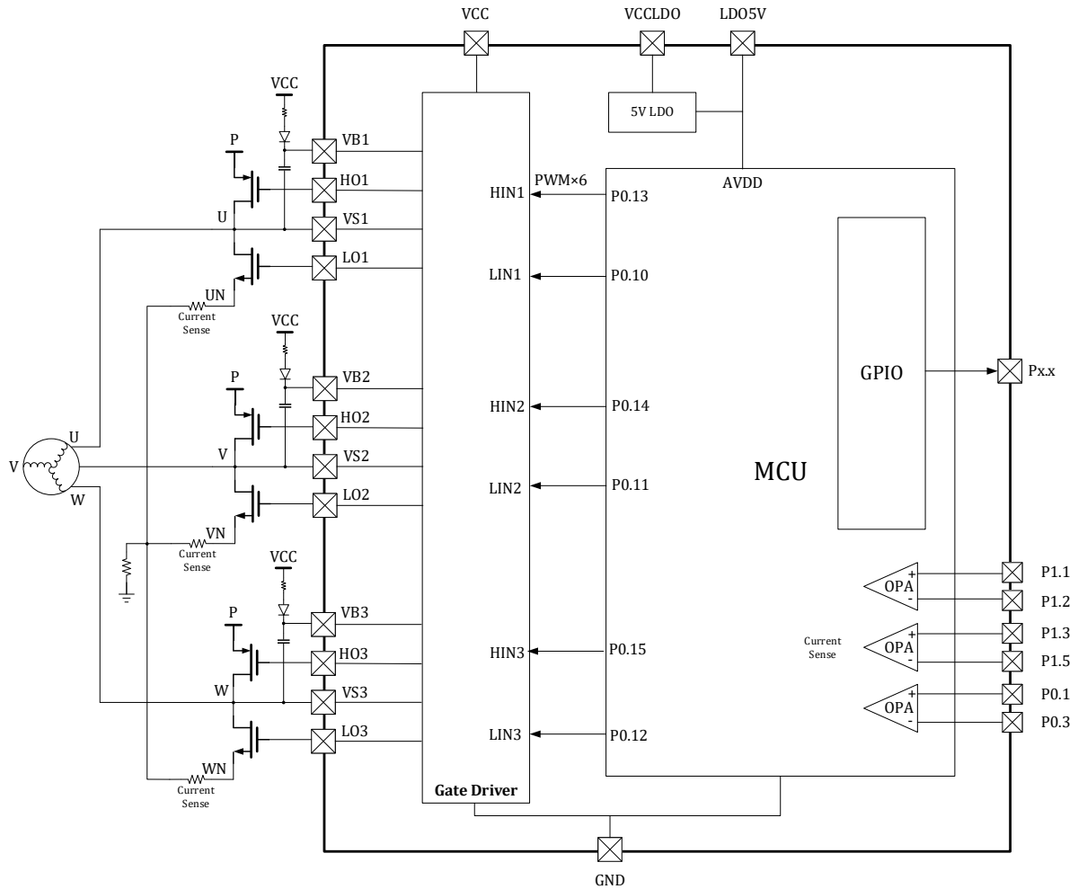
图 3-20 LKS32MC038KU6Q8B(C)预驱连接示意图
