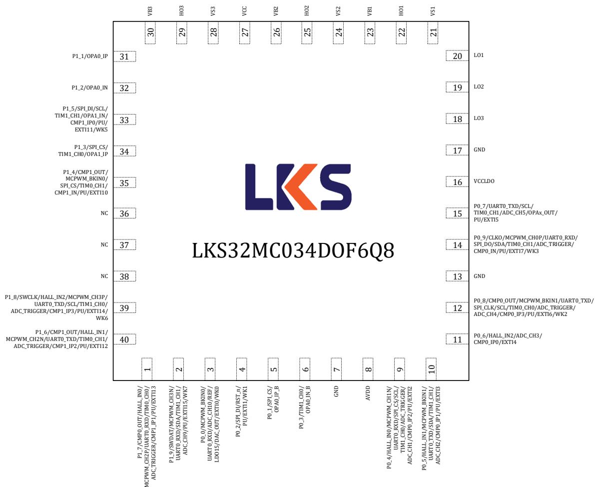
图 3-7 LKS32MC034DOF6Q8 管脚分布图
