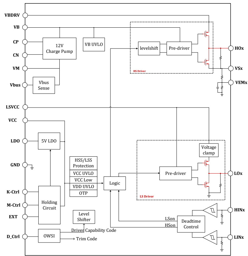
图 21-9 6N 型栅极驱动模块框图
