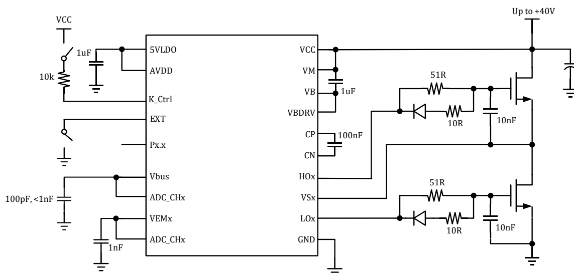
图 21-8 栅极驱动模块典型应用图
