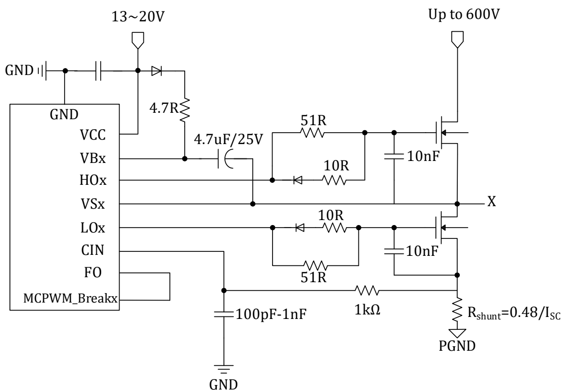
图 21-2 6N 型栅极驱动模块典型应用图
