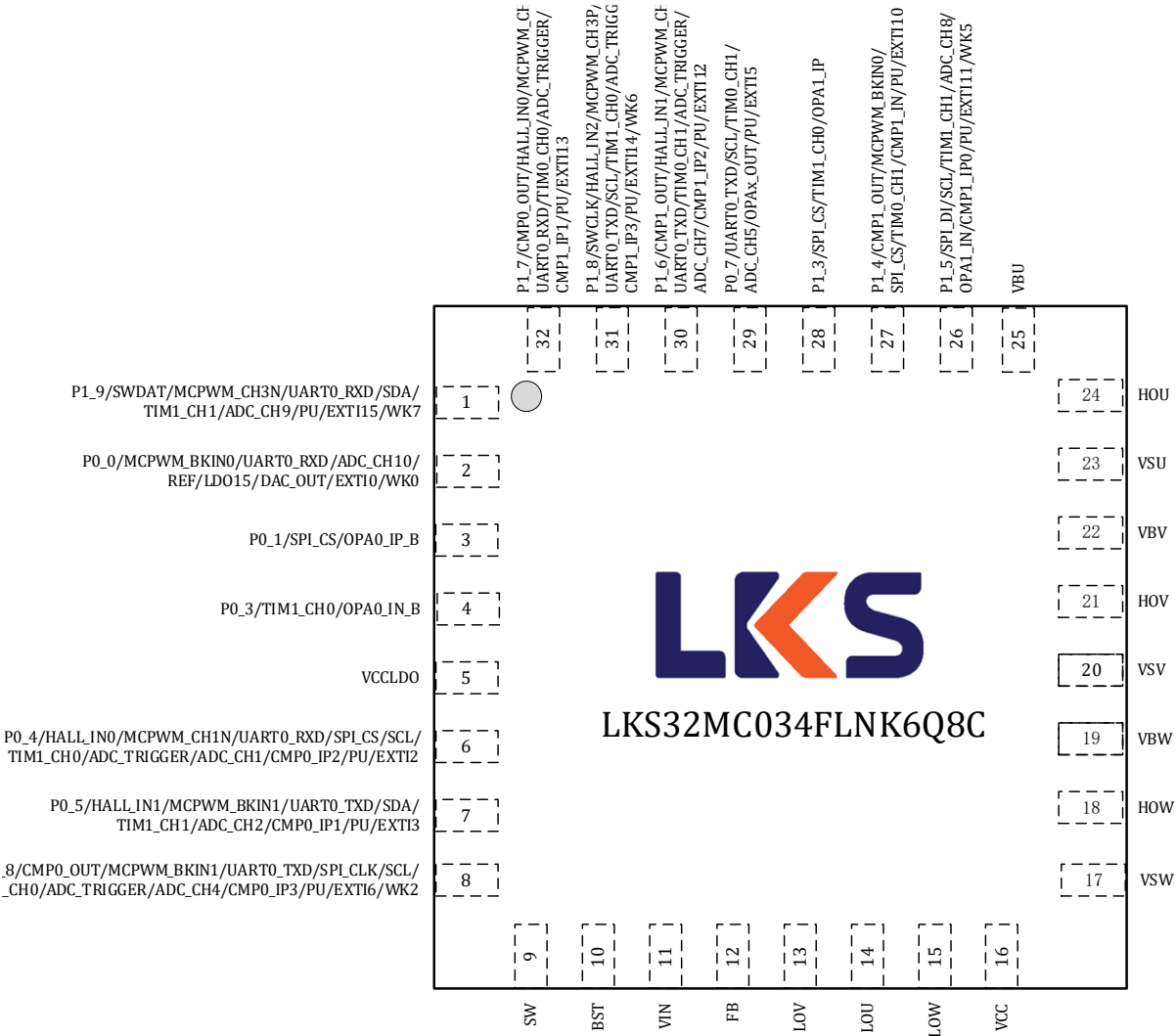
图 3-19 LKS32MC034FLNK6Q8C 管脚分布图
