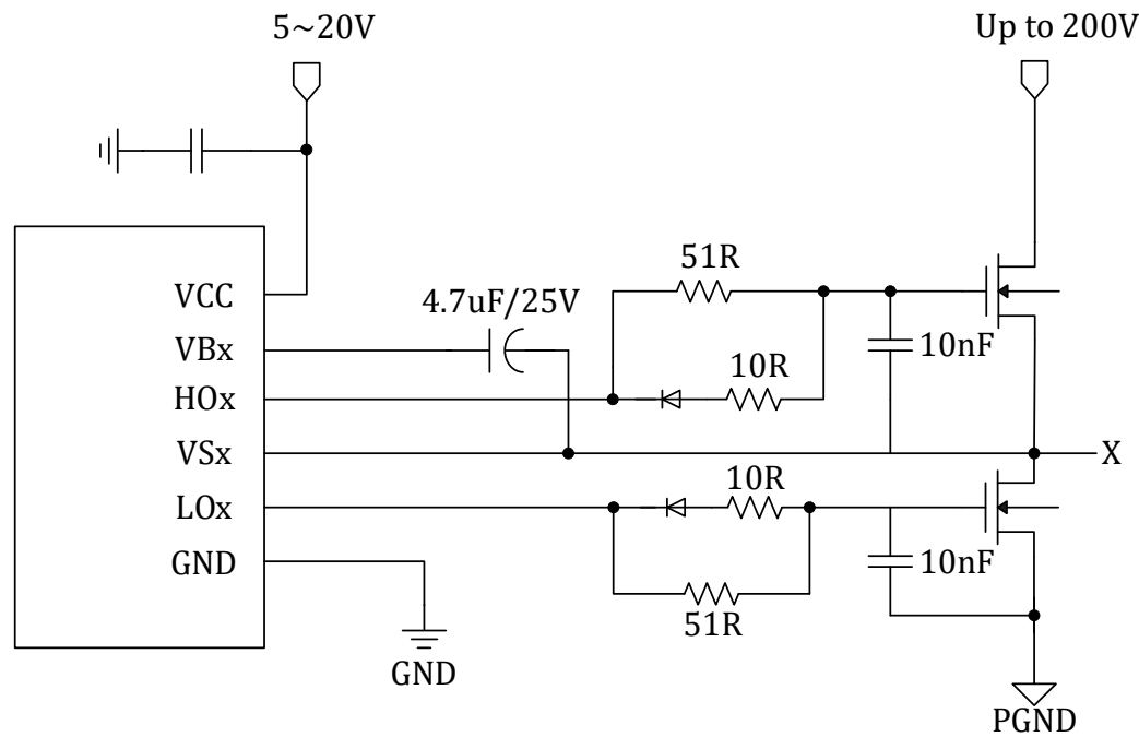
图 21-4 6N 型栅极驱动模块典型应用图
