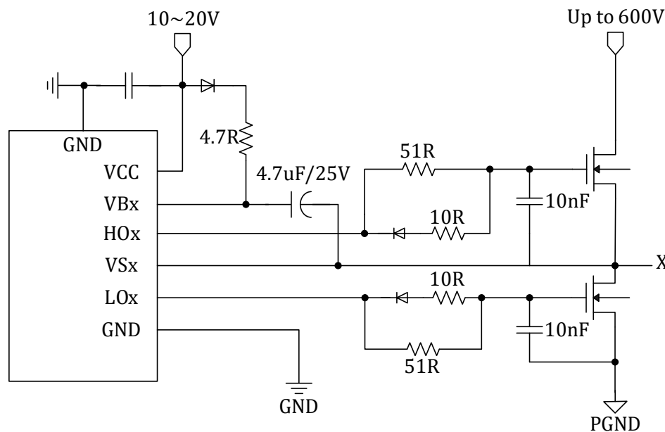
图 21-5 6N 型栅极驱动模块典型应用图
