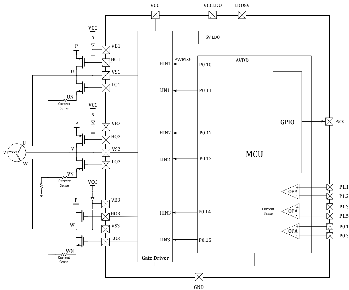
图 3-22 LKS32MC038KU6Q8B(C)预驱连接示意图
