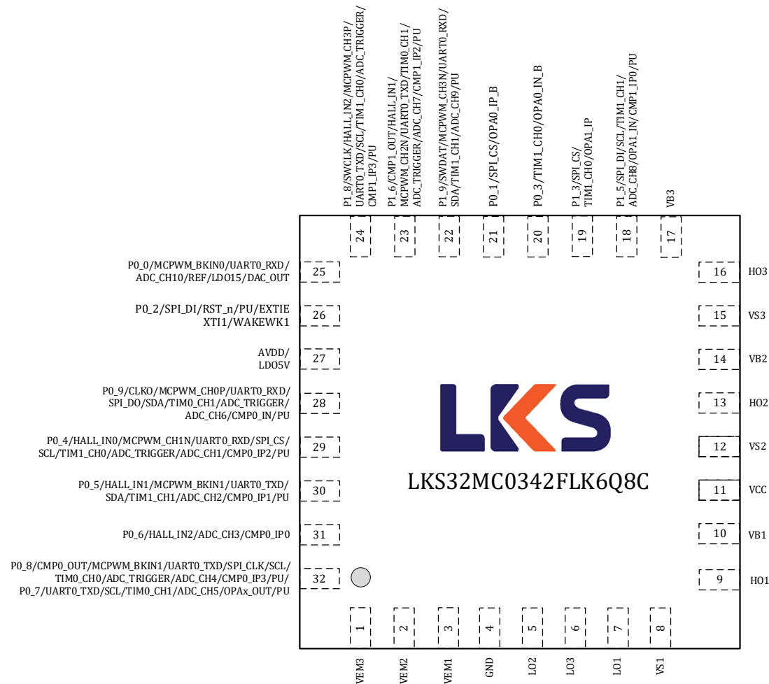
图 3-17 LKS32MC0342FLK6Q8C 管脚分布图
