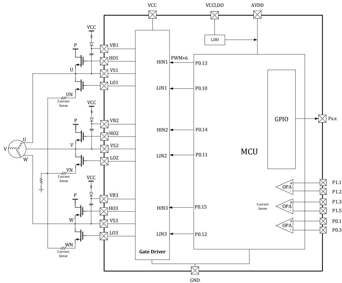
图 3-8 LKS32MC034DOF6Q8 预驱连接示意图
