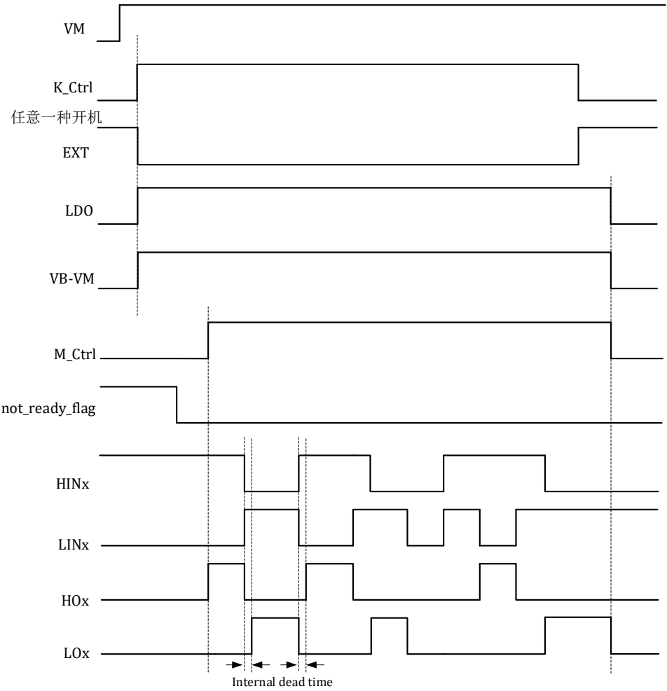
图 21-10 6N 型栅极驱动极性示意图
