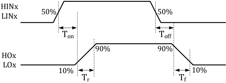
图 21-11 开关时序
