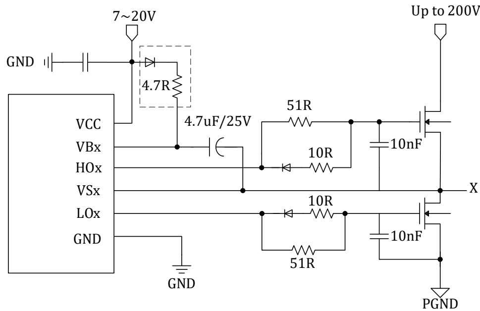
图 21-3 6N 型栅极驱动模块典型应用图
