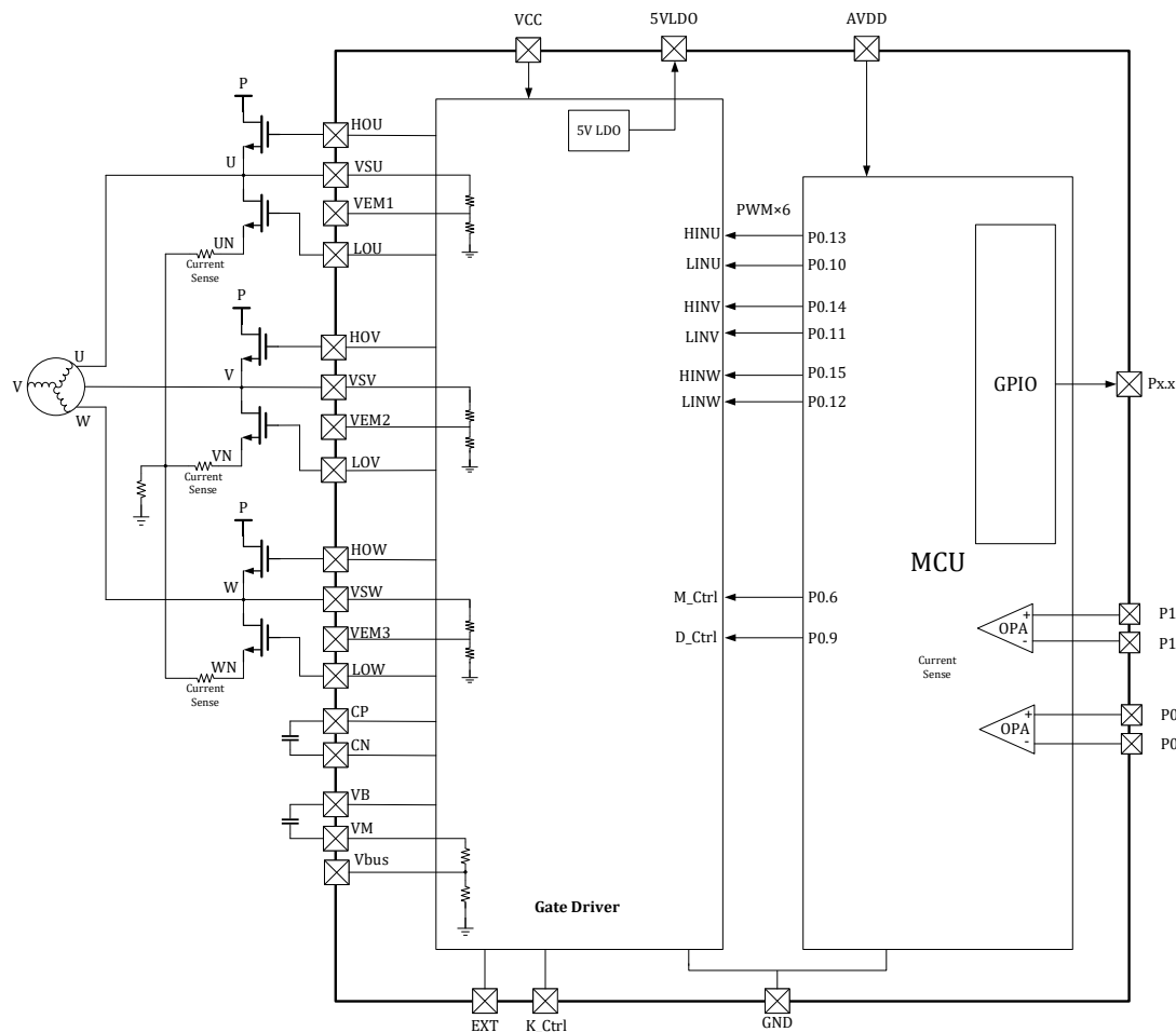
图 3-16 LKS32MC034F2LF6Q8C 预驱连接示意图
