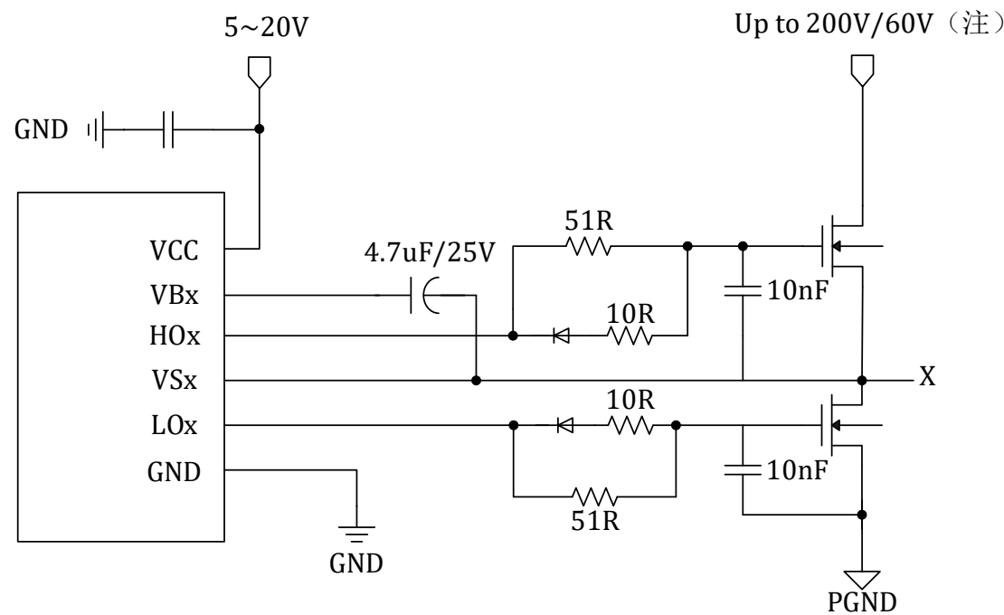
图 21-6 6N 型栅极驱动模块典型应用图
