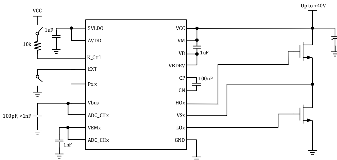
图 21-8 栅极驱动模块典型应用图
