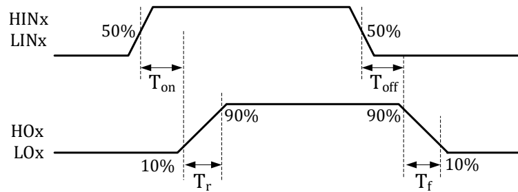
图 21-11 开关时序
