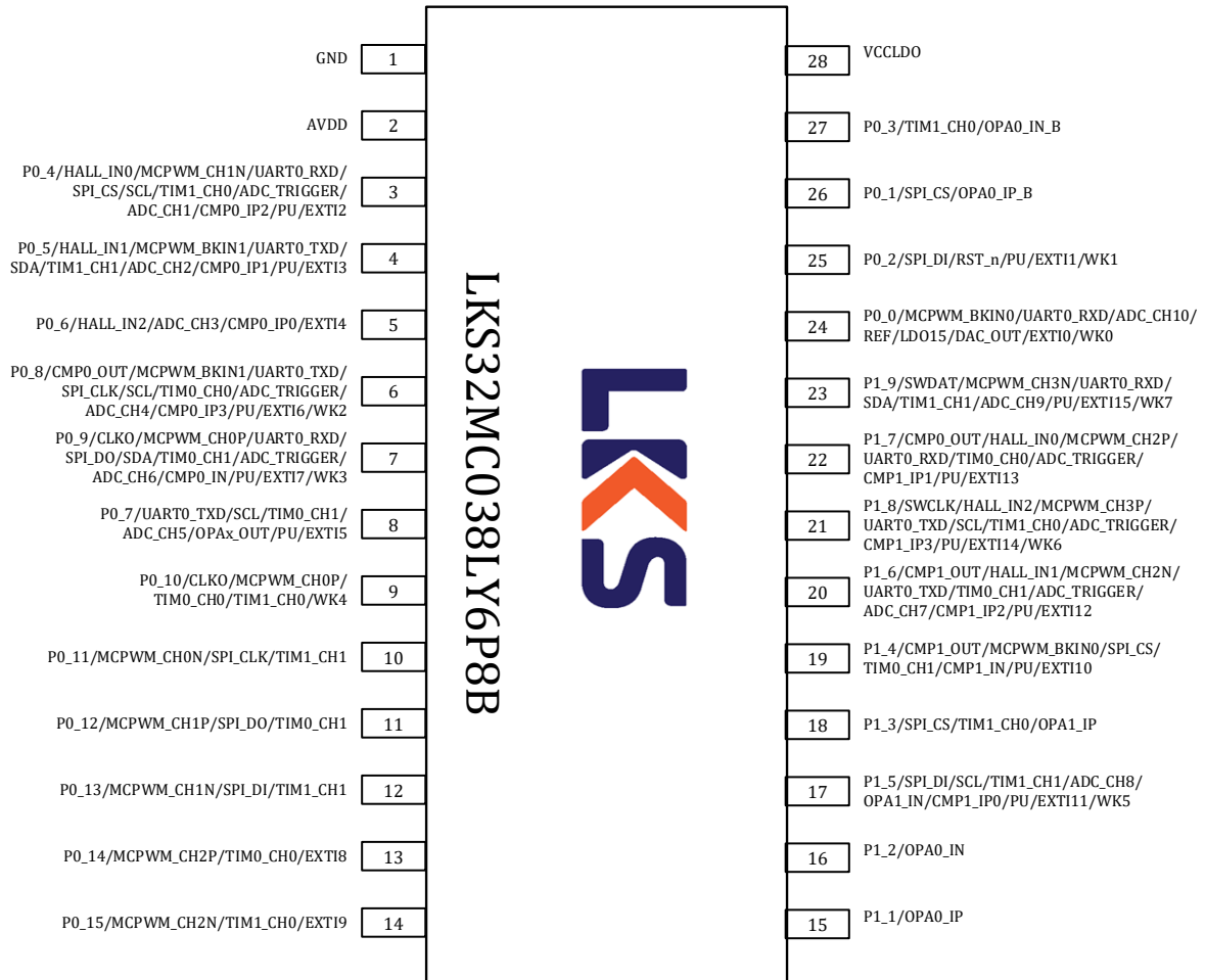
图 3-11 LKS32MC038LY6P8B/LKS32MC038LY6P8C 管脚分布图
