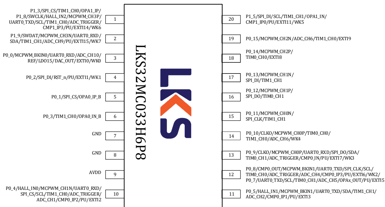
图 3-2 LKS32MC033H6P8 管脚分布图
