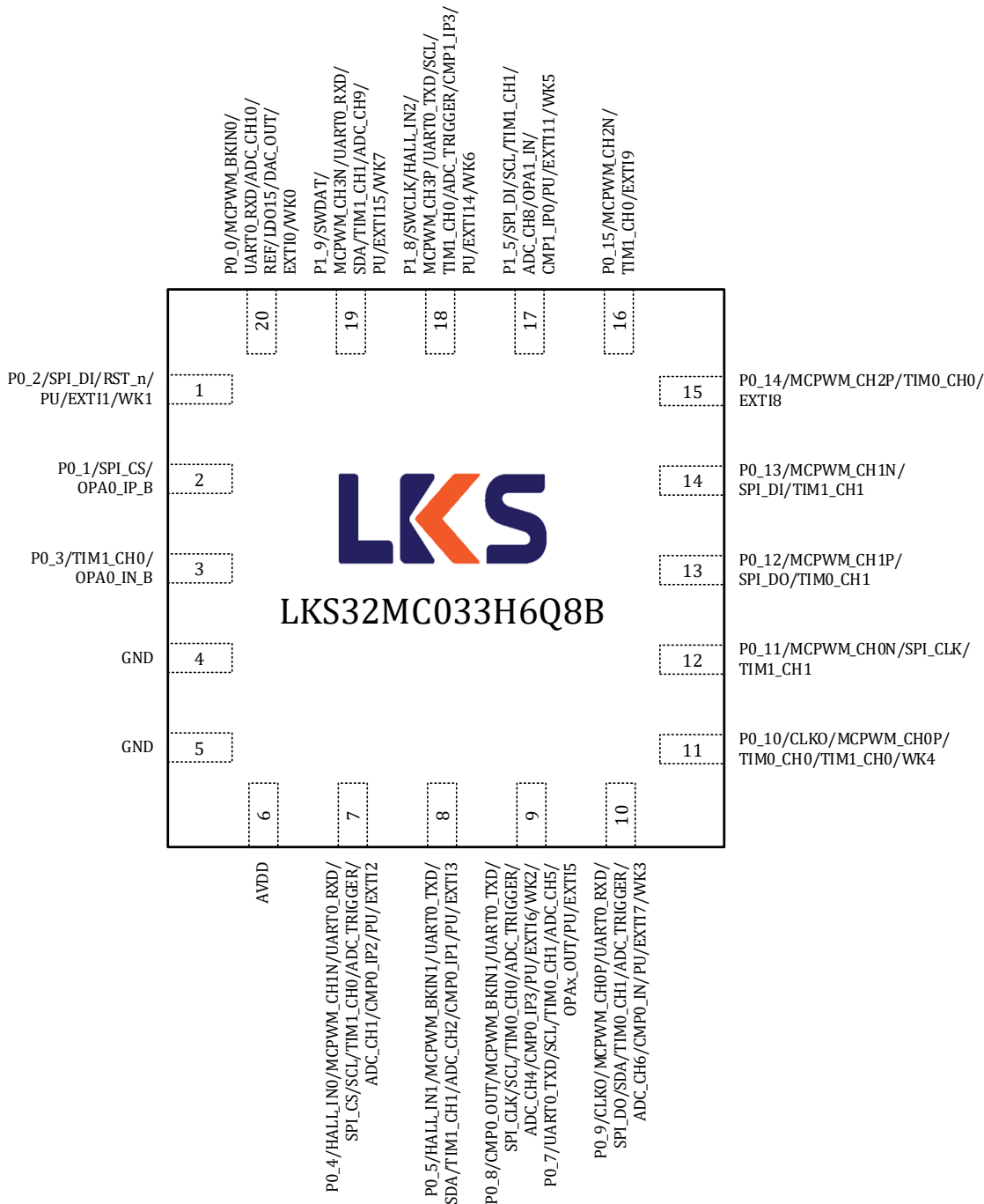
图 3-5 LKS32MC033H6Q8B 管脚分布图
