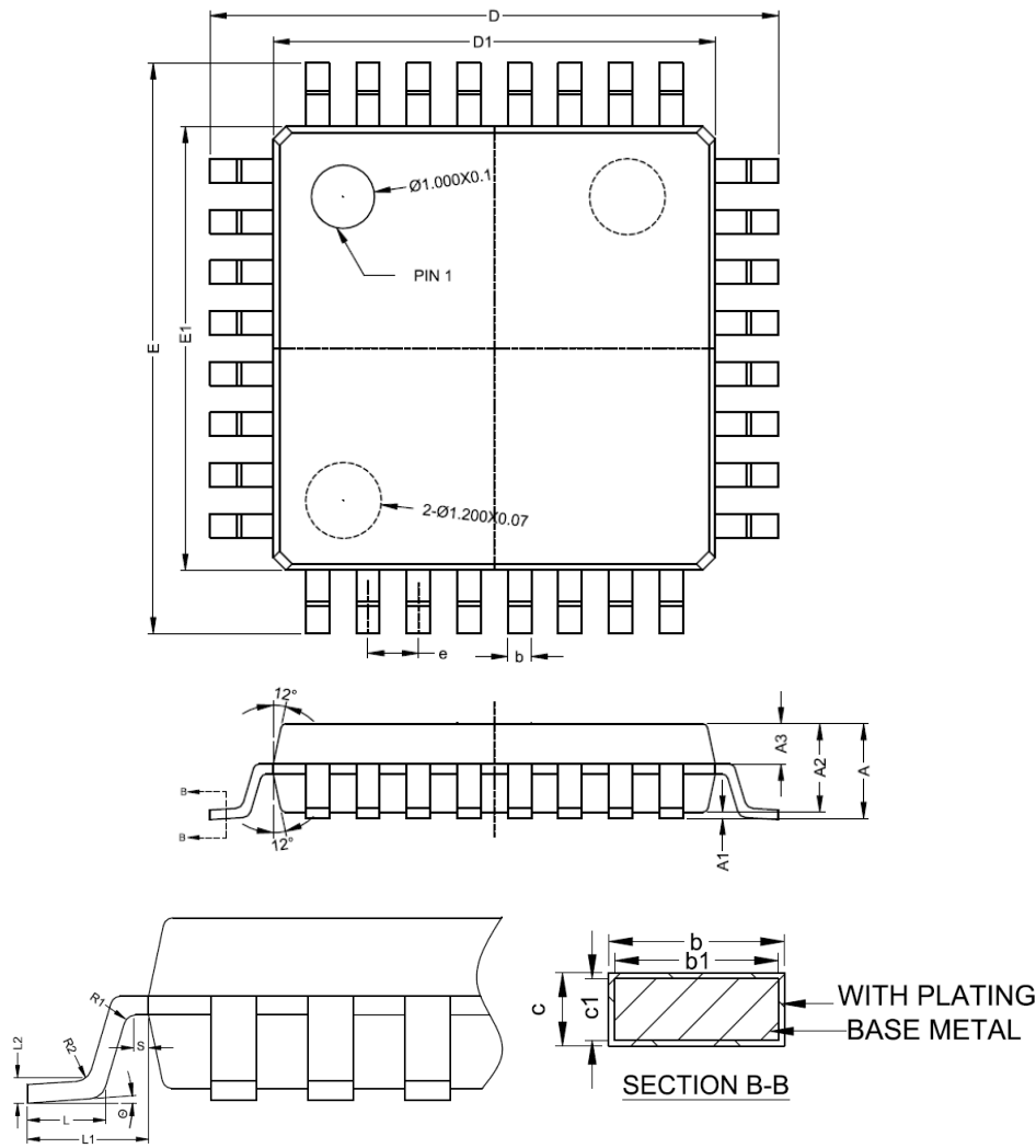
图 4-6 LKS32MC032LK6T8C 封装图示
