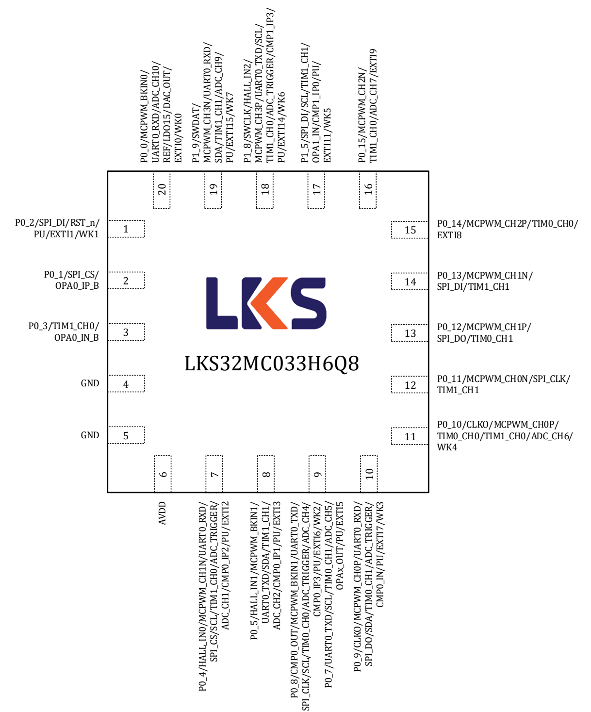
图 3-4 LKS32MC033H6Q8 管脚分布图
