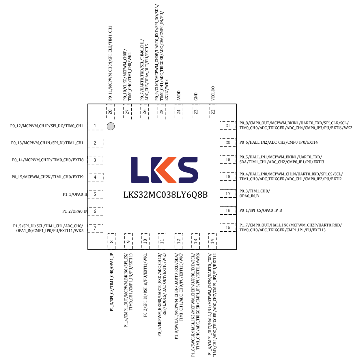
图 3-12 LKS32MC038LY6Q8B/LKS32MC038LY6Q8C 管脚分布图
