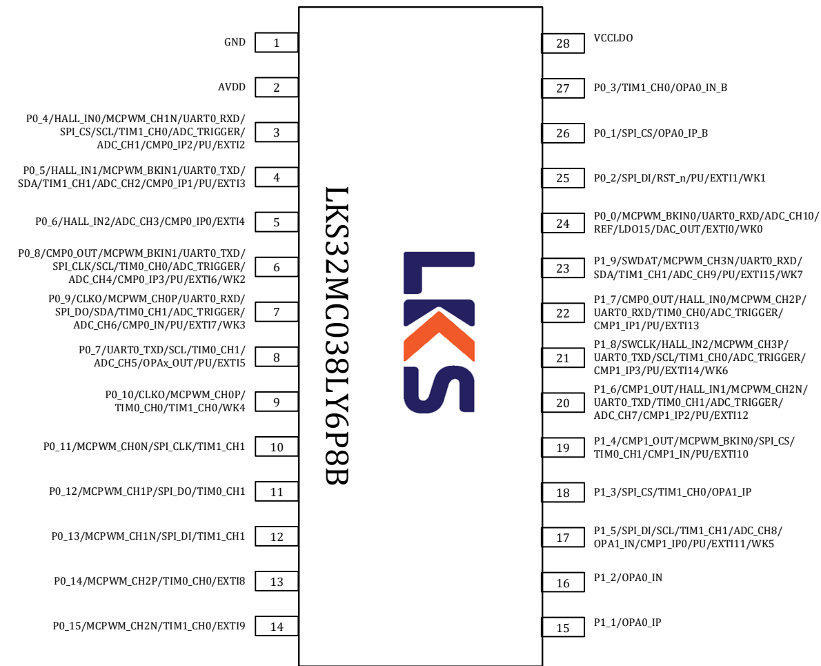
图 3-11 LKS32MC038LY6P8B/LKS32MC038LY6P8C 管脚分布图
