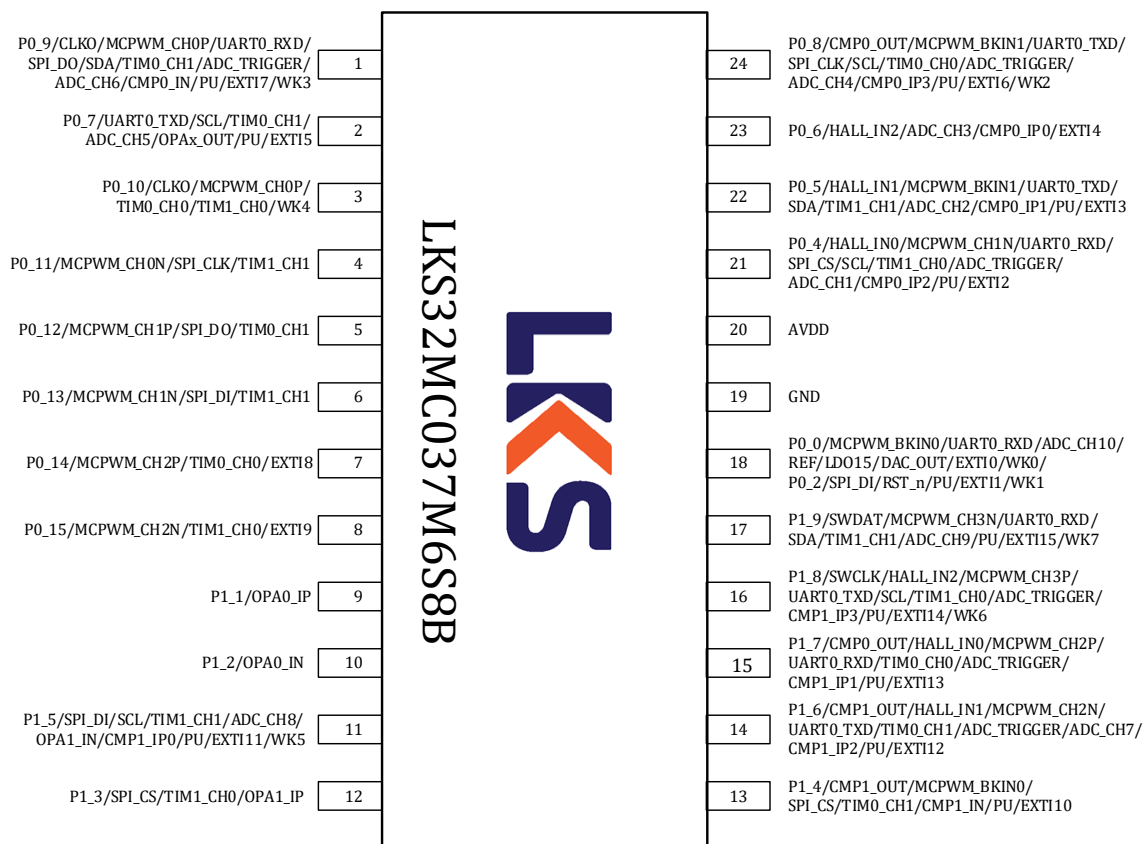
图 3-7 LKS32MC037M6S8B/LKS32MC037M6S8C 管脚分布图
