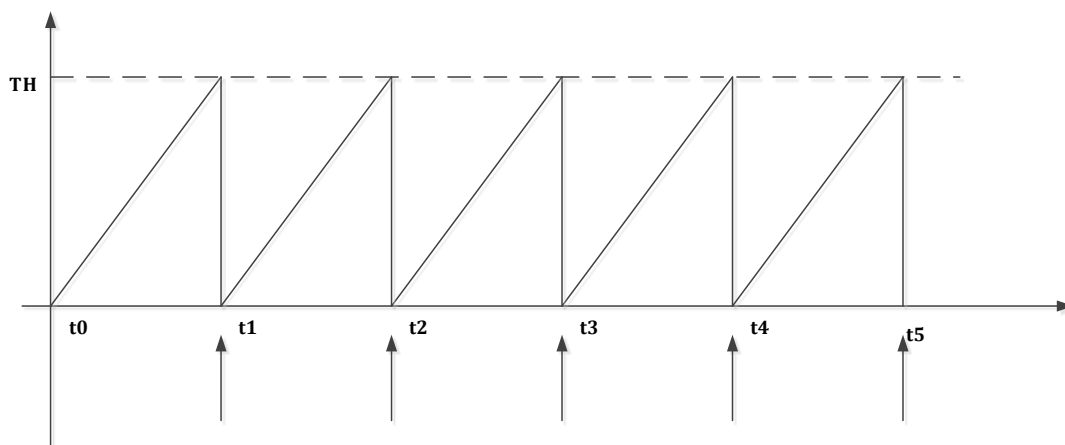
Fig. 13-3 UTimer
