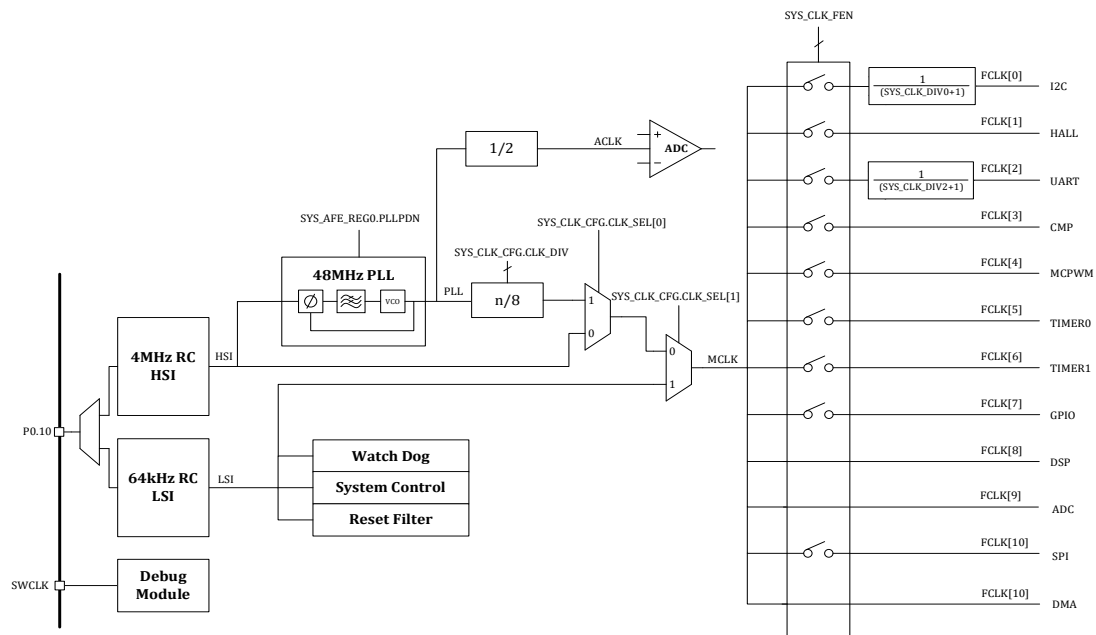
图 6-1 时钟架构
