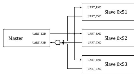
图 16-4 UART 多机通讯示例
