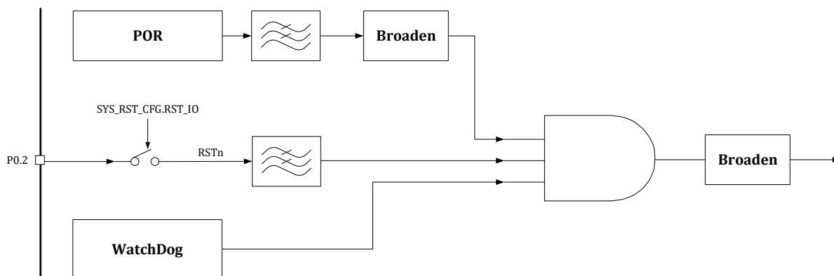
图 6-2 复位架构
