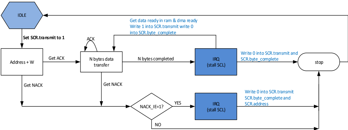
图 9-11 主模式下多字节发送示意图
