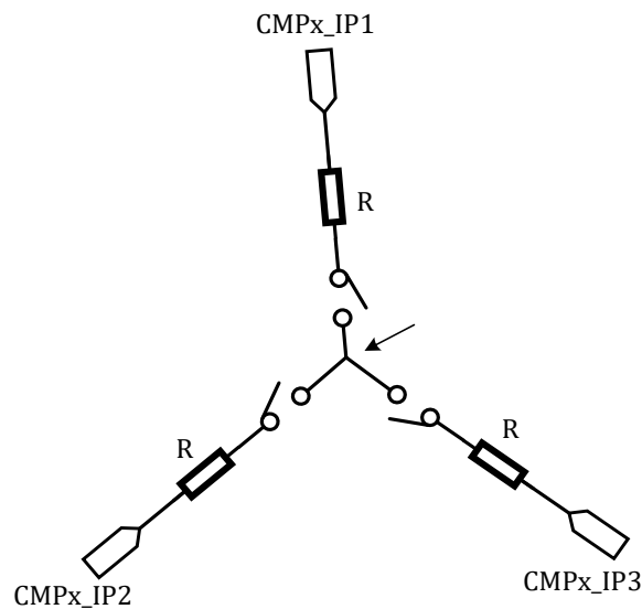
图 5-5 BEMFx_MID 信号
