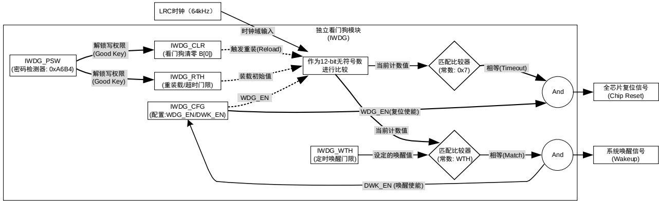
图 19-2 IWDG 工作原理和信号流向
