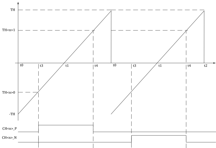
图 14-9 MCPWM 时序 TH_{<n>0} 和 TH_{<n>1} -中心对齐推挽模式
