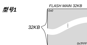
图 7-1 非易失性存储体空间划分框图及型号
