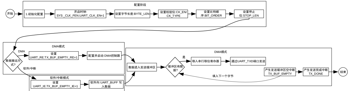
图 16-1 UART 发送流程和硬件机制
