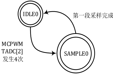
图 12-6 ADC 单段采样状态转移图
