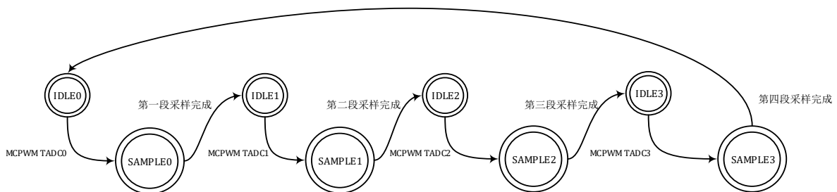
图 12-8 ADC 四段采样状态转移图
