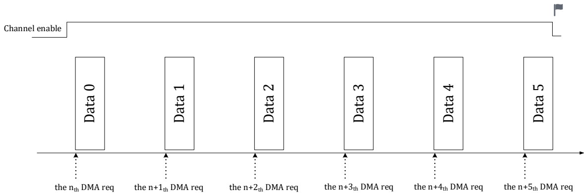
图 17-3 RMODE=1 DMA 传输情况
