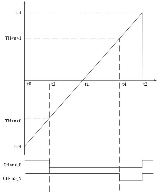
图 14-10MCPWM 时序边沿对齐模式
