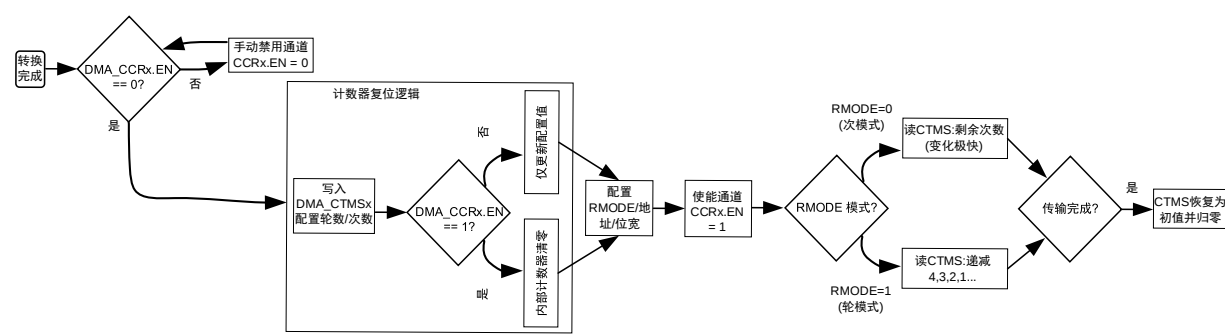
图 17-7 DMA 操作逻辑流程图
