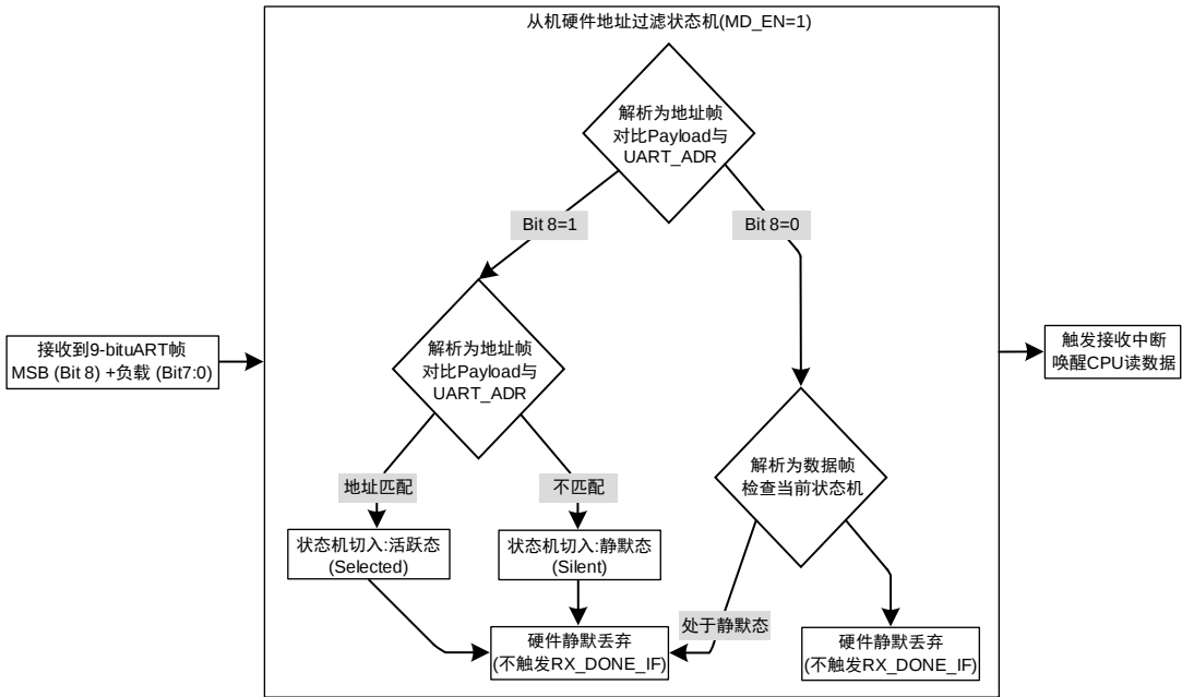
图 16-4 从机 9-bit UART 地址帧过滤状态机处理流程
