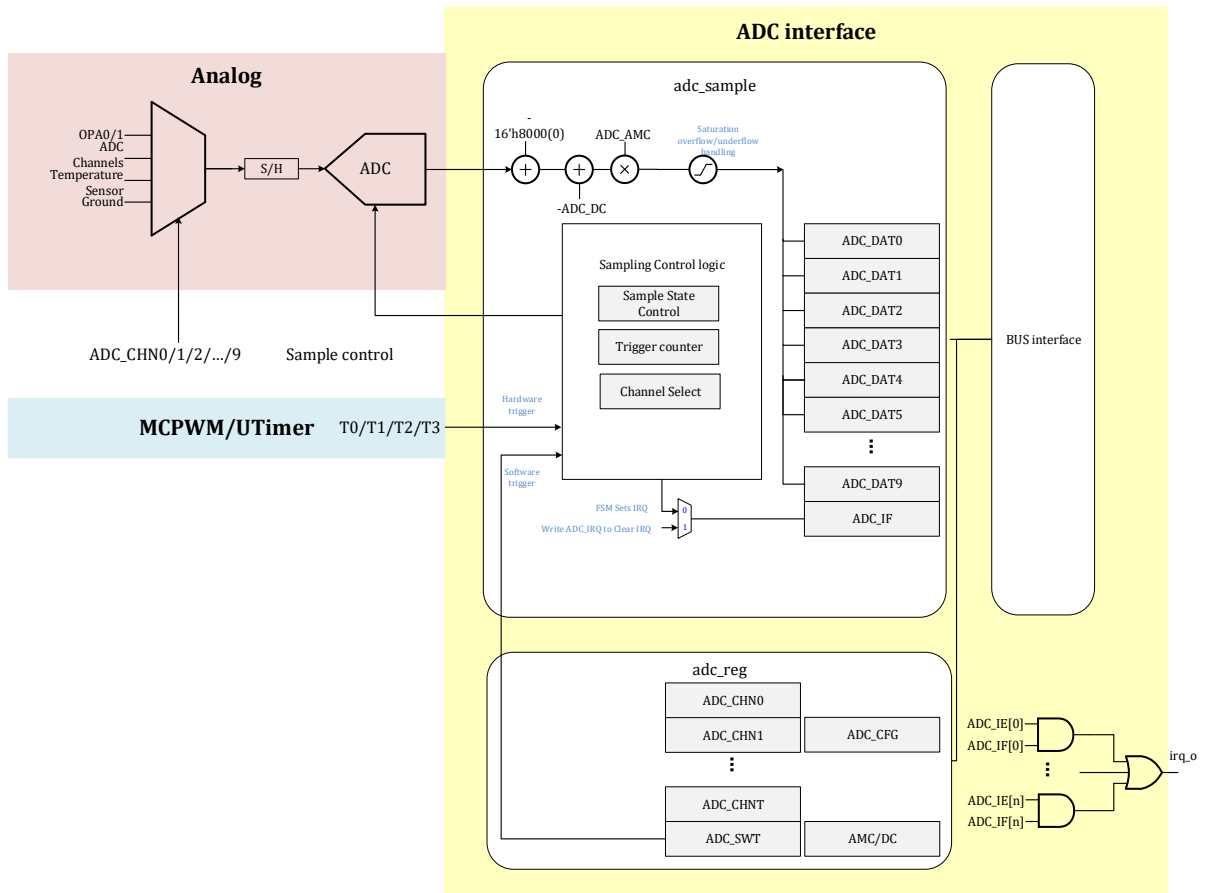
图 12-1 ADC 采集模块功能框图
