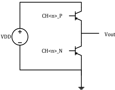
图 14-12MCPWM IO 控制示意图
