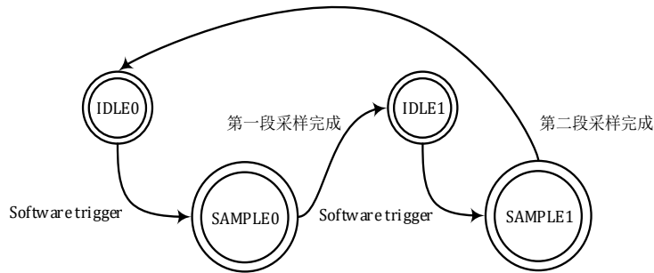
图 12-7 ADC 两段采样状态转移图
