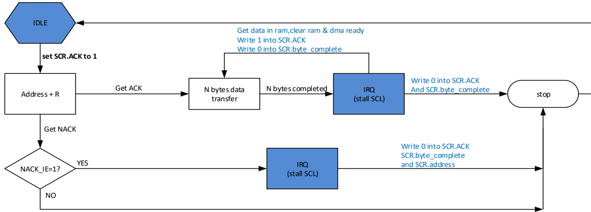
图 9-12 主模式下多字节接收示意图
