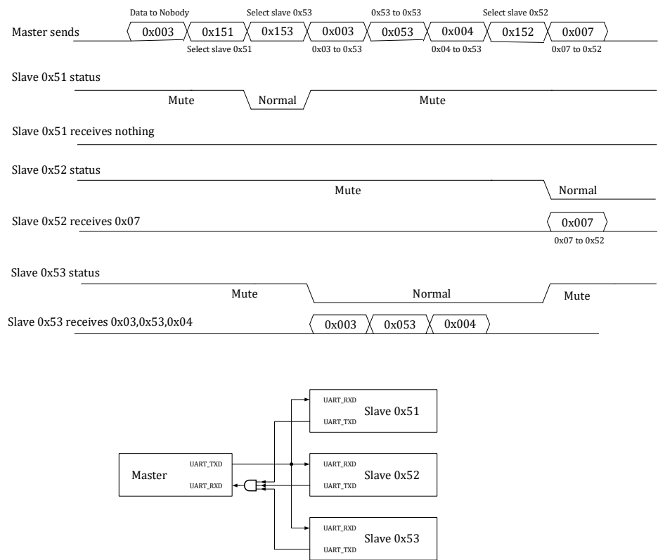
图 16-5 UART 多机通讯示例
