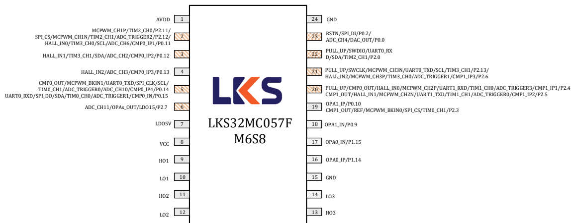
图 3-2 LKS32MC057FM6S8 管脚分布图
