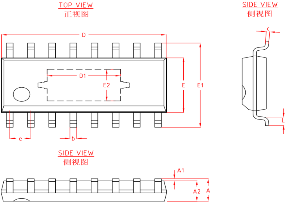
图 4-3 LKS32MC055EL6S8 封装图示
