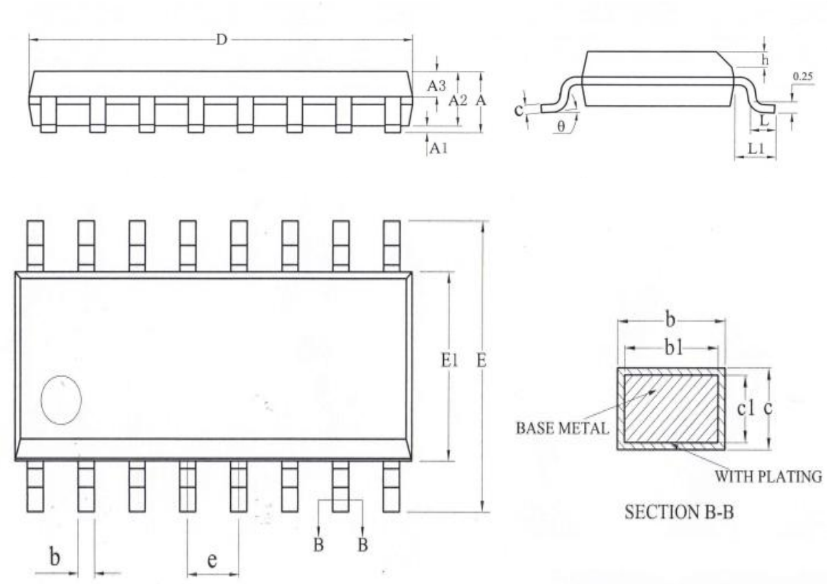
图 4-2 LKS32MC055DL6S8 封装图示
