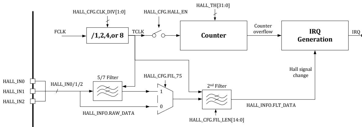
图 11-2 数据流程框图
