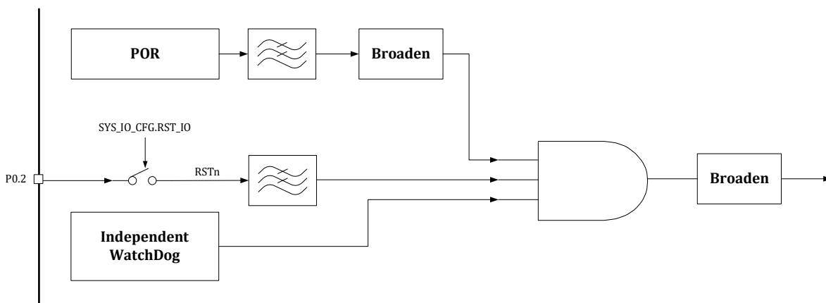
图 6-2 复位架构
