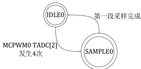
图 12-10 ADC 单段采样状态转移图
