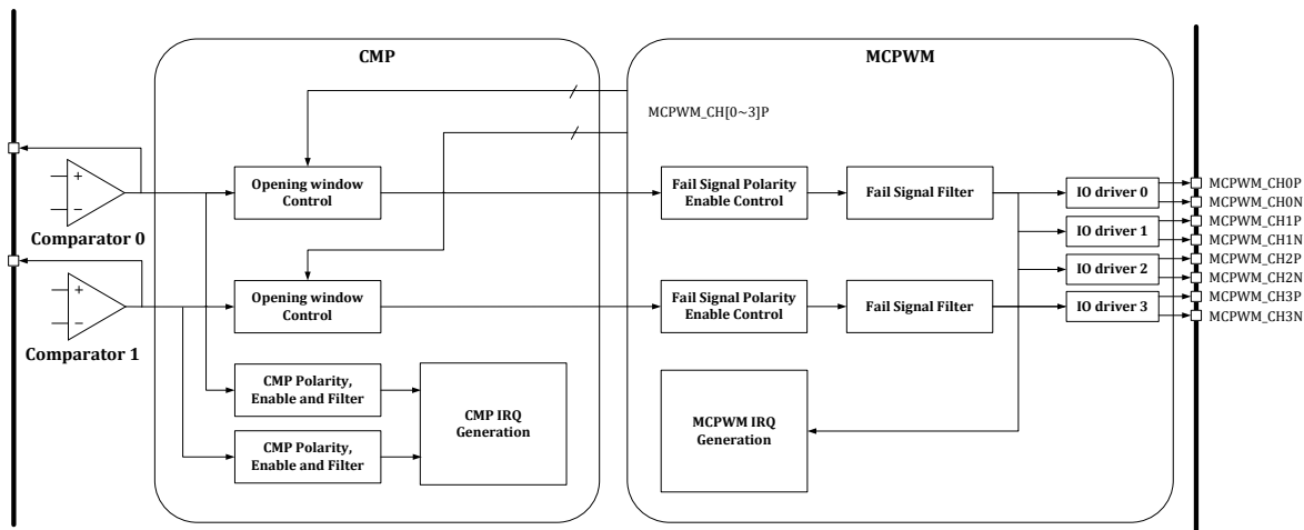
图 10-3 CMP 与 MCPWM 的联动
