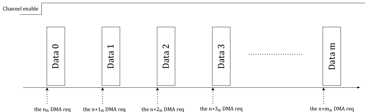
图 18-5 CIRC=1 且 RMODE=1 DMA 传输情况
