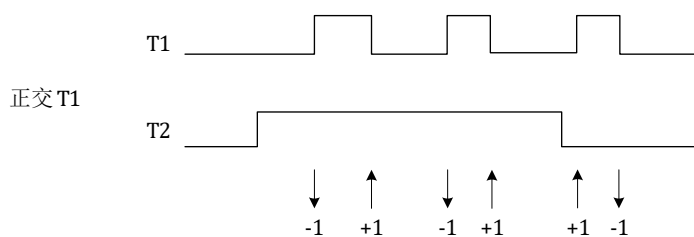
图 13-14 编码器在 T1 或 T2 时刻计数的正交编码信号计数情况
