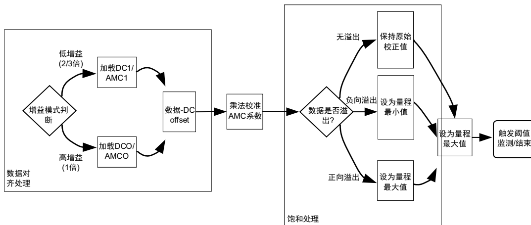
图 12-9 ADC 自动校准逻辑流程图
