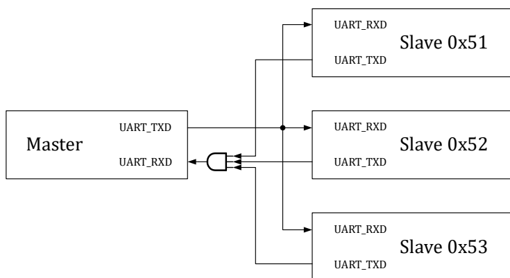
图 17-3 UART 多机通讯互联拓扑
