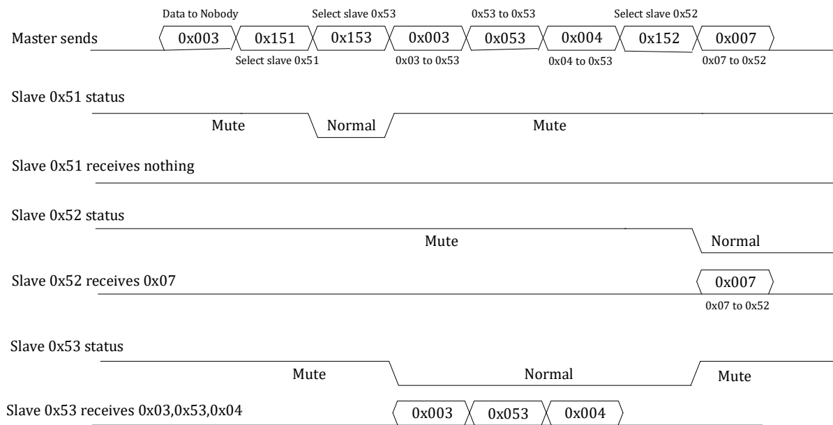
图 17-4 UART 多机通讯示例
