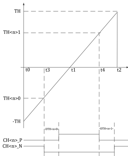
图 14-8MCPWM 时序 TH<n>0 和 TH<n>1-中心对齐模式
