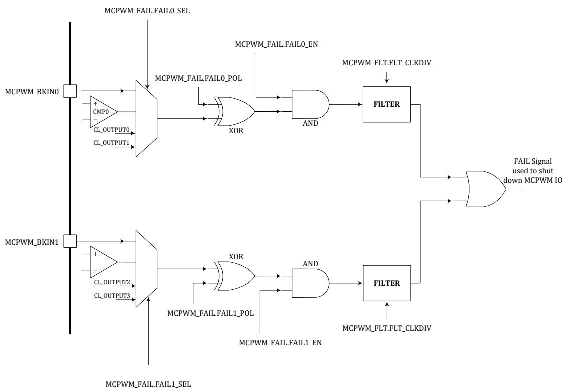
图 14-5 MCPWM FAIL 逻辑示意图
