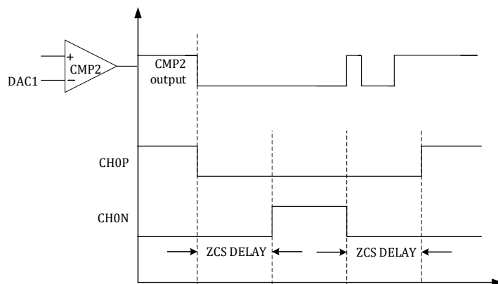
图 14-15 比较器 2 触发 ZCS 事件发生时 MCPWM 通道 0 动作时序
