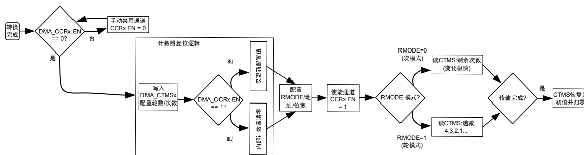
图 18-8 DMA 操作逻辑流程图
