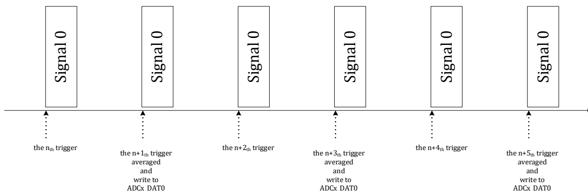
图 12-7 过采样转换时序示例 2
