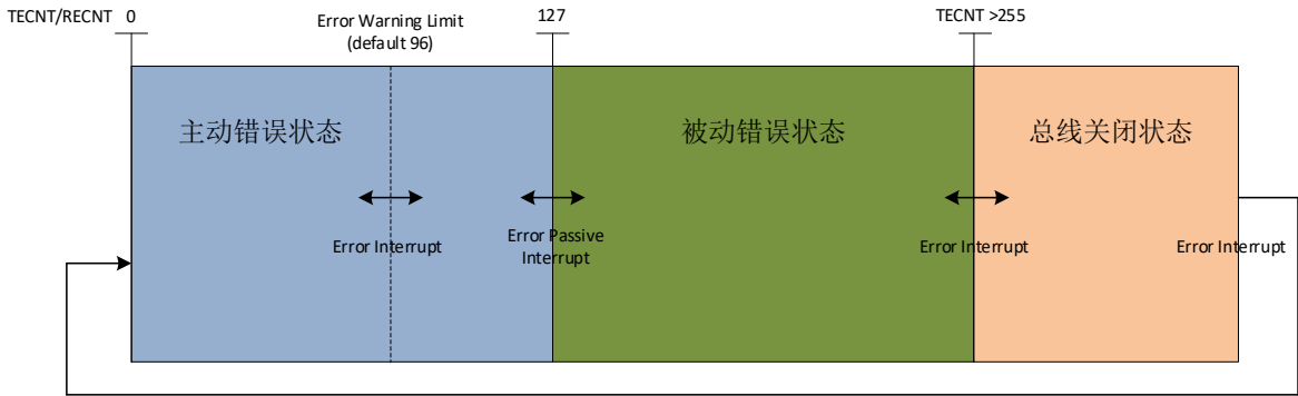
图 24-5 CAN 模块错误管理
