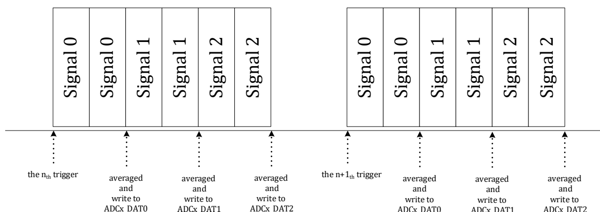
图 12-6 过采样转换时序示例 1
