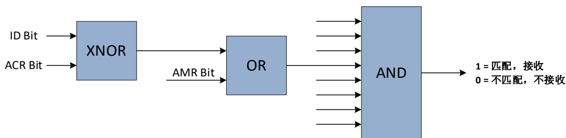
图 24-4 CAN 模块 ID 滤波逻辑关系
