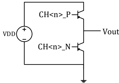
图 14-12MCPWM IO 控制示意图
