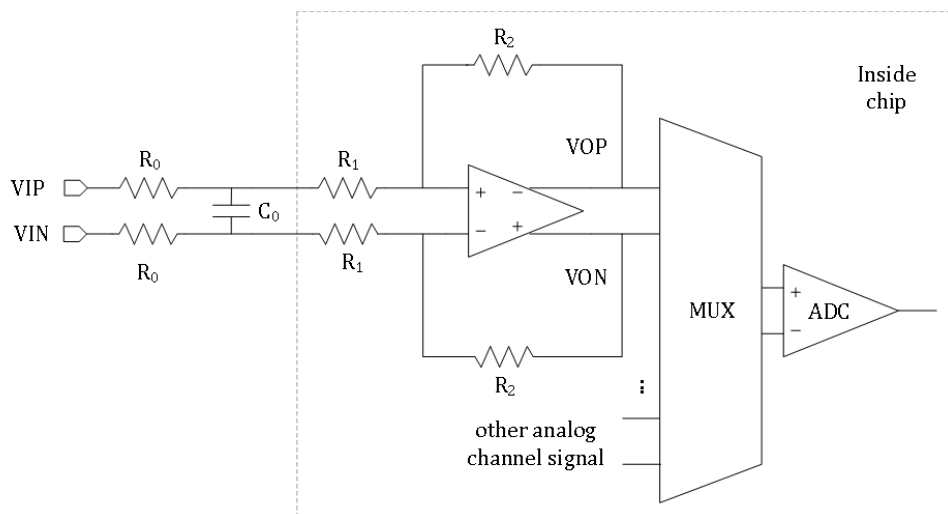
图 5-2 放大器框图
