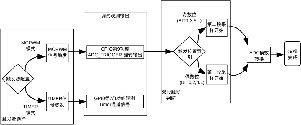
图 12-8 ADC 触发与调试观测流程图
