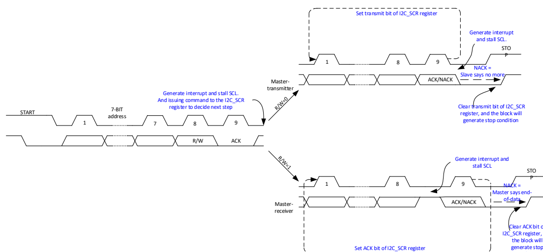
图 9-9 主模式下单字节传输示意图
