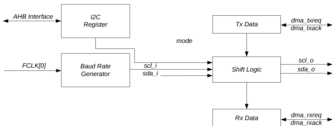
图 9-1I2C 模块顶层功能框图
