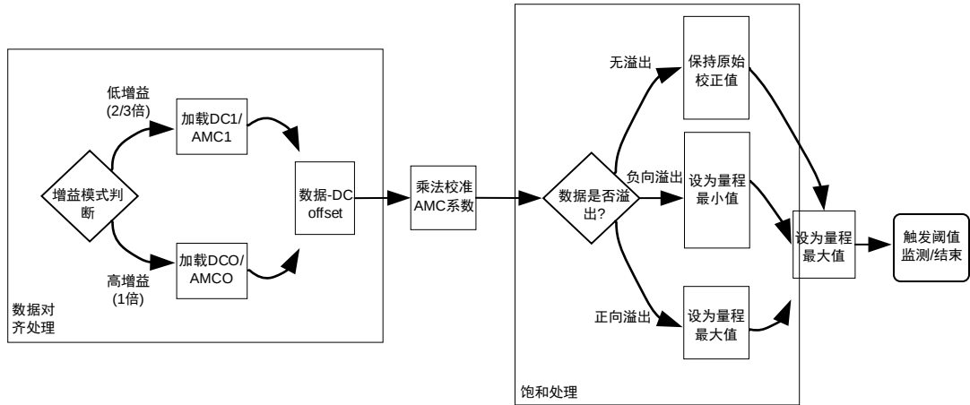
图 12-9 ADC 自动校准逻辑流程图
