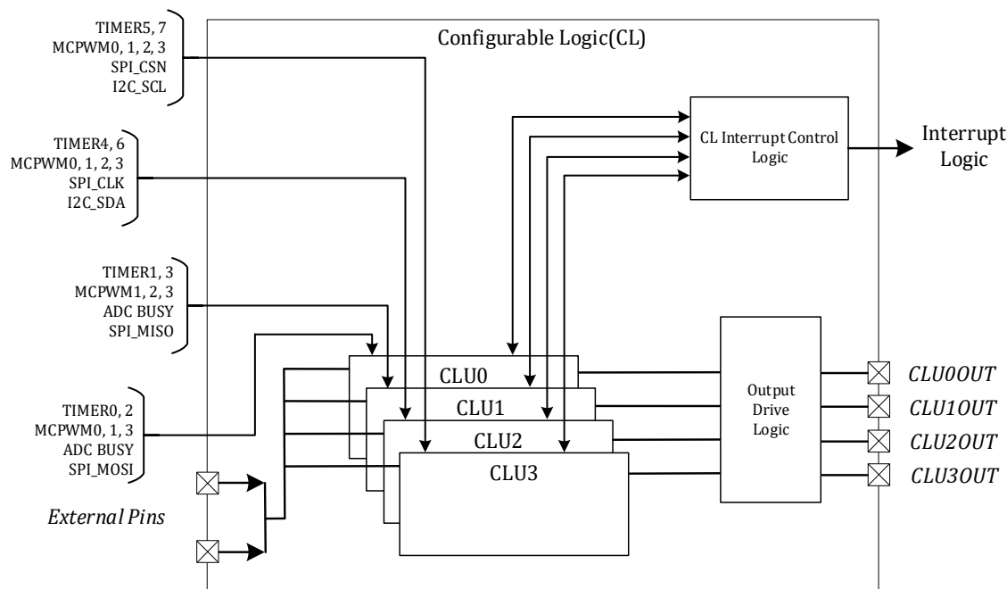
图 23-1 CL 模块顶层功能框图
