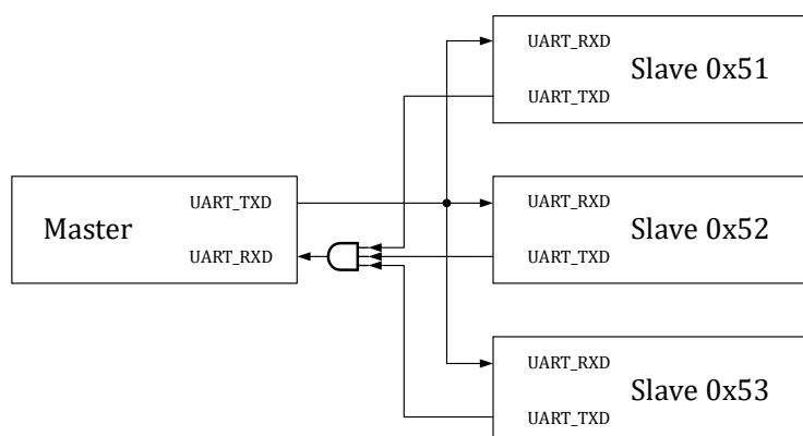
图 17-3 UART 多机通讯互联拓扑
