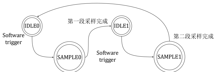
图 12-11 ADC 两段采样状态转移图
