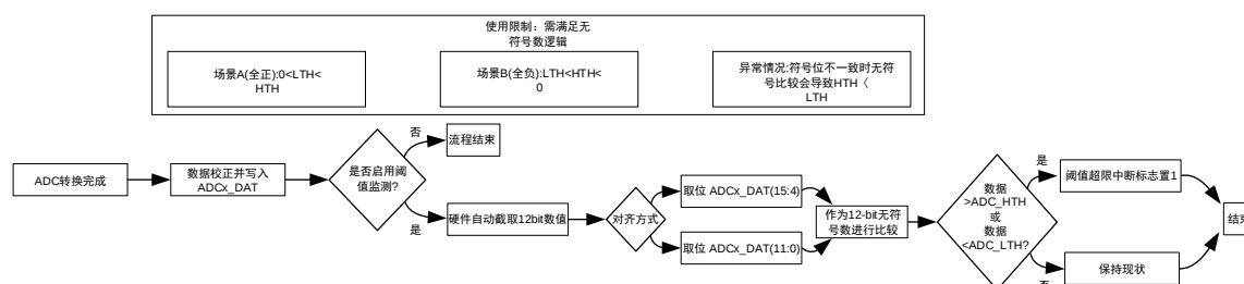
图 12-5 ADC 校正处理流程图
