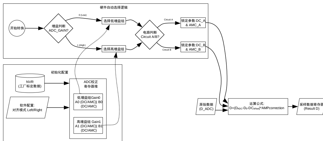
图 12-4 ADC 校正处理流程图
