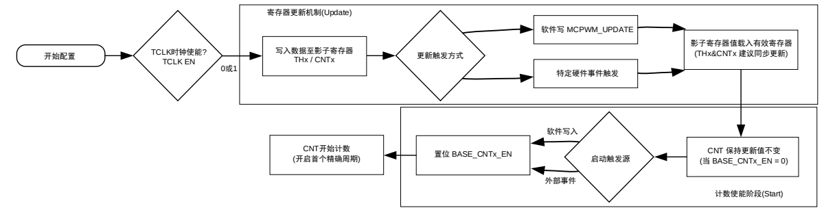
图 14-4 时基寄存器更新与计数使能流程图
