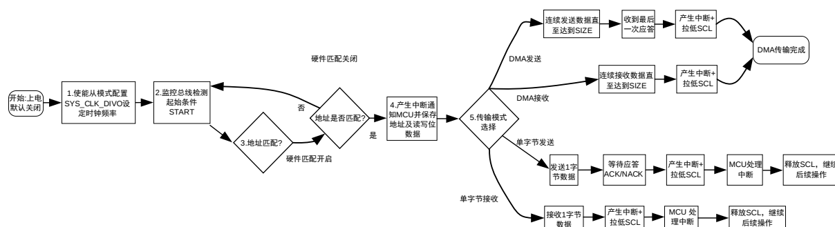
图 9-4 I2C 从模式工作流程图
