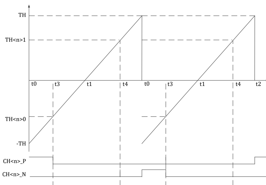
图 14-11 MCPWM 时序 TH&lt;n&gt;0 和 TH&lt;n&gt;1 边沿对齐推挽模式
