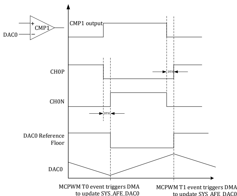
图 14-14 MCPWM 通道 0 受比较器 1 控制进行状态动作时序图
