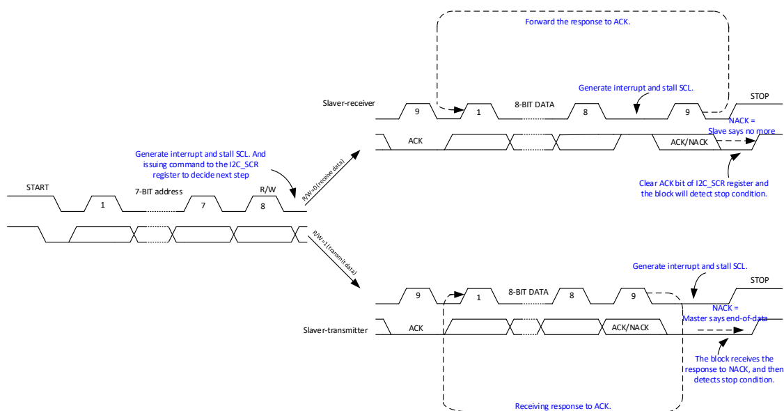
图 9-5 从模式传输示意图
