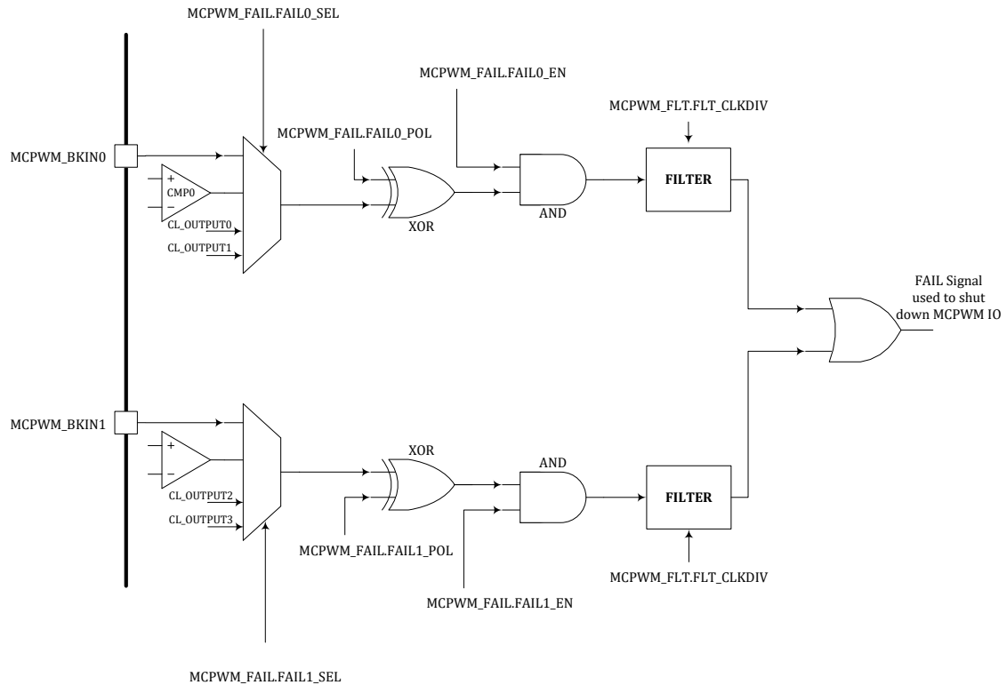
图 14-5 MCPWM FAIL 逻辑示意图
