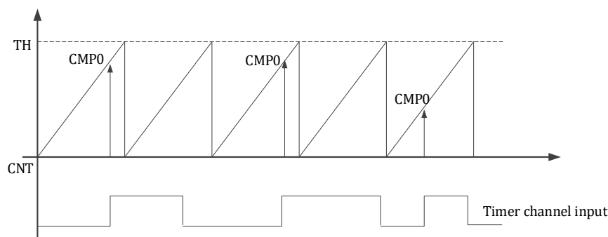
图 13-4 TIMER 捕获模式
