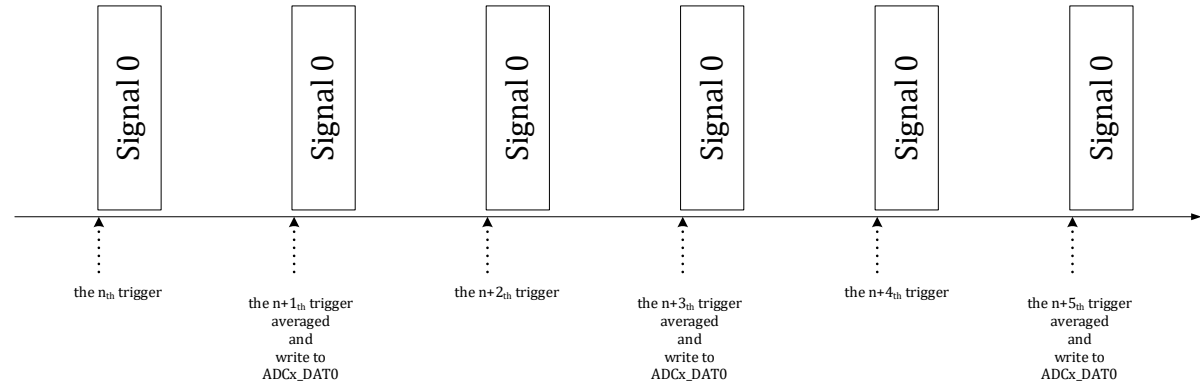
图 12-7 过采样转换时序示例 2
