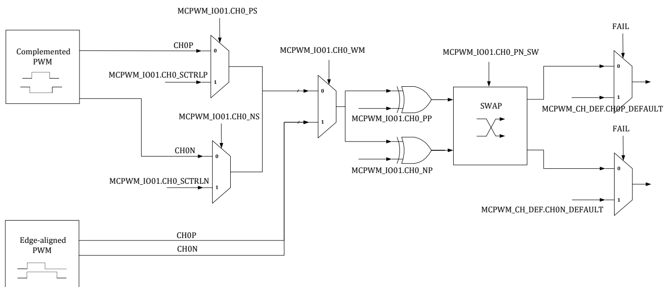
图 14-7 IO Driver 模块数据流程图
