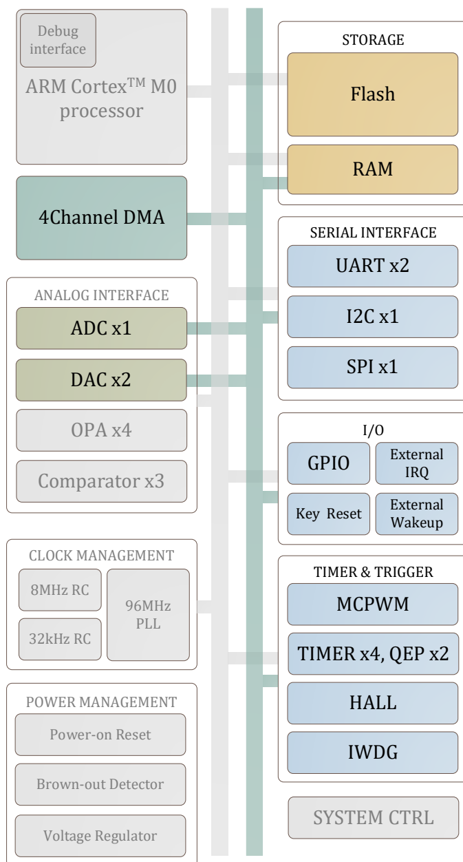
图 18-1 multi-layer AHB 总线架构
