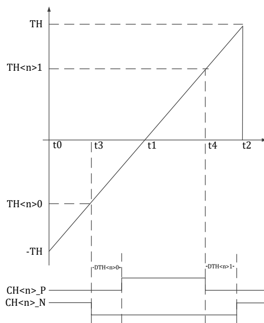
图 14-8 MCPWM 时序 TH&lt;n&gt;0 和 TH&lt;n&gt;1-中心对齐模式
