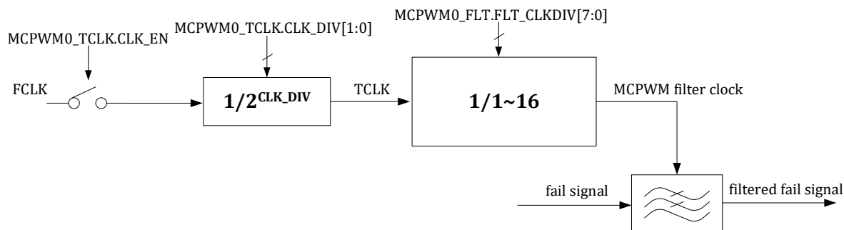
图 14-6 MCPWM Fail 信号滤波时钟生成逻辑
