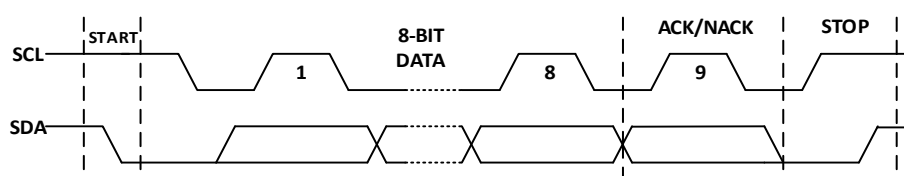
图 9-2 基本 I2C 传输时序图
