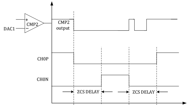
图 14-15 比较器 2 触发 ZCS 事件发生时 MCPWM 通道 0 动作时序
