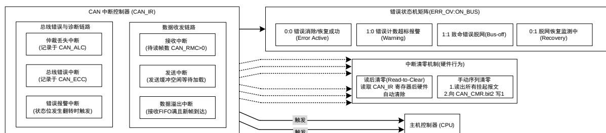
图 24-2 CAN 模块中断处理与状态机架构
