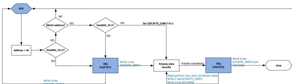
图 9-8 从模式下多字节接收示意图
