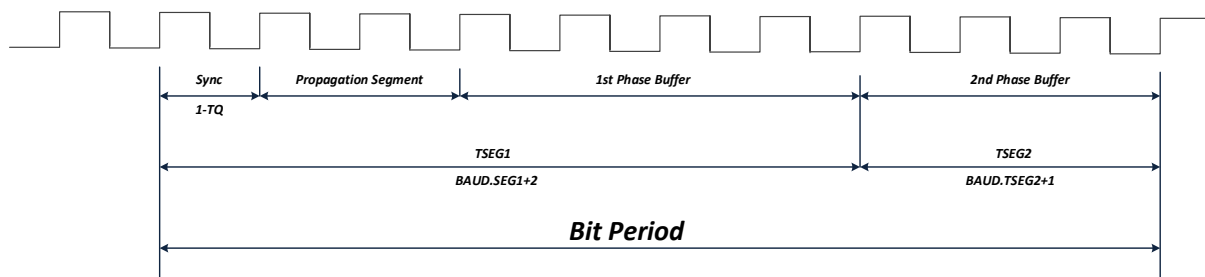
图 24-3 CAN 模块 Bit 周期介绍图
