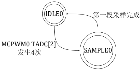
图 12-10 ADC 单段采样状态转移图
