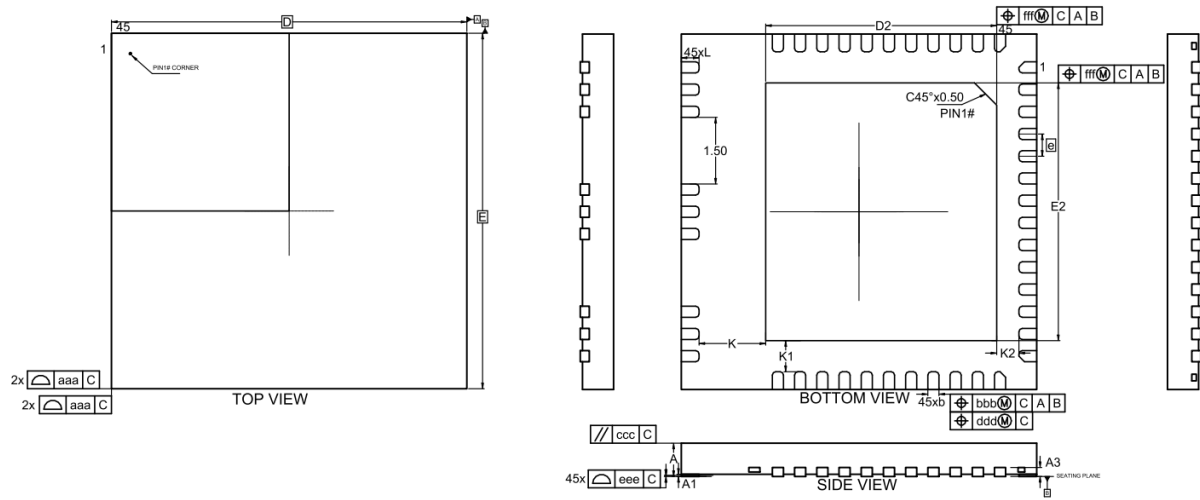
图 4-5 LKS32MC078KUBQ8 封装图示
