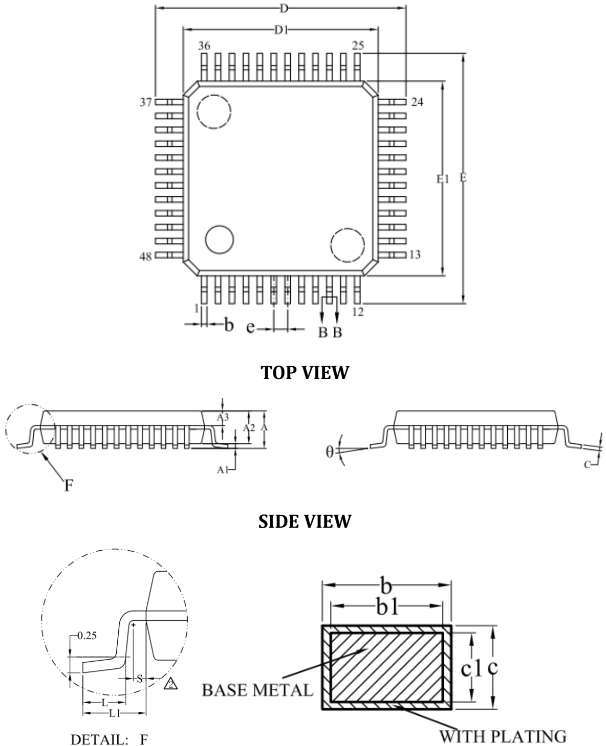
图 4-2 LKS32MC071DOC8T8 封装图示
