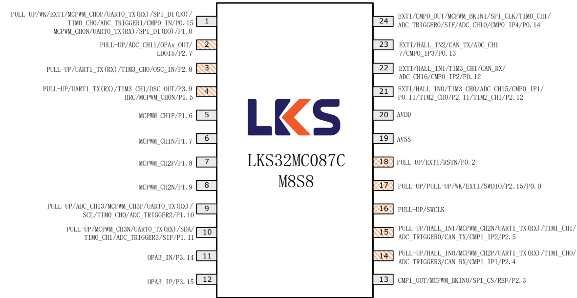
图 3-7 LKS32MC087CM8S8(B)管脚分布图
