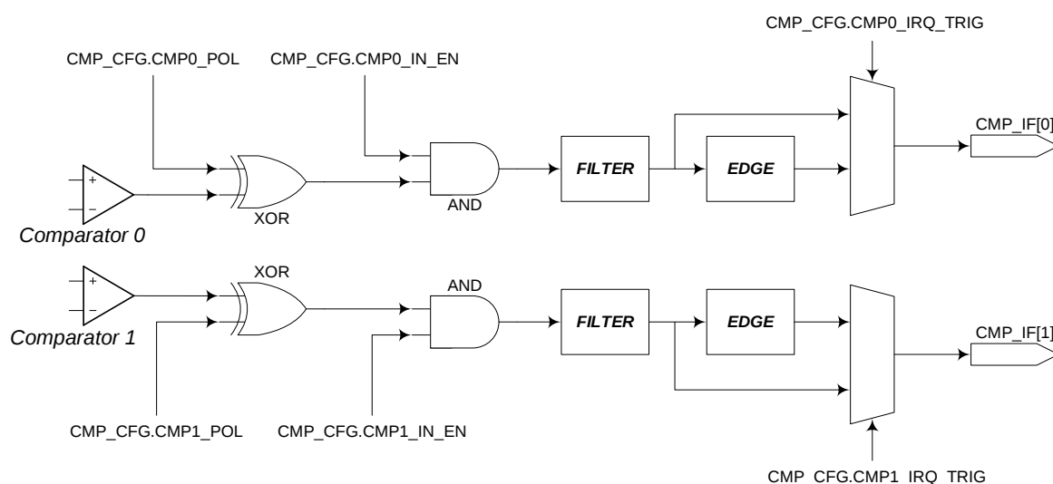
图 18-3 比较器控制及中断产生逻辑
