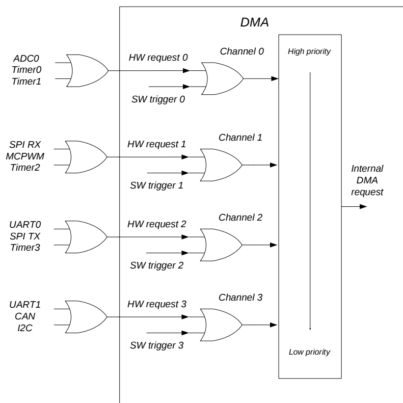
图 7-4 DMA 通道优先级
