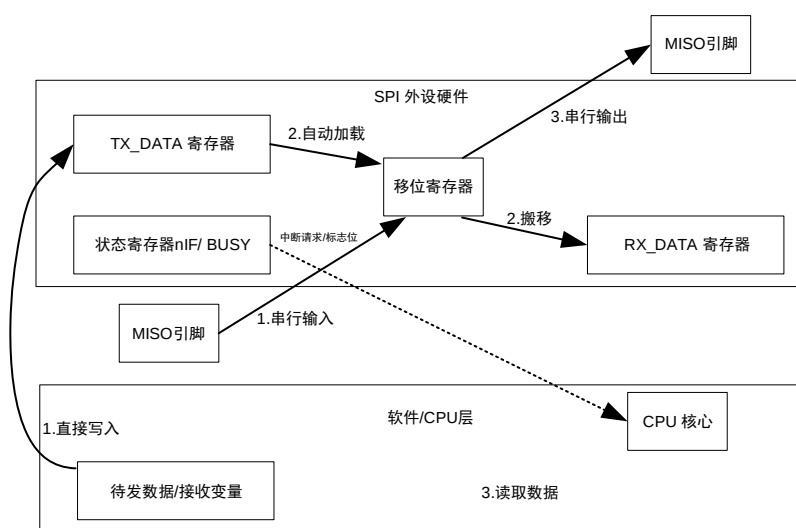
图 17-11 SPI CPU 传输数据流框图
