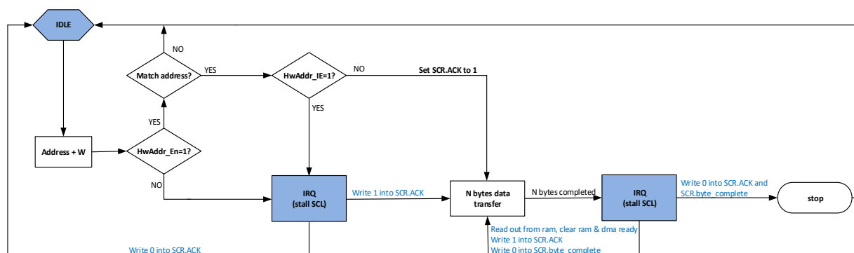
图 16-8 从模式下多字节接收示意图
