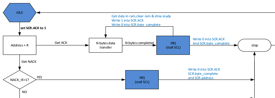
图 16-12 主模式下多字节接收示意图
