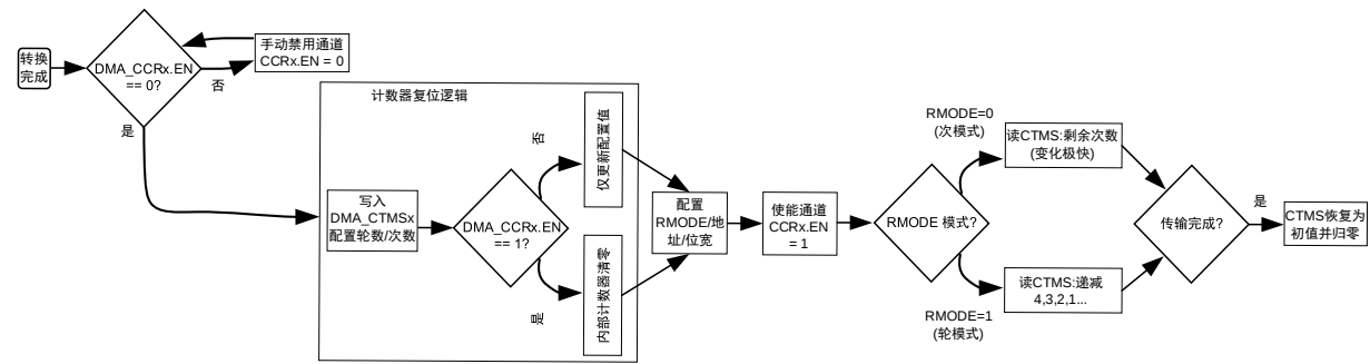
图 7-5 DMA 操作逻辑流程图
