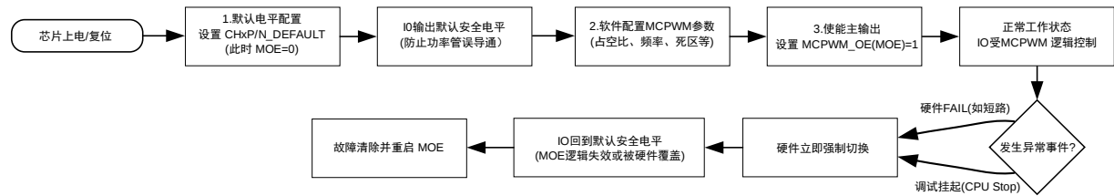
图 13-12 Fail 保护与输出控制流程图
