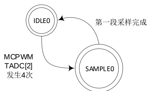
图 10-8 ADC 单段采样状态转移图
