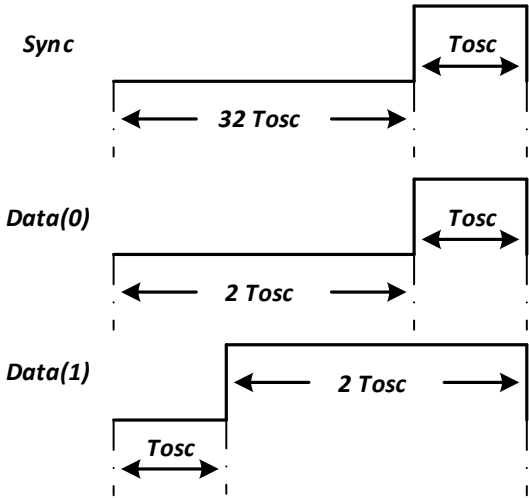
图 20-2 SIF 基本传输时序图
