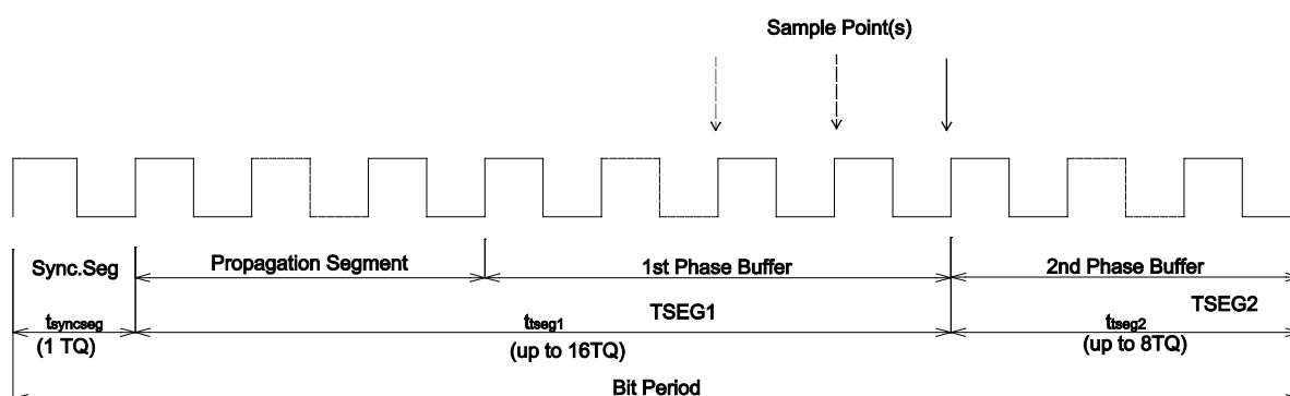
图 19-4 CAN 模块 Bit 周期介绍图
