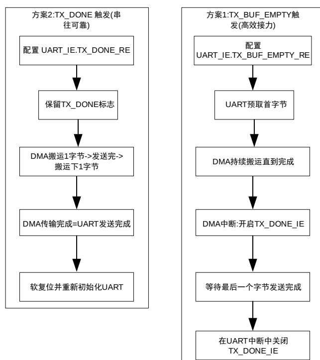
图 14-2 UART DMA 发送对比
