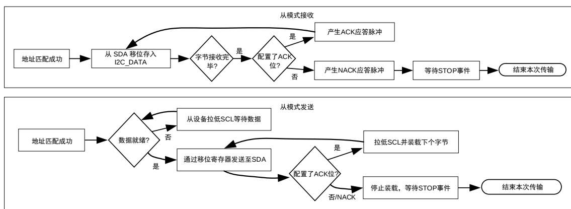
图 16-6 I2C 从模式（发送/接收/DMA）的逻辑流程图
