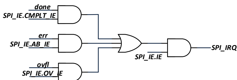
图 17-13 SPI 模块中断选信号产生图
