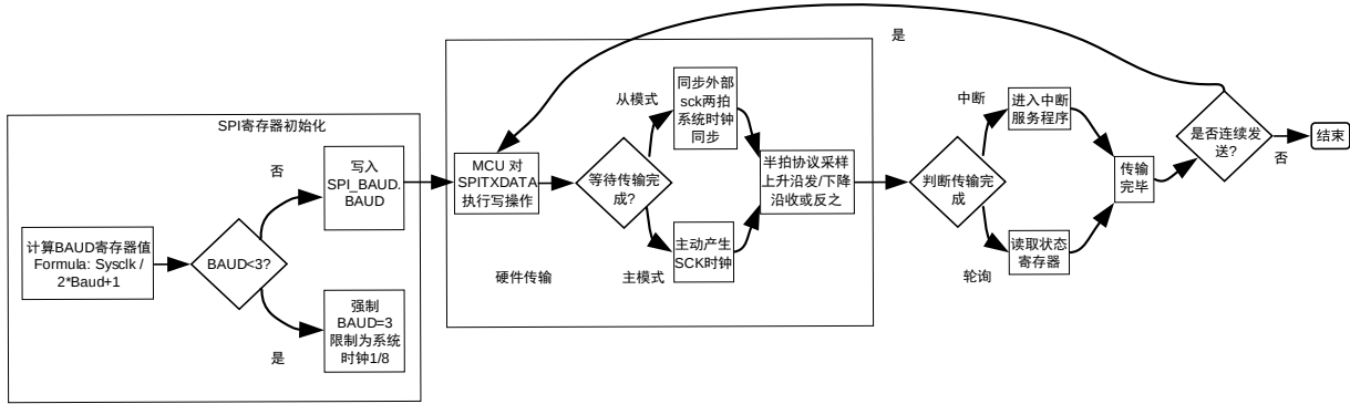
图 17-14 SPI 工作原理
