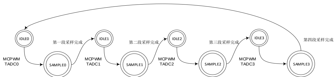
图 10-10 ADC 四段采样状态转移图
