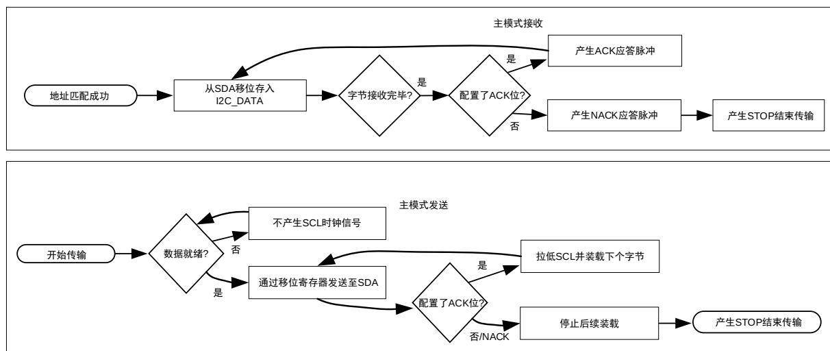
图 16-10 I2C 主模式发送和接收的逻辑流程图
