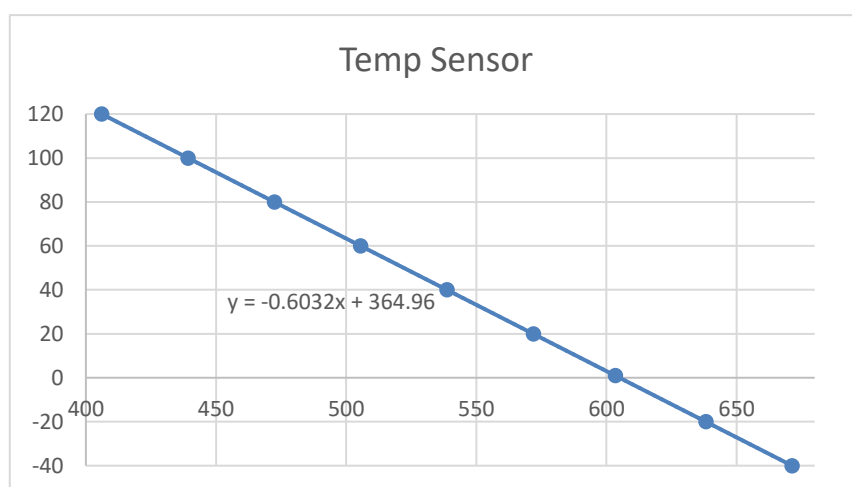
图 4-3 温度传感器曲线
