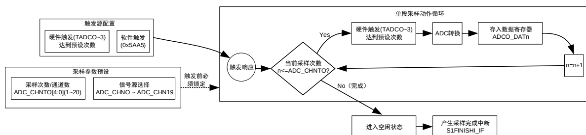
图 10-7 单段采样的数据与触发逻辑图
