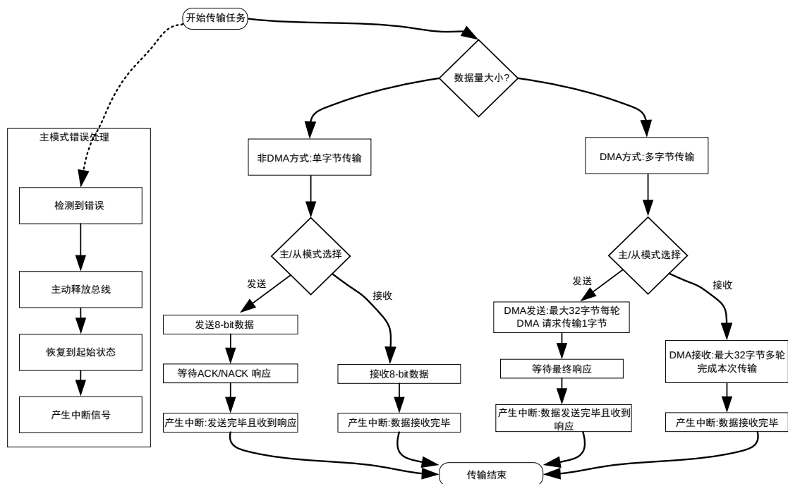
图 16-3 I2C 传输模式决策与执行流程图
