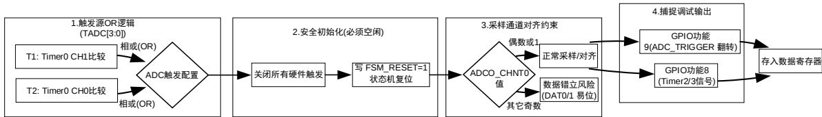
图 10-5 ADC 触发逻辑、状态机复位及采样通道对齐规则流程图
