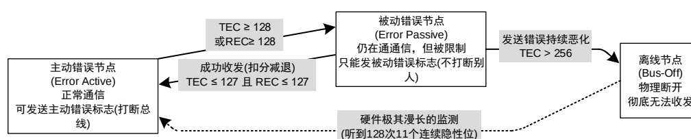
图 19-9 CAN 控制器三种错误状态切换原理图
