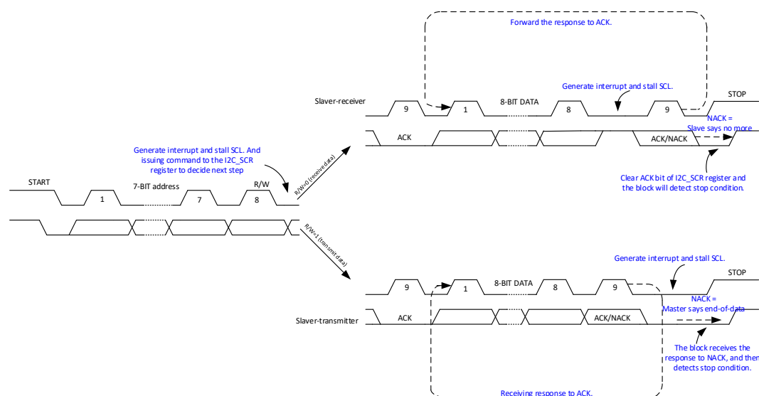
图 16-5 从模式下单字节传输示意图
