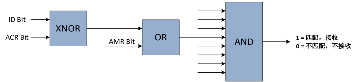
图 19-5 CAN 模块 ID 滤波逻辑关系
