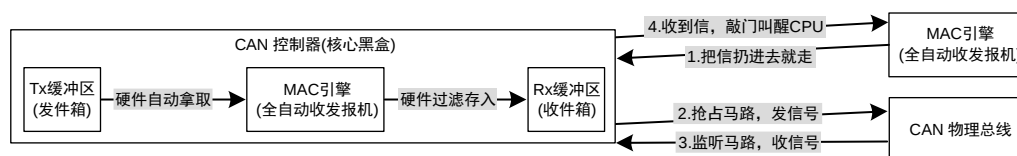
图 19-7 CAN 模块错误管理
