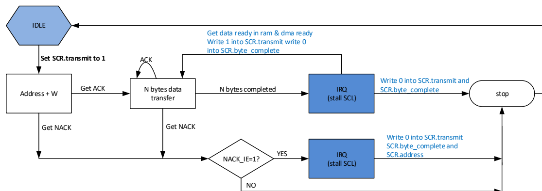
图 16-11 主模式下多字节发送示意图
