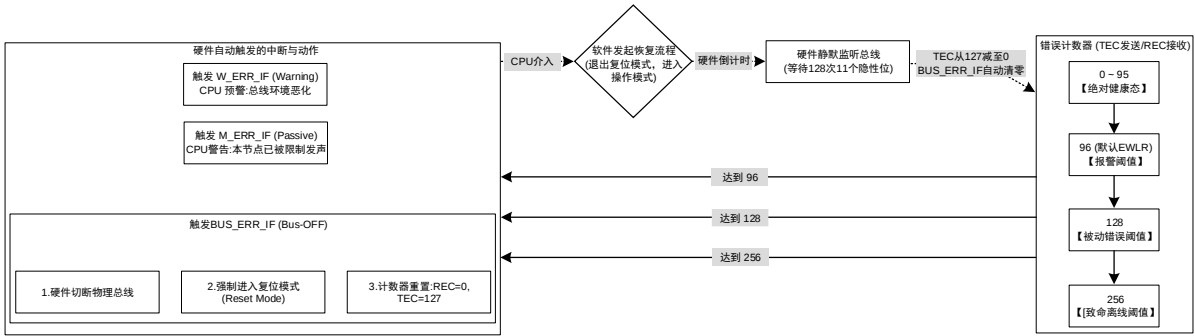
图 19-10 CAN 故障分级中断上报与总线关闭恢复流程
