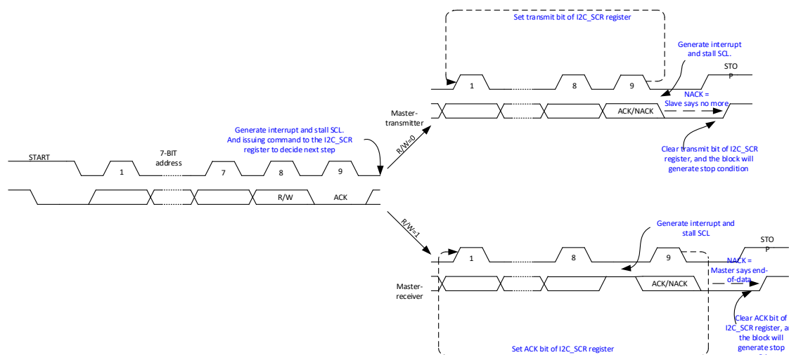
图 16-9 主模式下单字节传输示意图
