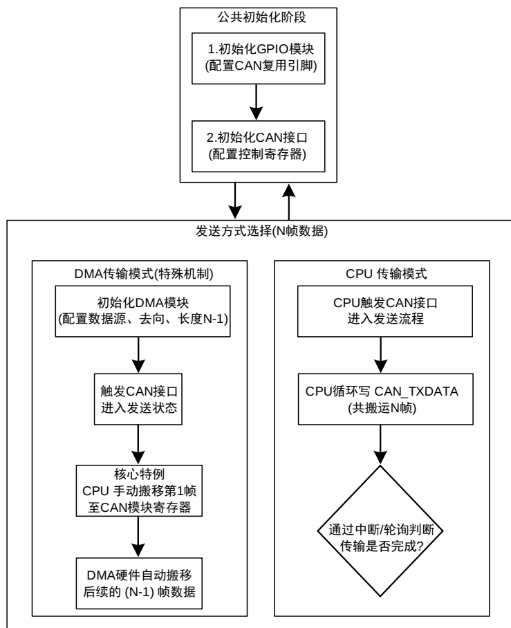
图 19-2 CAN 多帧数据 DMA 与 CPU 发送流程
