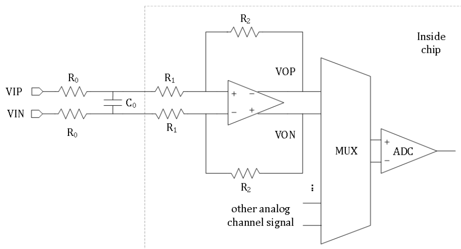
图 4-2 放大器框图
