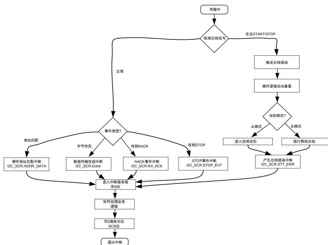
图 16-14 I2C 总线错误处理及中断管理流程图
