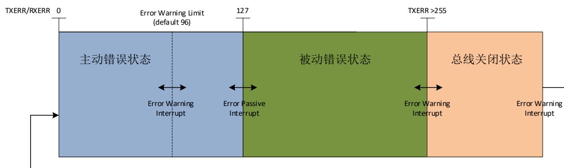
图 19-8 CAN 模块错误管理
