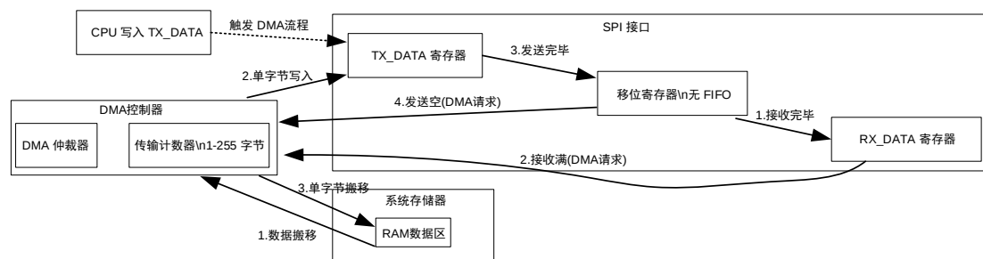
图 17-10 SPI DMA 数据流与握手逻辑框图
