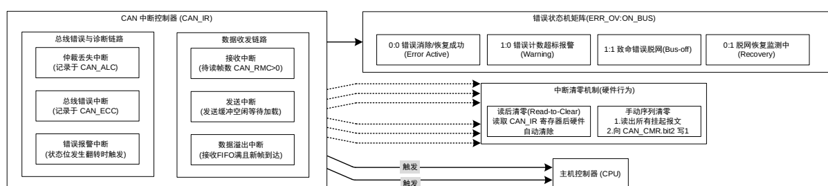
图 19-3 CAN 模块中断处理与状态机架构
