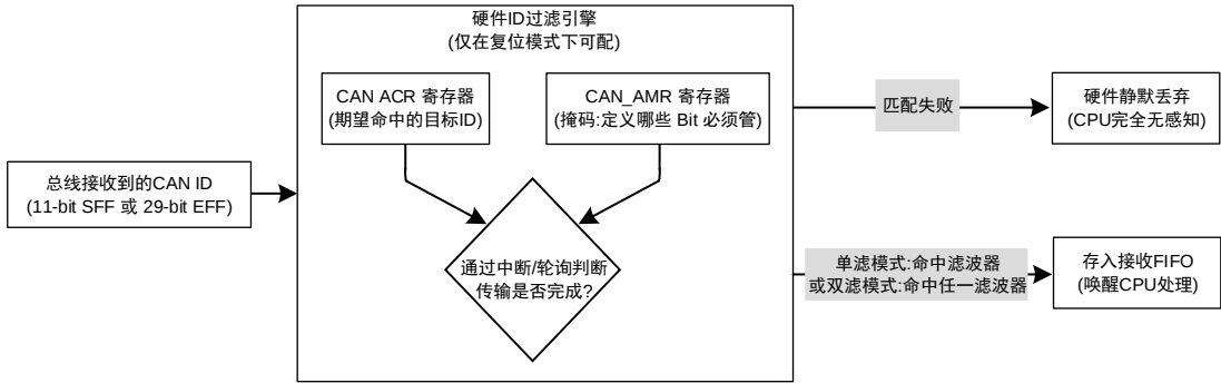
图 19-6 CAN 硬件 ID 过滤接收判断流程
