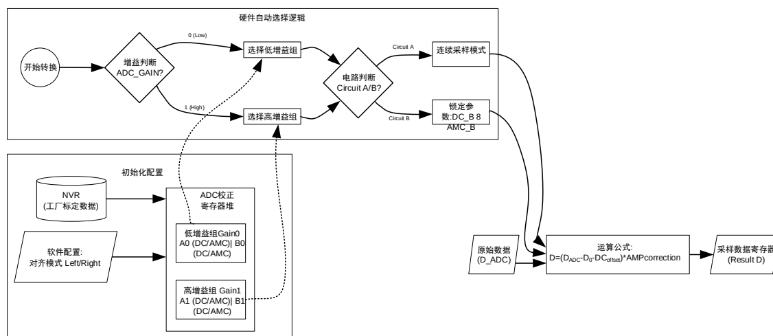
图 10-4 ADC 校正处理流程图
