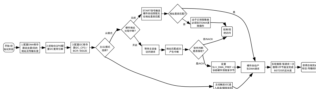
图 16-13 I2C 接口在大容量数据传输下的 DMA 配置与执行逻辑流程图
