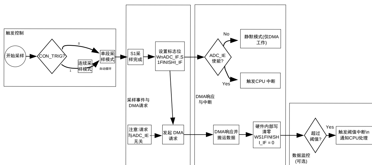
图 10-6 ADC DMA 与连续采样控制流程图
