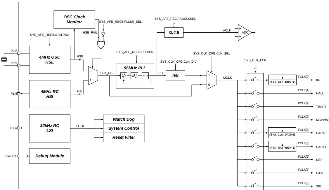
图 5-1 时钟架构
