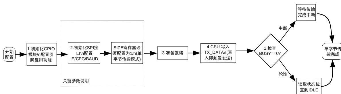
图 17-12 软件配置流程图
