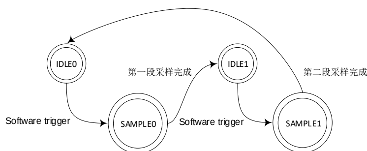
图 10-9 ADC 两段采样状态转移图
