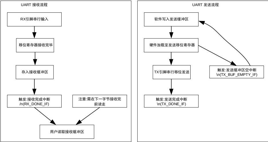
图 14-1 UART 发送与接收中断
