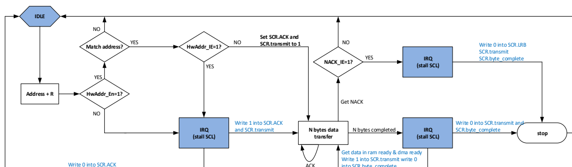
图 16-7 从模式下多字节发送示意图
