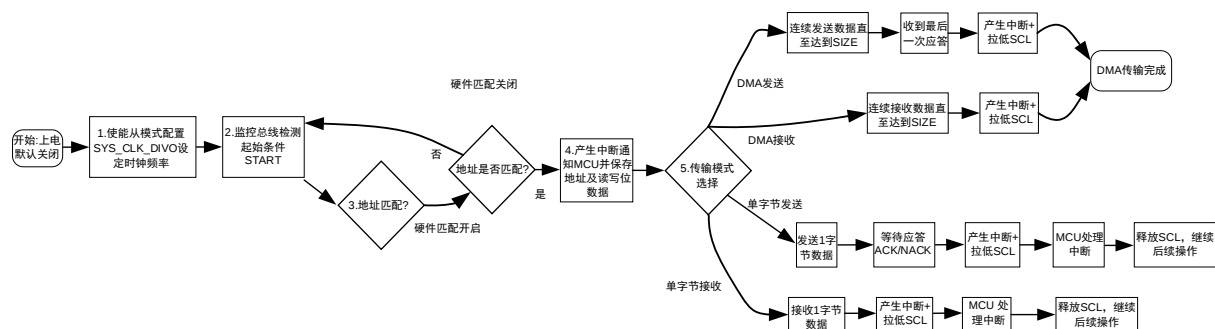
图 16-4 I2C 从模式工作流程图
