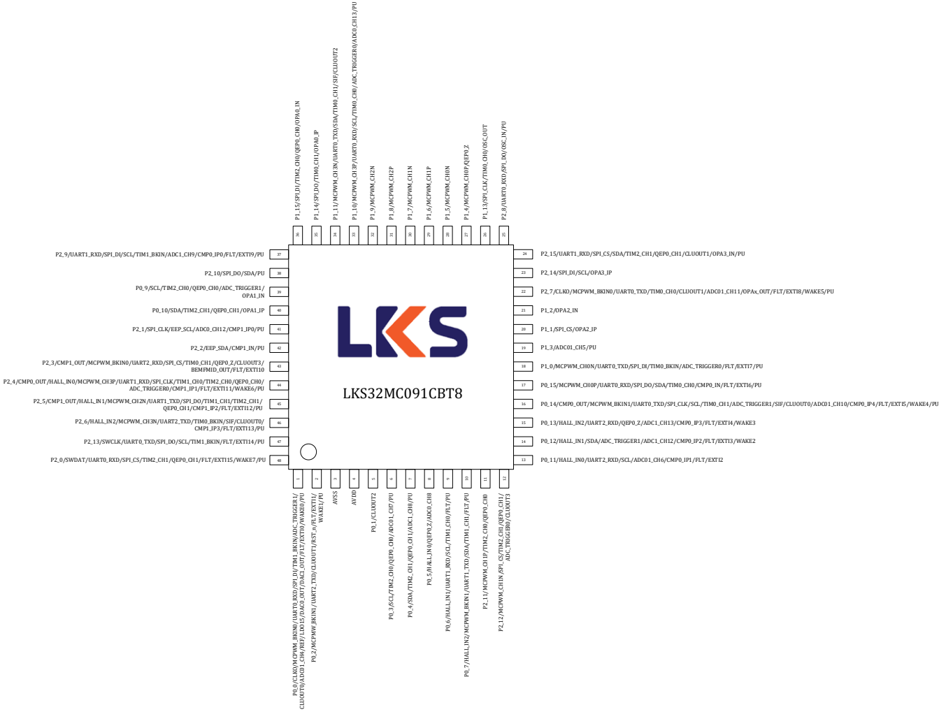
图 3-1 LKS32MC091CBT8/LKS32MC091C8T8 管脚分布图
