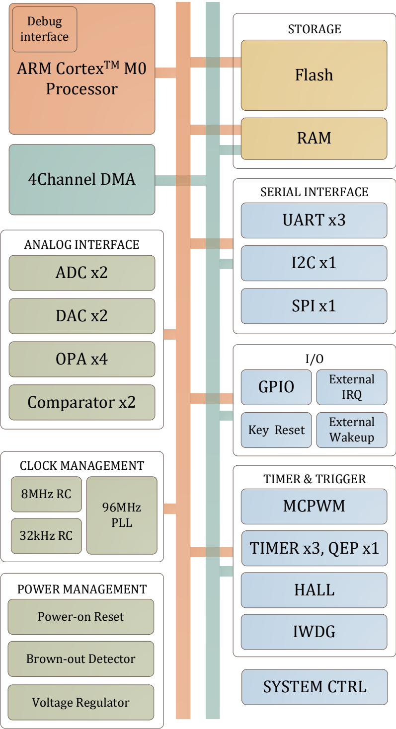
图 1-2 LKS32MC09x 系统资源框图
