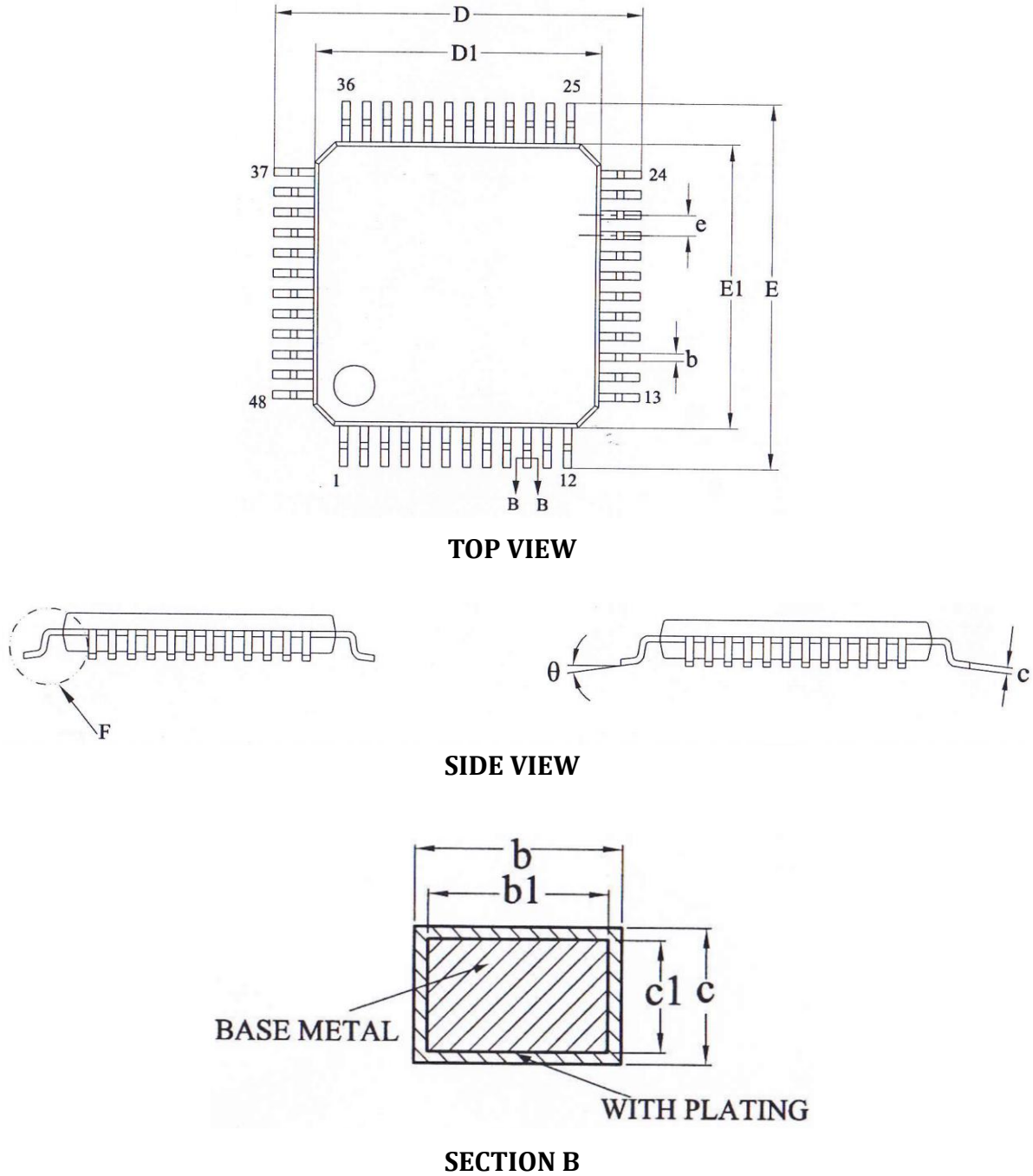
图 4-1 LKS32MC091CBT8/LKS32MC091C8T8 封装图示
