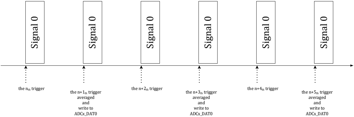
图 12-6 过采样转换时序示例 1
