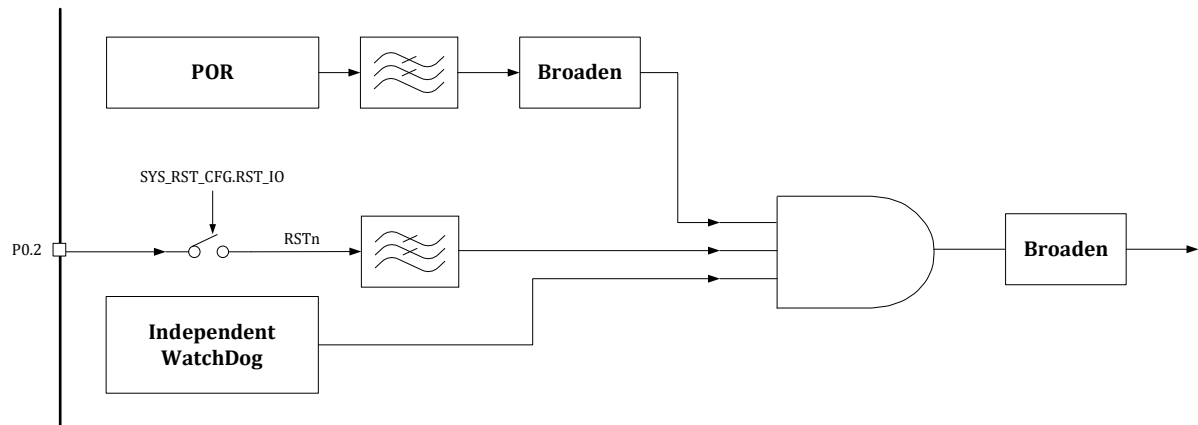
图 6-2 复位架构
