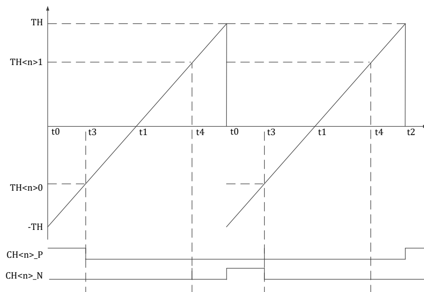
图 14-11MCPWM 时序 TH< n >0 和 TH< n >1 边沿对齐推挽模式
