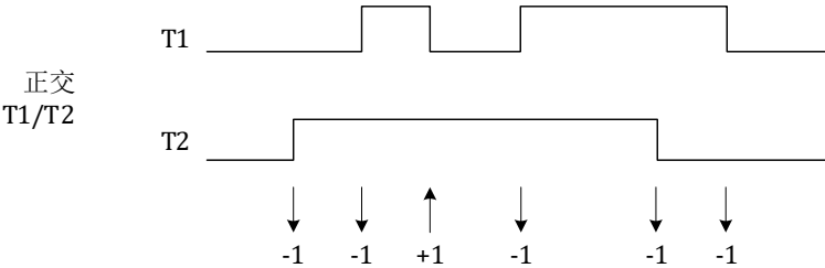
图 13-15 编码器在 T1 或 T2 时刻计数的正交编码信号计数情况
