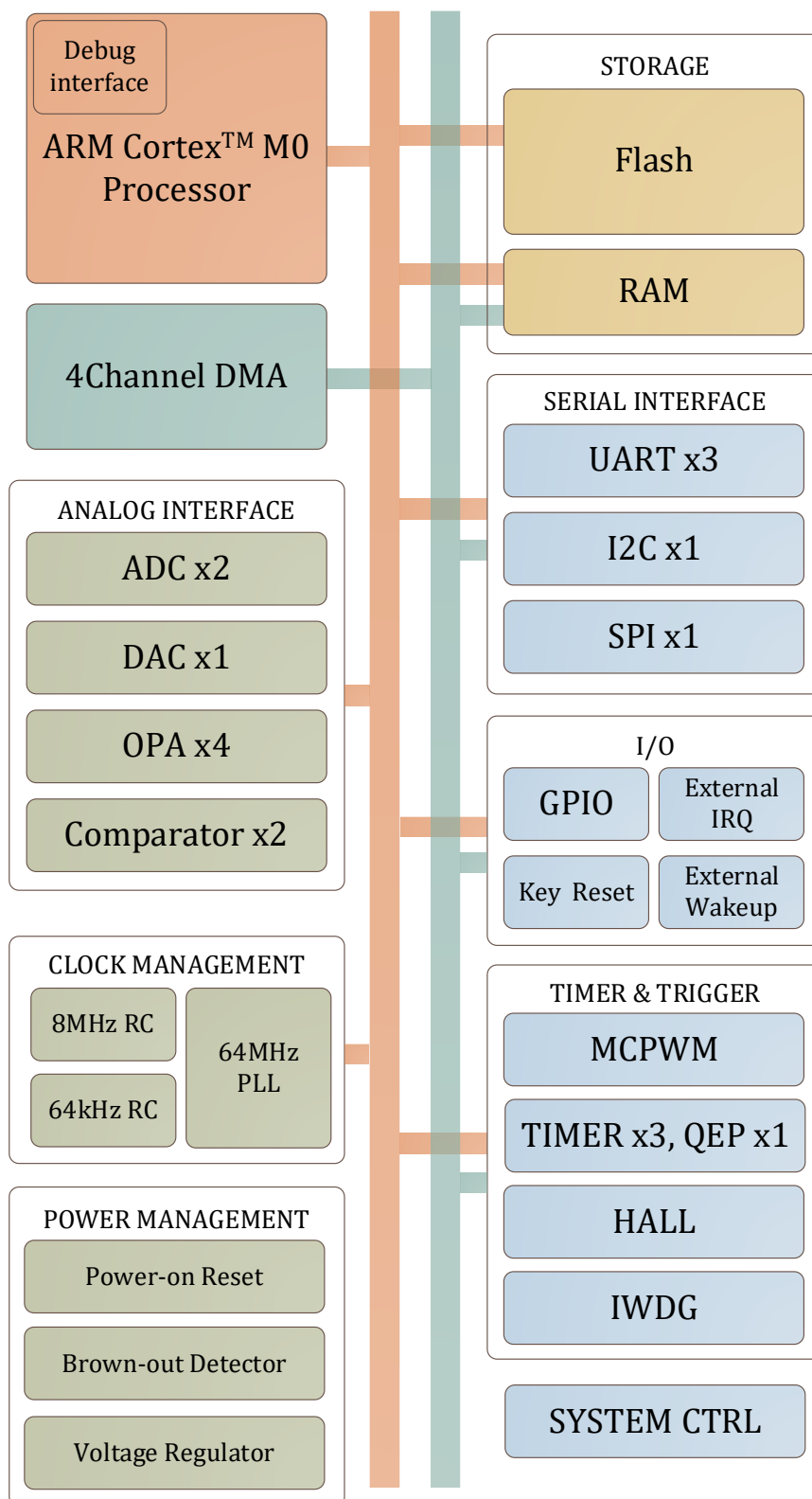
图 2-1 LKS32MC09x 系统框图
