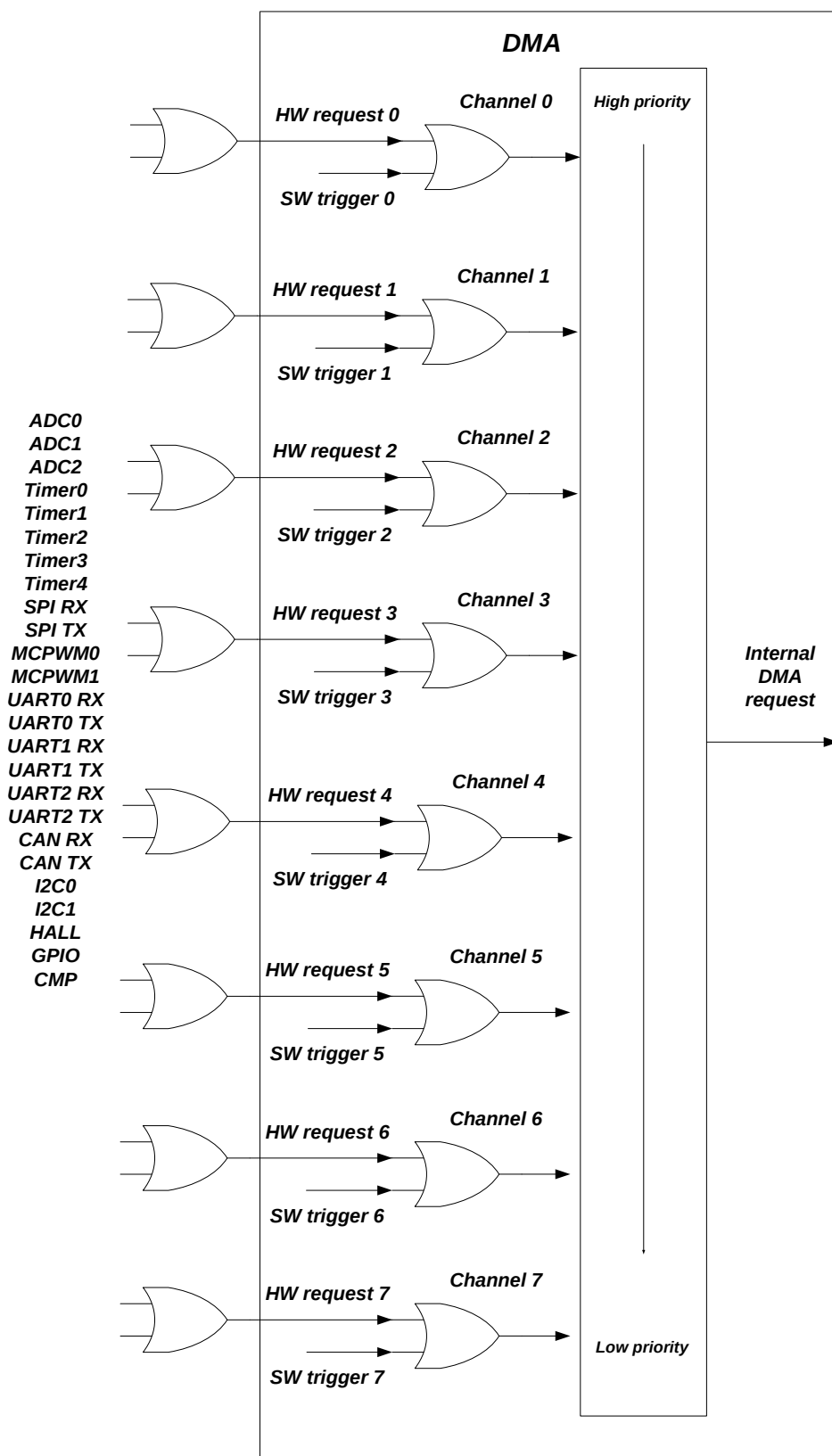
图 8-8 DMA 通道优先级
