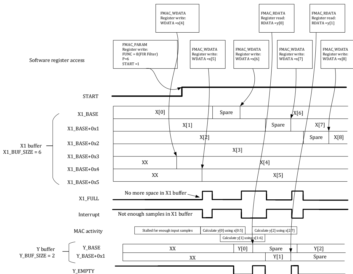
图 12-15 滤波器操作示例 2
