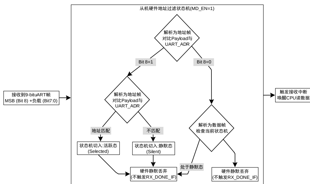
图 17-4 从机 9-bit UART 地址帧过滤状态机处理流程
