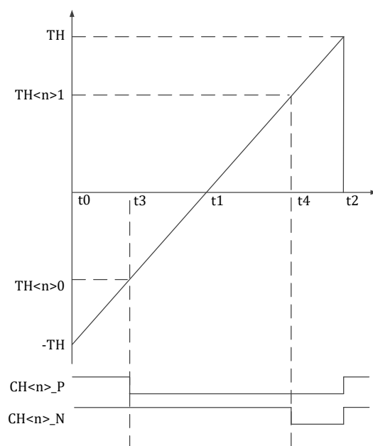
图 16-13 MCPWM 时序边沿对齐模式
