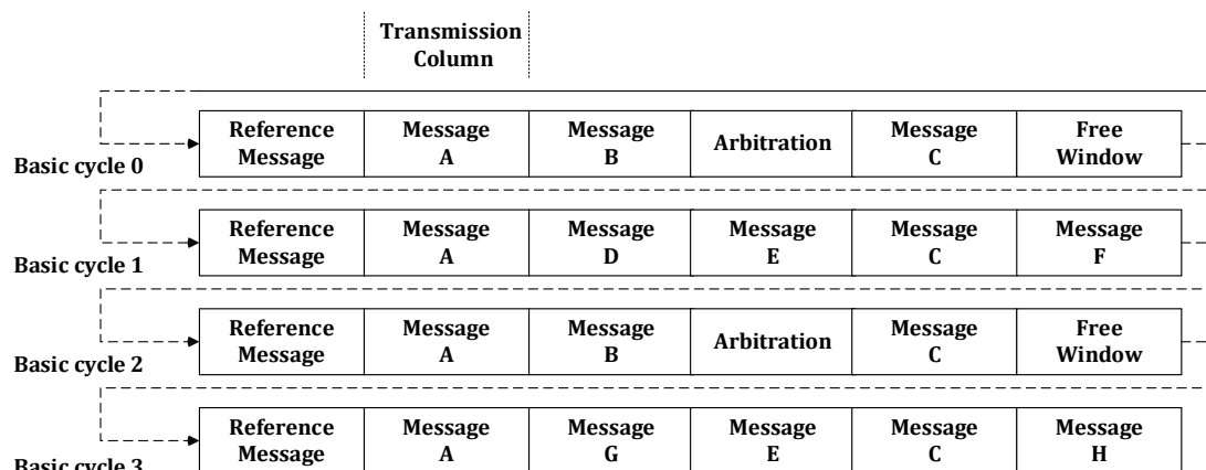
图 21-15 TTCAN 时空矩阵示例
