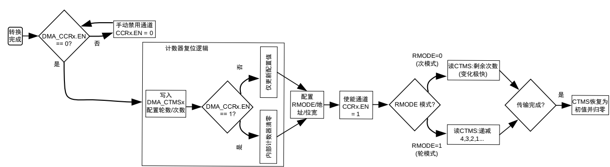
图 8-9 DMA 操作逻辑流程图
