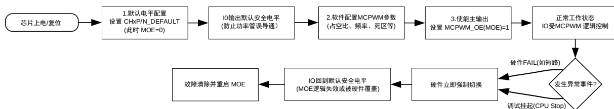
图 16-16 Fail 保护与输出控制流程图
