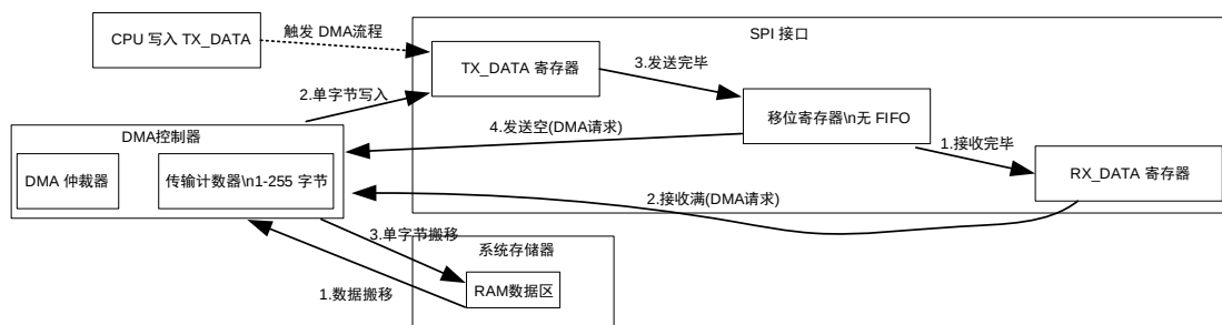
图 19-6 SPI DMA 数据流与握手逻辑框图
