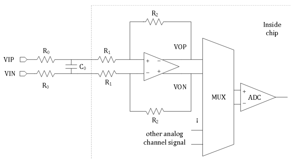
图 5-2 放大器框图
