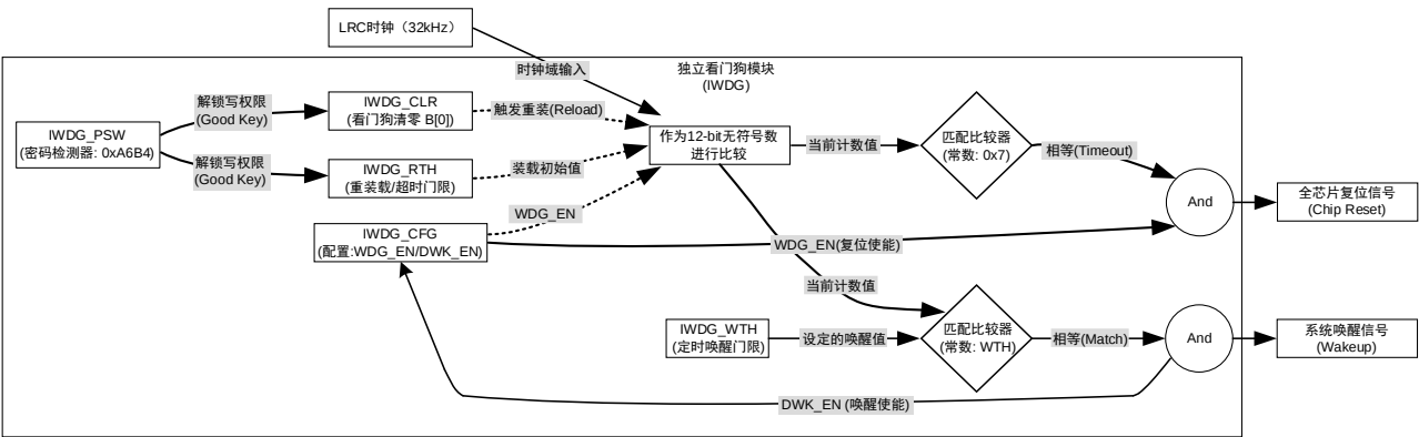
图 23-1 IWDG 工作原理和信号流向
