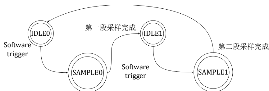
图 13-11 ADC 两段采样状态转移图
