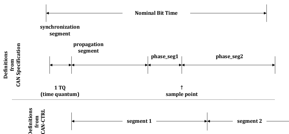
图 21-16 CAN 位时序规范
