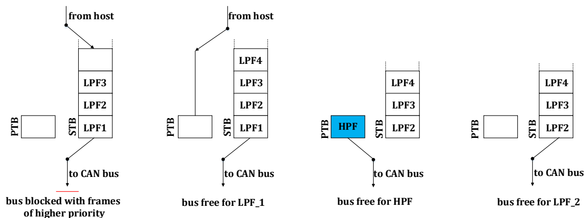
图 21-5 发送缓冲器应用示例 (TSALL=1)
