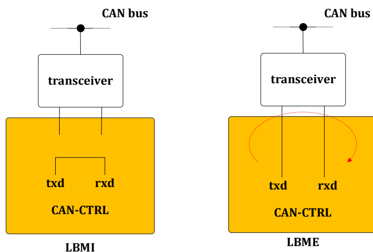
图 21-14 环回模式：内部和外部
