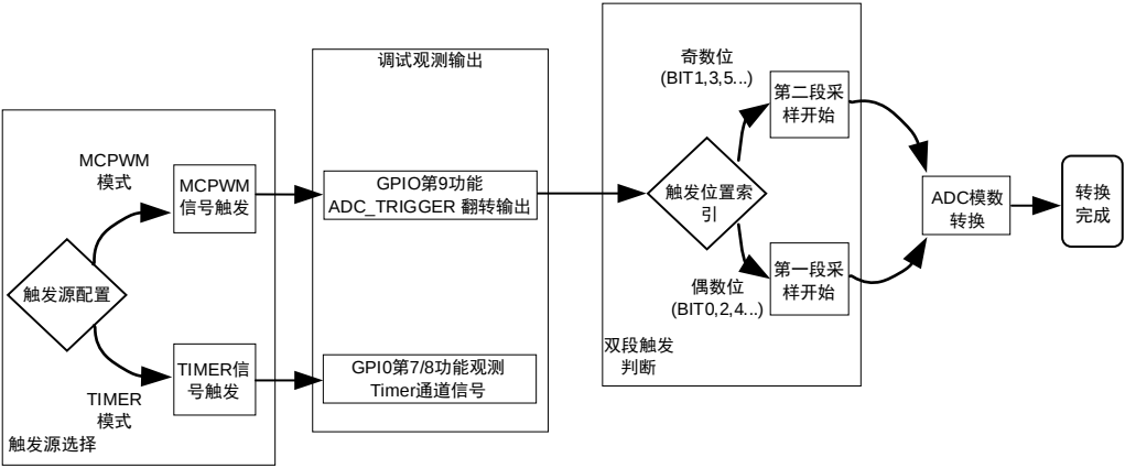
图 13-7 ADC 触发与调试观测流程图
