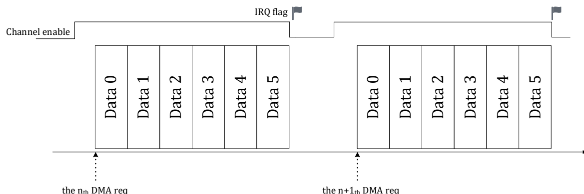
图 8-2 RMODE=0 DMA 传输情况
