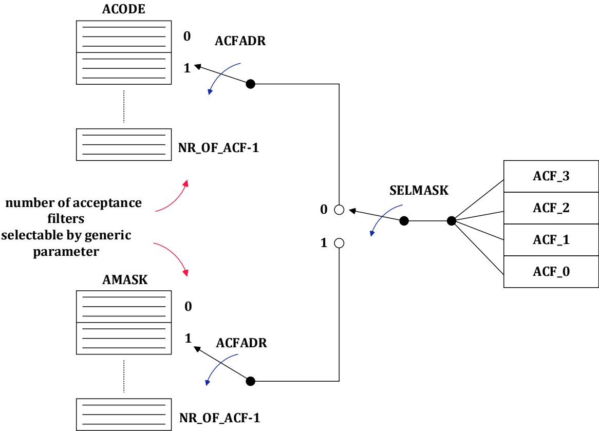
图 21-10 接收过滤器
