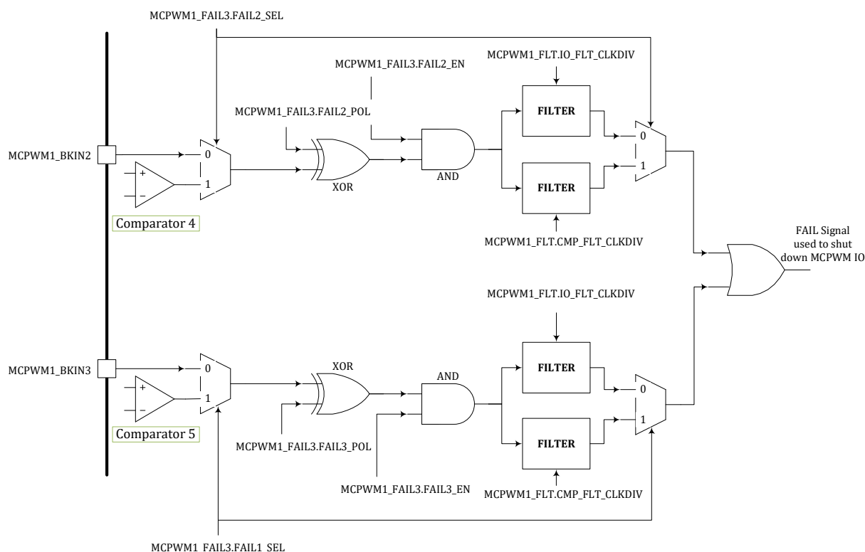
图 16-8 MCPWM1 FAIL2/3 逻辑示意图
