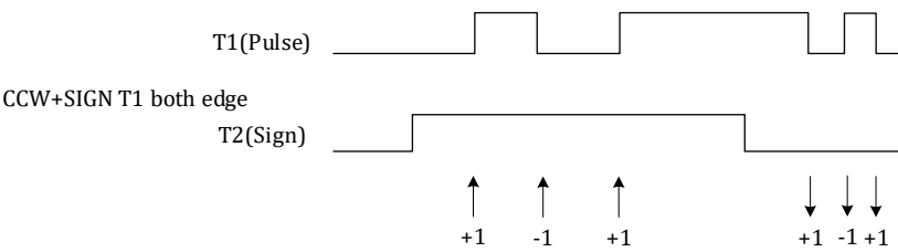
图 14-8 编码器在 T1 上升下降沿都计数的符号加脉冲信号计数情况
