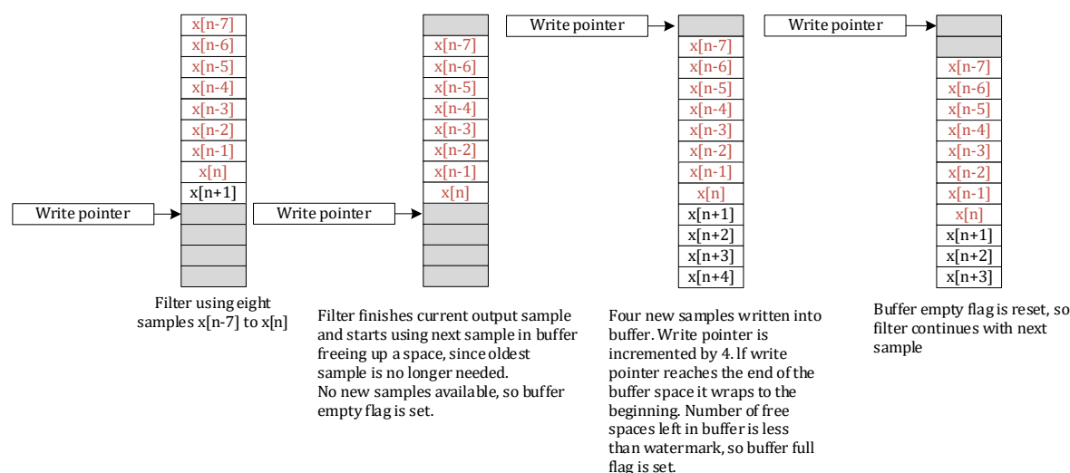
图 12-5 循环输入 buffer 的读写操作
