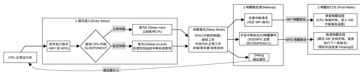
图 24-2 常规休眠模式进入与唤醒流程图
