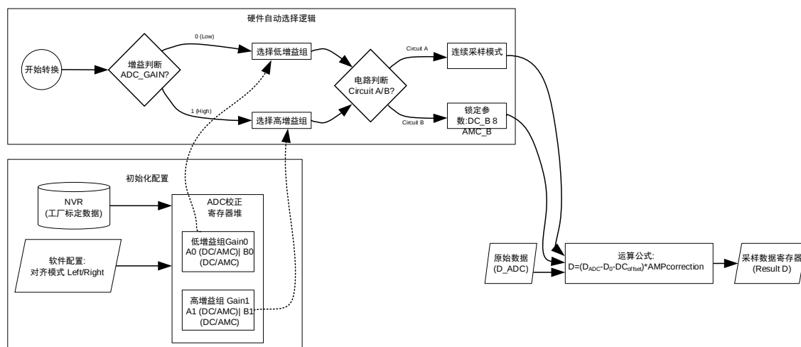
图 13-3 ADC 校正处理流程图
