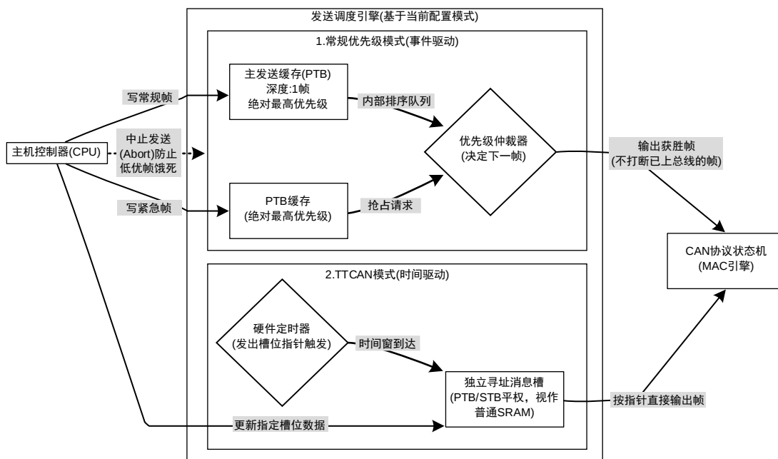
图 21-6 CAN Tx 常规事件与 TTCAN 时间驱动机制
