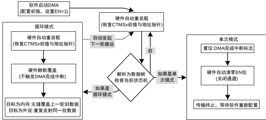
图 8-7 DMA 循环 / 单次传输模式硬件处理逻辑
