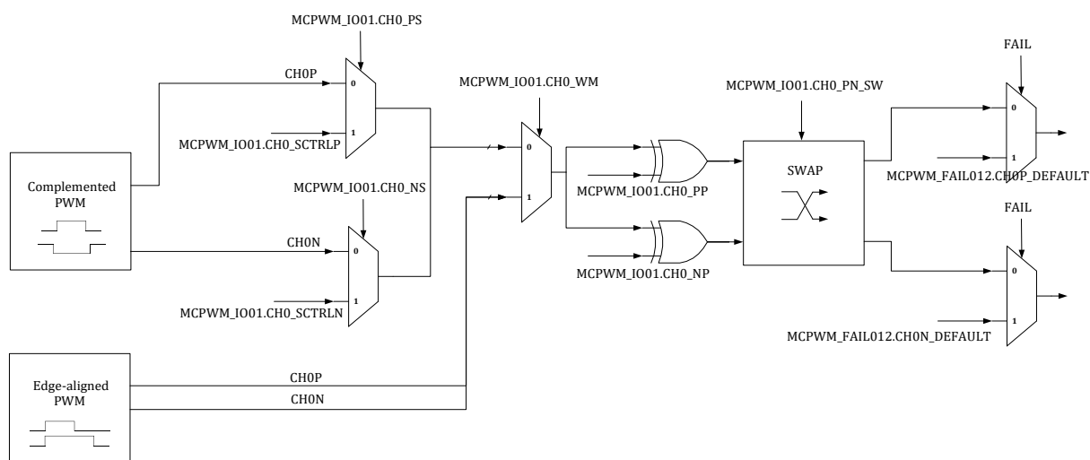
图 16-10 IO Driver 模块数据流程图
