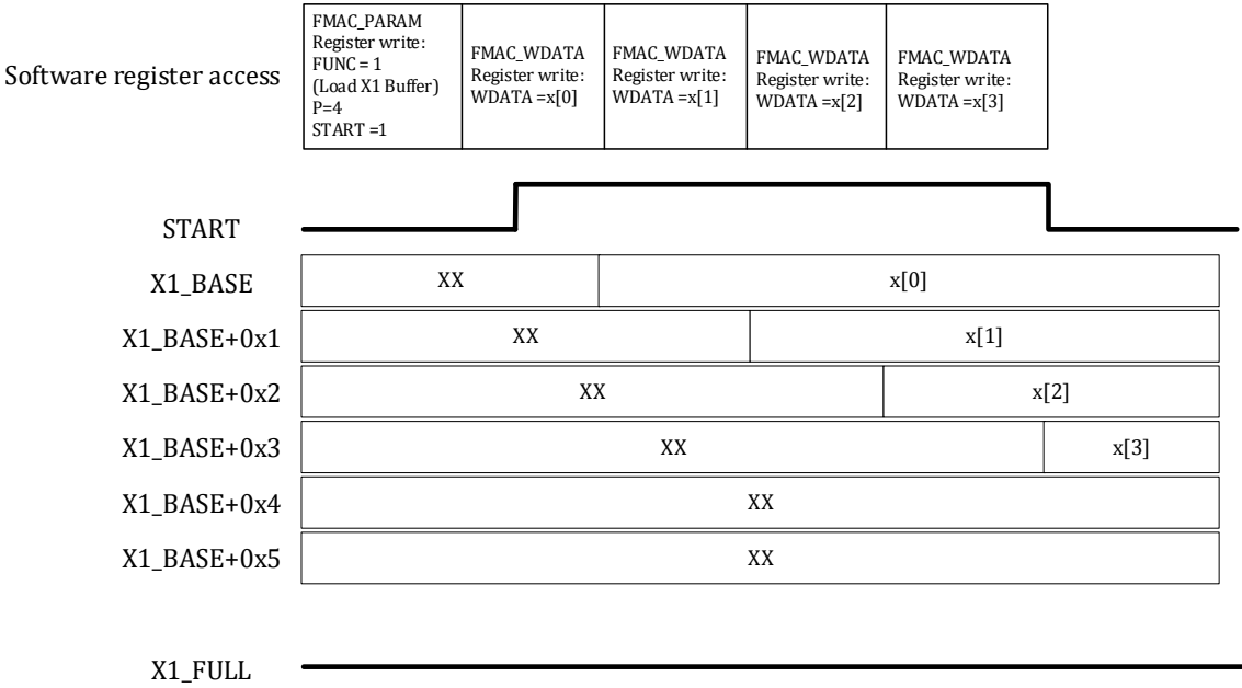
图 12-13 X1 buffer 初始化
