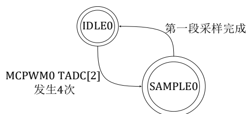
图 13-9 ADC 单段采样状态转移图
