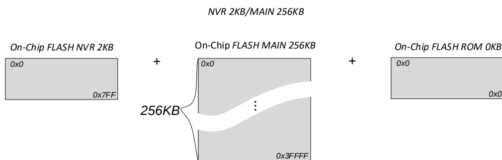
图 7-1 On-Chip FLASH 存储体空间划分框图
