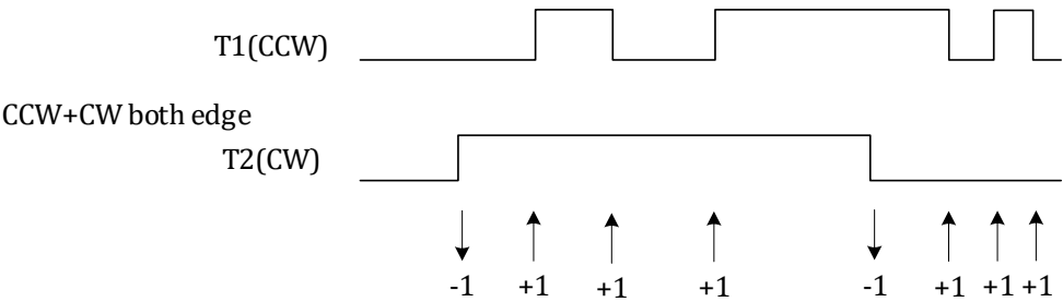
图 14-11 编码器在 T1/T2 上升下降沿计数的 CCW/CW 双脉冲信号计数情况
