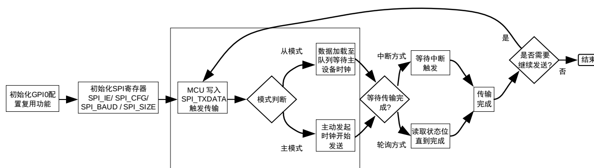
图 19-7 SPI 传输的软件配置与操作流程
