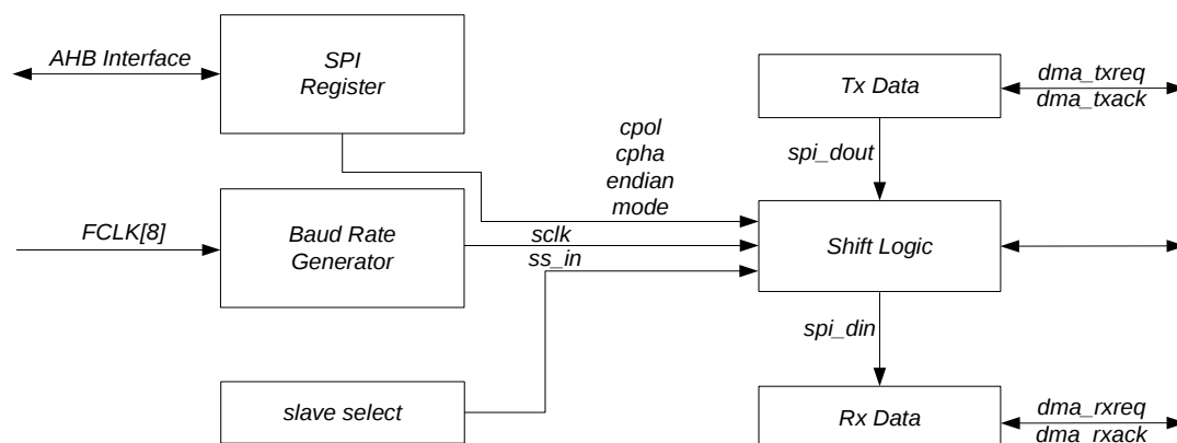
图 19-1 SPI 模块结构框图
