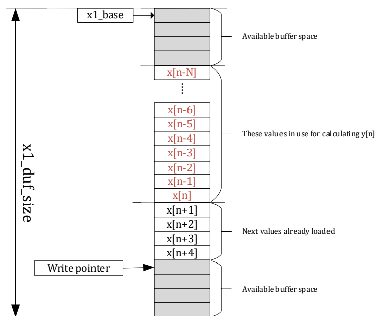
图 12-4 循环输入 buffer
