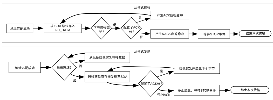
图 18-6 I2C 从模式（发送/接收）的逻辑流程图
