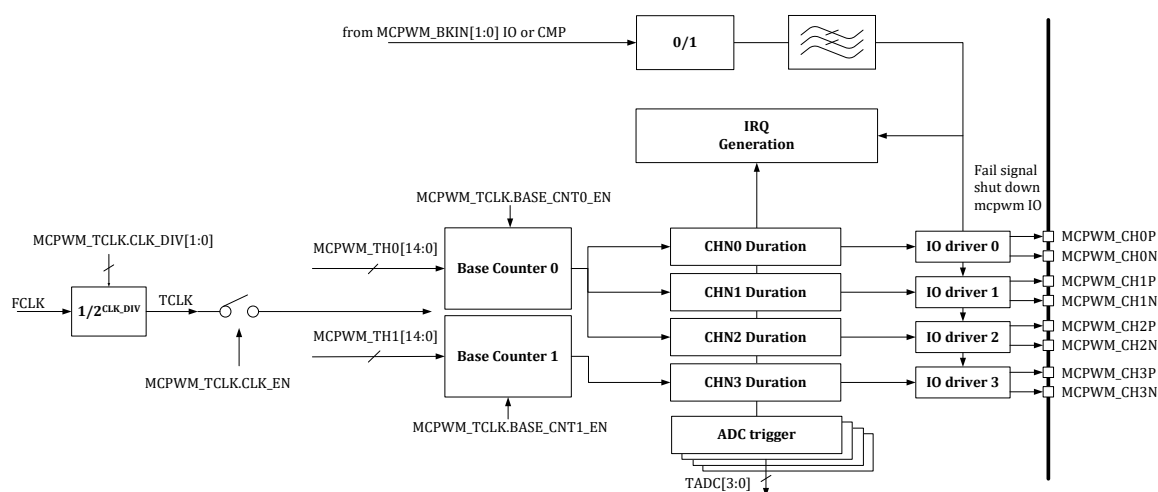
图 16-1 MCPWM 模块框图
