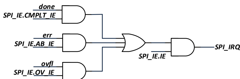
图 19-8 SPI 模块中断选信号产生图
