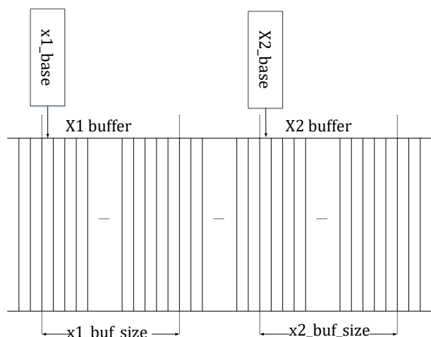
图 12-3 输入缓存区域
