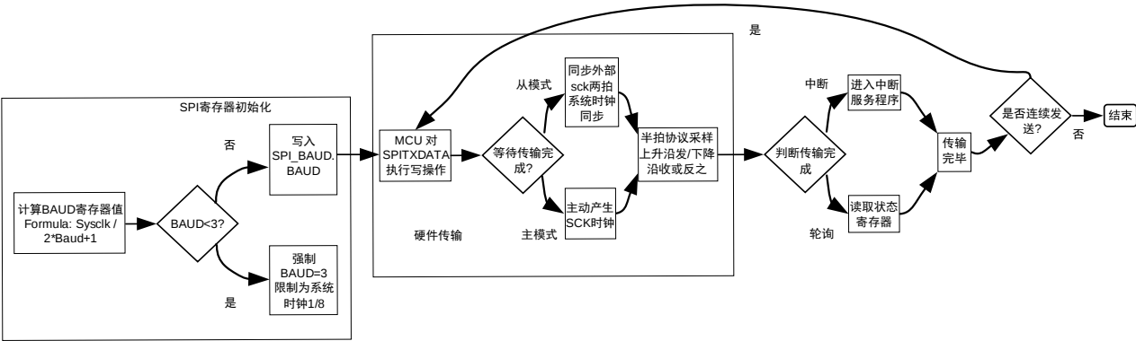
图 19-9 SPI 工作原理
