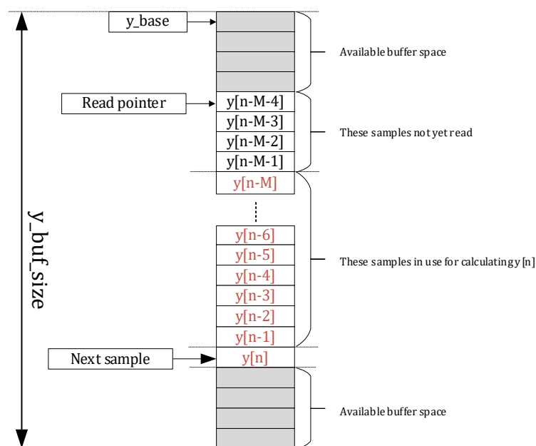
图 12-6 循环输出 buffer
