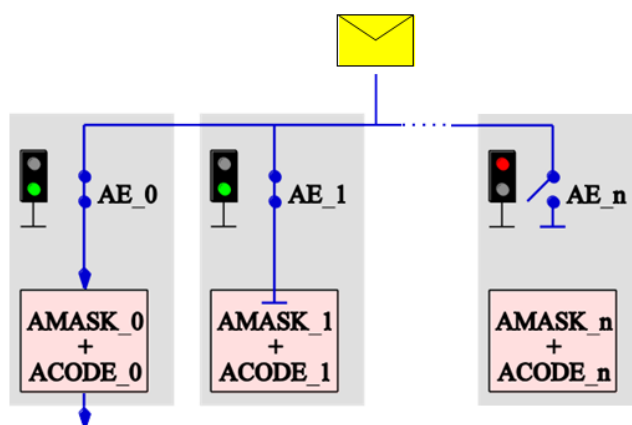
图 21-11 接收过滤示例
