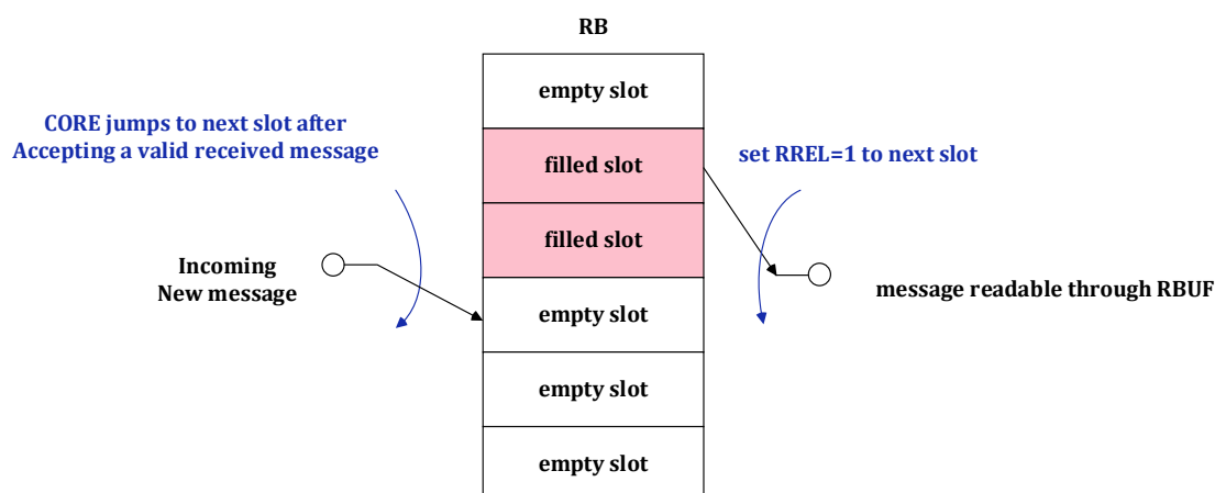
图 21-8 类似 FIFO 的 RB 示意图（6 个消息槽示例）
