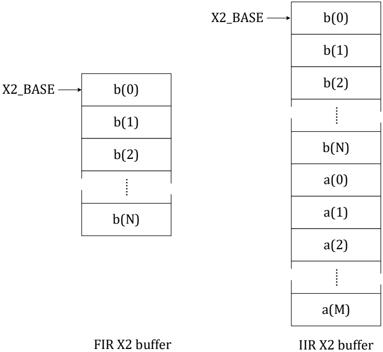
图 12-8 FIR 和 IIR 滤波器 x2 buffer 系数排列
