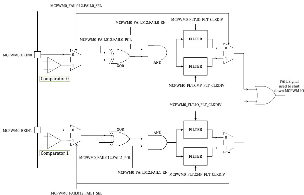
图 16-5 MCPWM0 FAIL0/1 逻辑示意图
