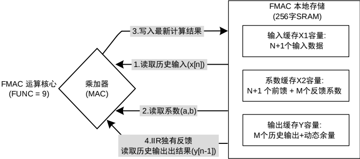
图 12-12 FMAC 工作模式下 IIR 滤波器数据交互架构
