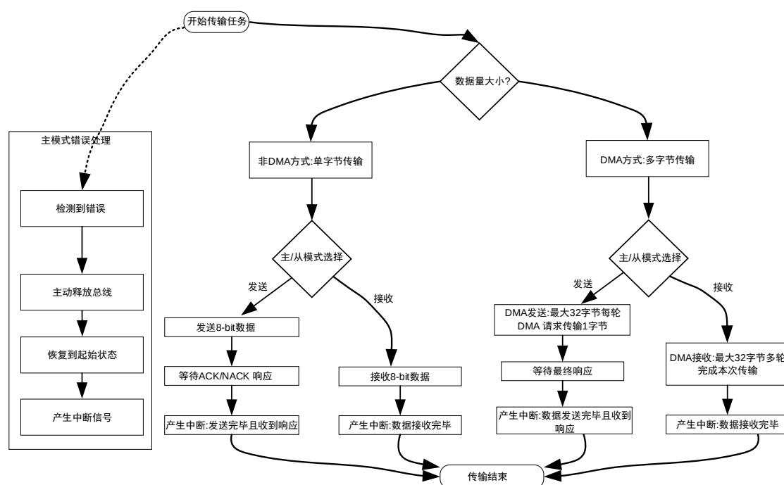
图 18-3 I2C 传输模式决策与执行流程图
