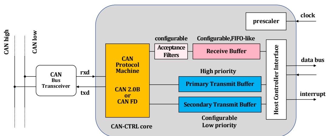
图 21-1 CAN 总线的连接和 CAN 总线控制器的主要特性
