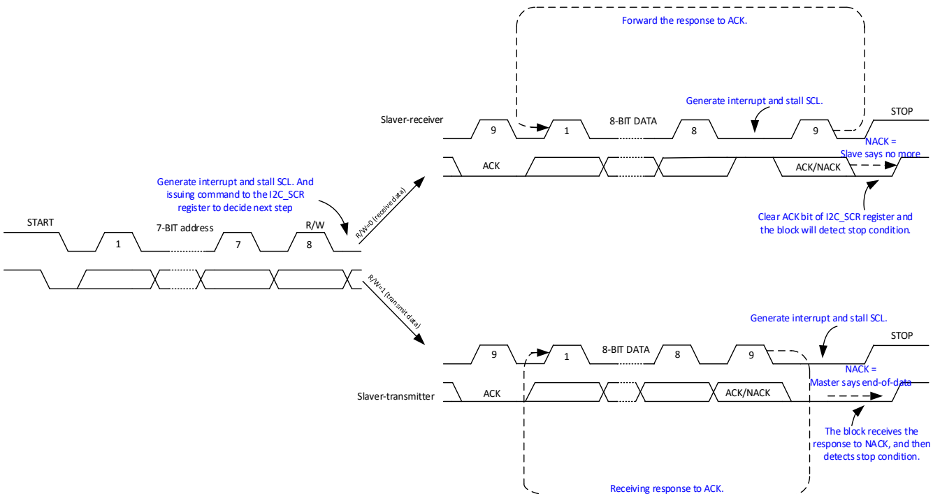
图 18-5 从模式传输示意图
