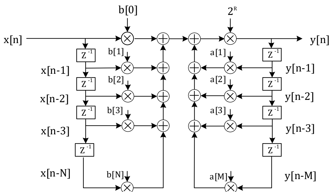
图 12-10 直接 1 型 IIR 滤波器结构
