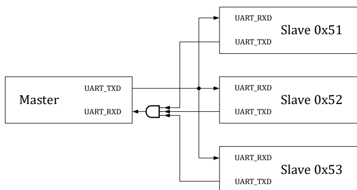
图 17-3 UART 多机通讯互联拓扑
