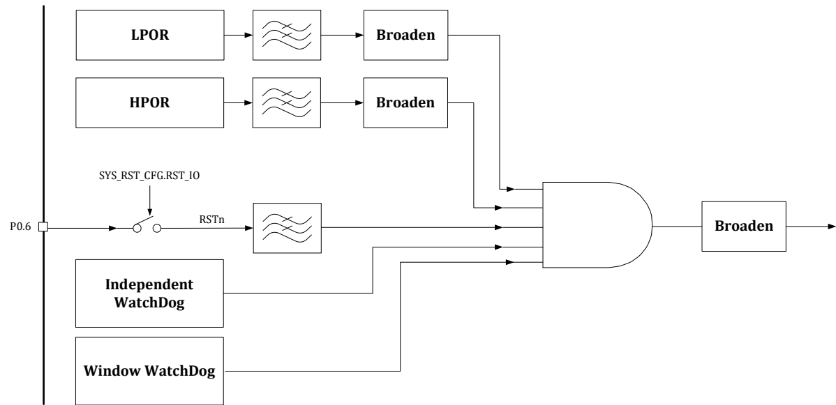
图 6-2 复位架构
