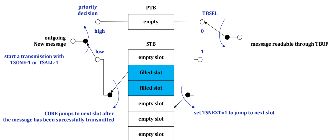
图 21-13 FIFO 模式下的 PTB 和 STB 示意图（空 PTB 和 6 个 STB 消息槽）
