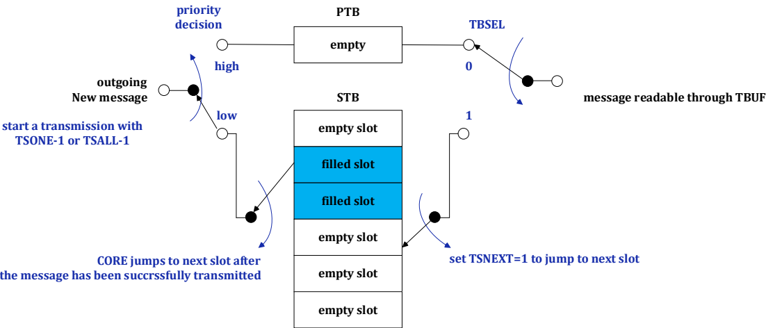
图 21-9 FIFO 模式下的 PTB 和 STB 示意图 (6 个 STB 消息槽)
