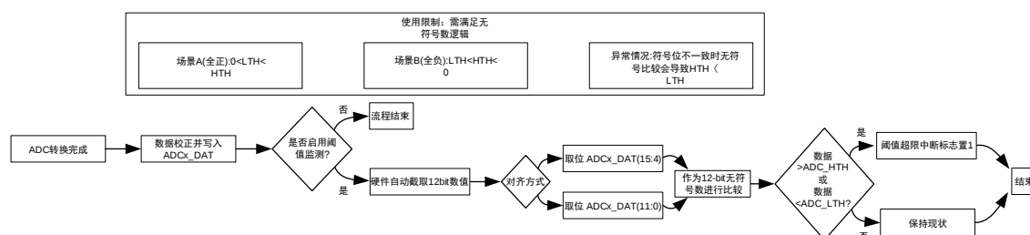
图 13-4 ADC 校正处理流程图
