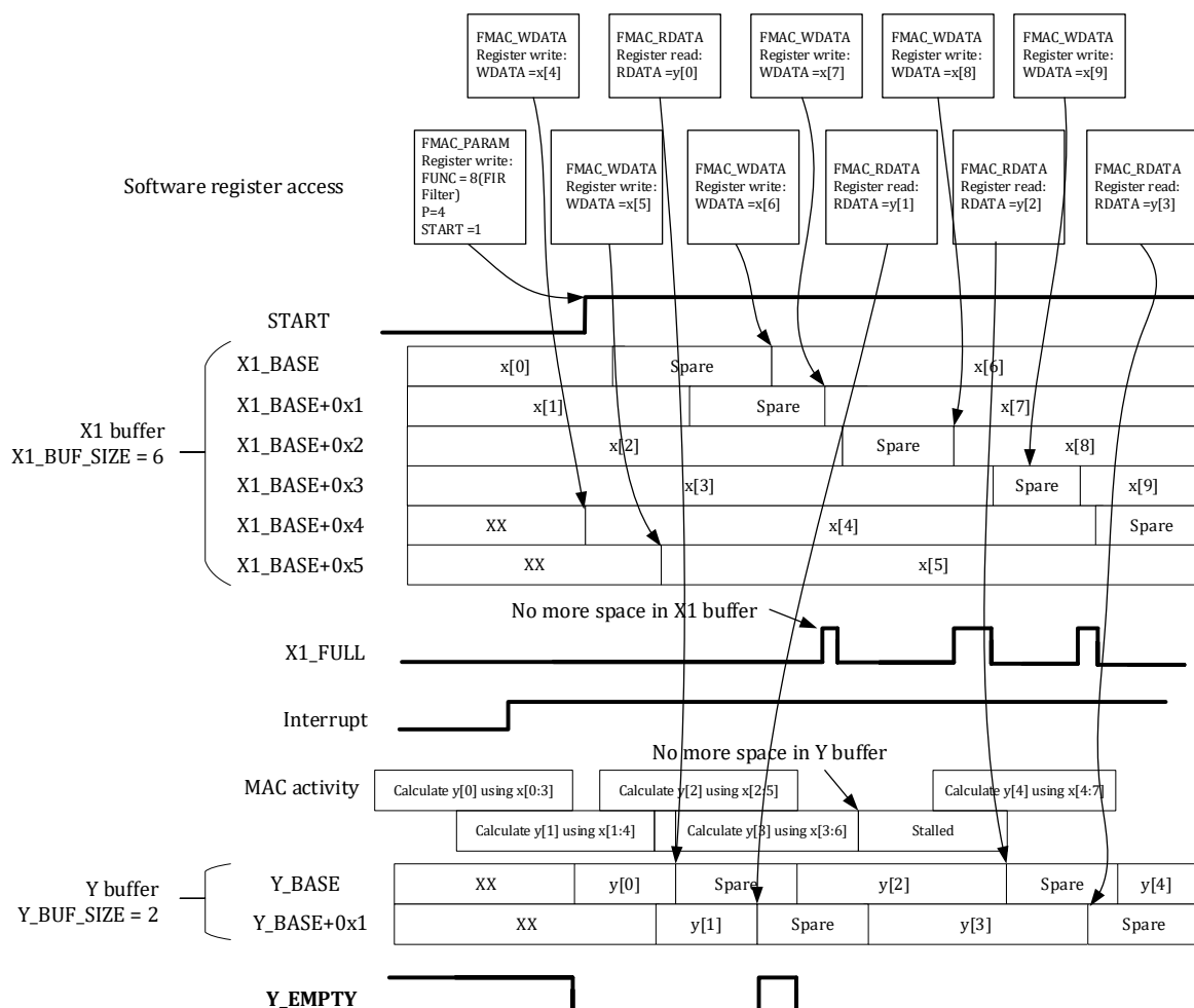
图 12-14 滤波器操作示例 1
