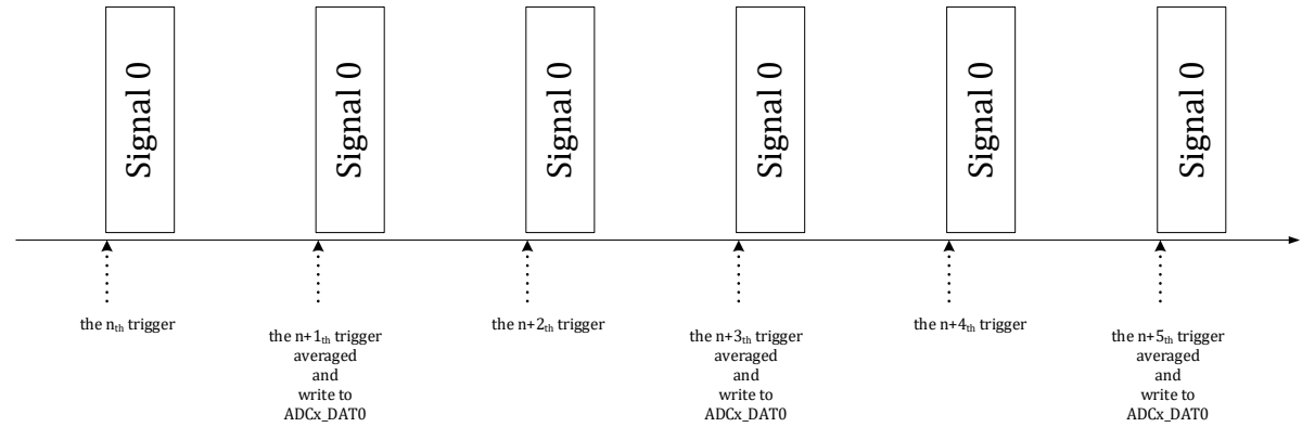
图 13-6 过采样转换时序示例 2
