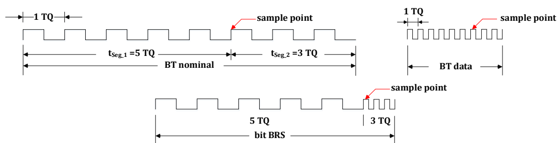
图 21-18 比特 BRS 的波特率切换 S\_PRESC \neq F\_PRESC
