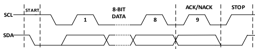
图 18-2 基本 I2C 传输时序图
