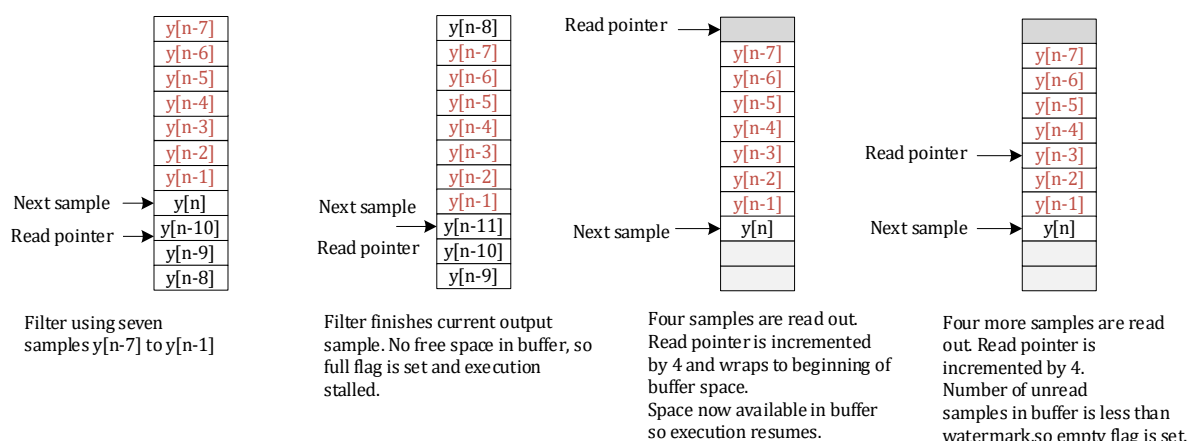
图 12-7 循环输出 buffer 读写操作
