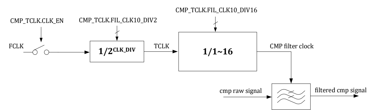
图 20-1 比较器滤波时钟产生
