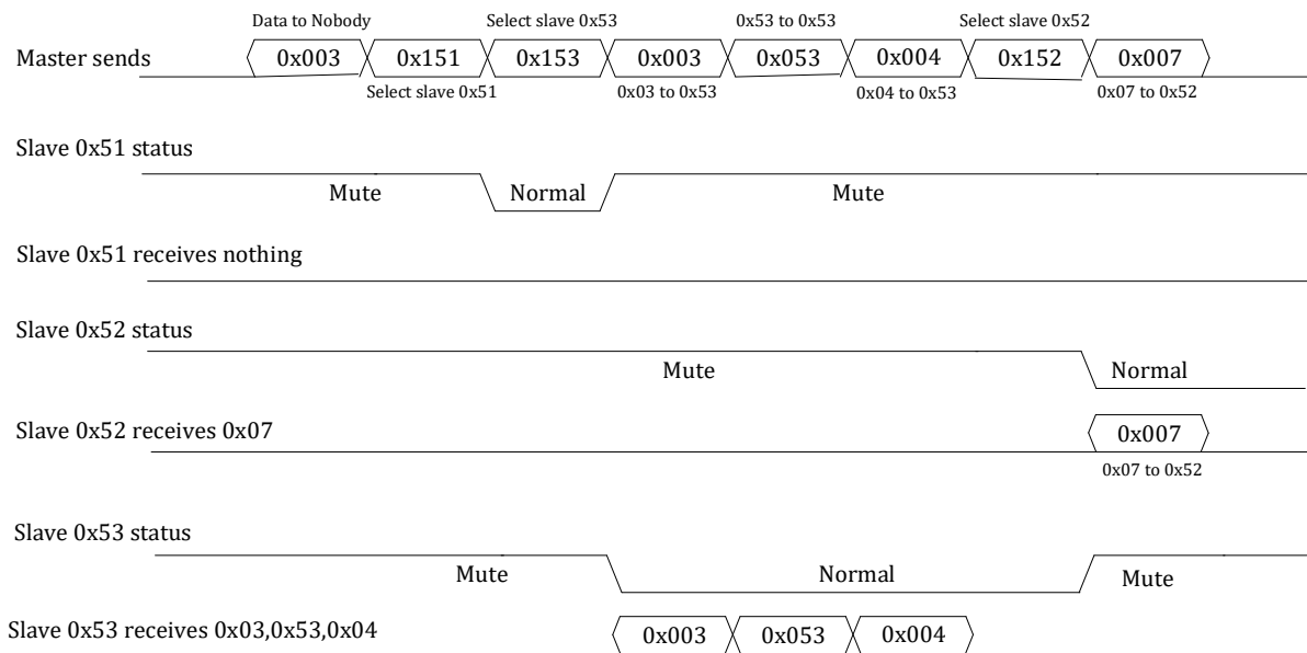
图 17-5 UART 多机通讯示例
