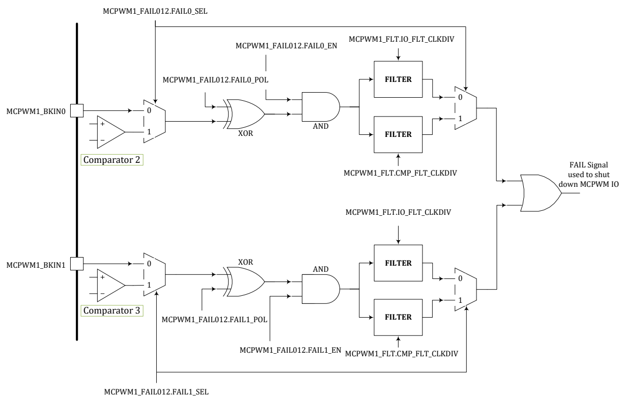
图 16-7 MCPWM1 FAIL0/1 逻辑示意图
