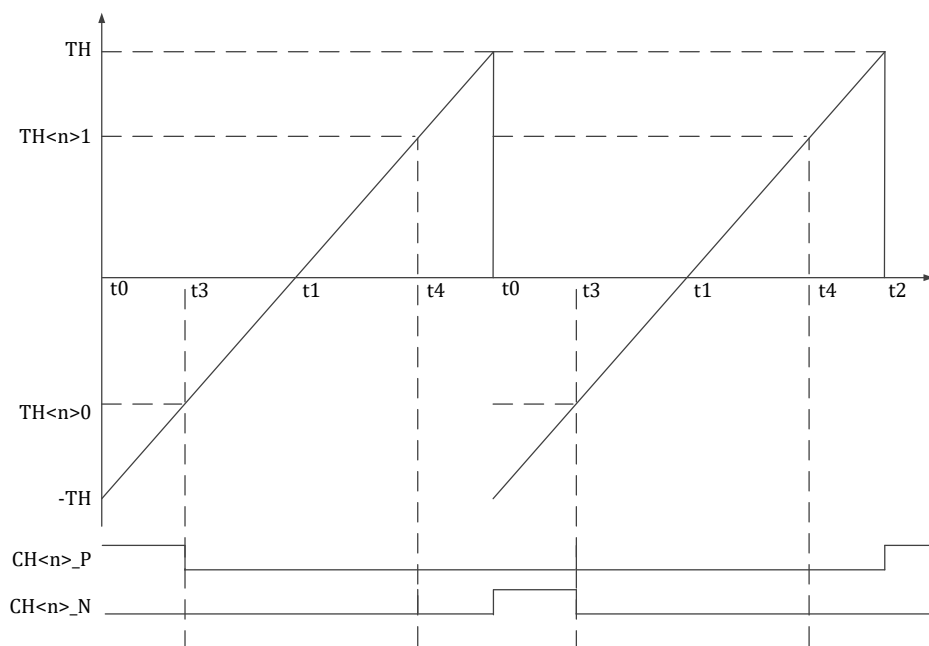
图 16-14MCPWM 时序 TH&lt;n&gt;0 和 TH&lt;n&gt;1 边沿对齐推挽模式
