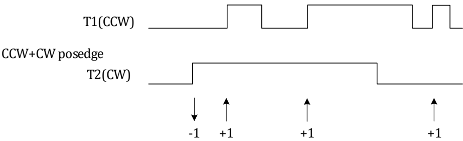
图 14-10 编码器仅在 T1/T2 上升沿计数的 CCW/CW 双脉冲信号计数情况
