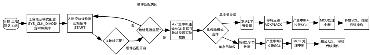
图 18-4 I2C 从模式工作流程图
