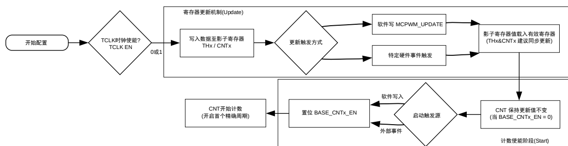
图 16-4 时基寄存器更新与计数使能流程图
