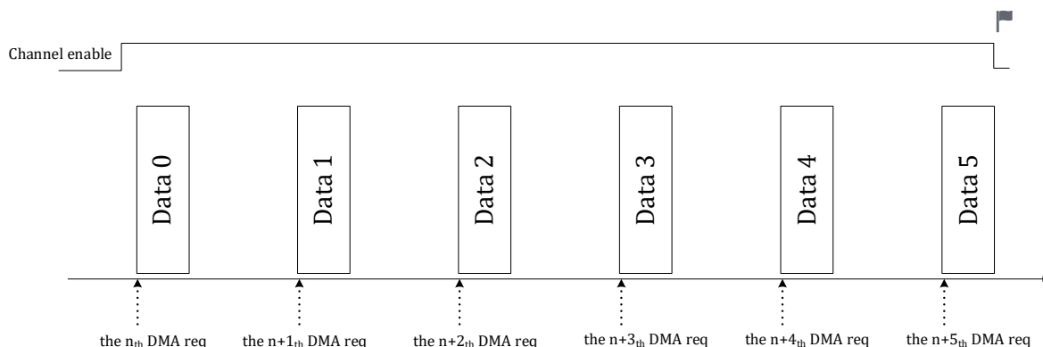
图 8-3 RMODE=1 DMA 传输情况
