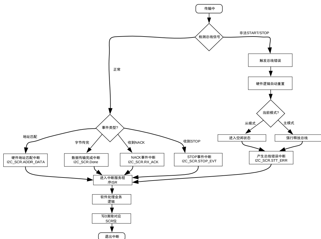
图 18-9 I2C 总线错误处理及中断管理流程图
