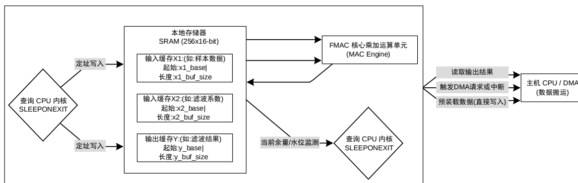
图 12-2 FMAC 硬件乘加运算单元整体架构框图
