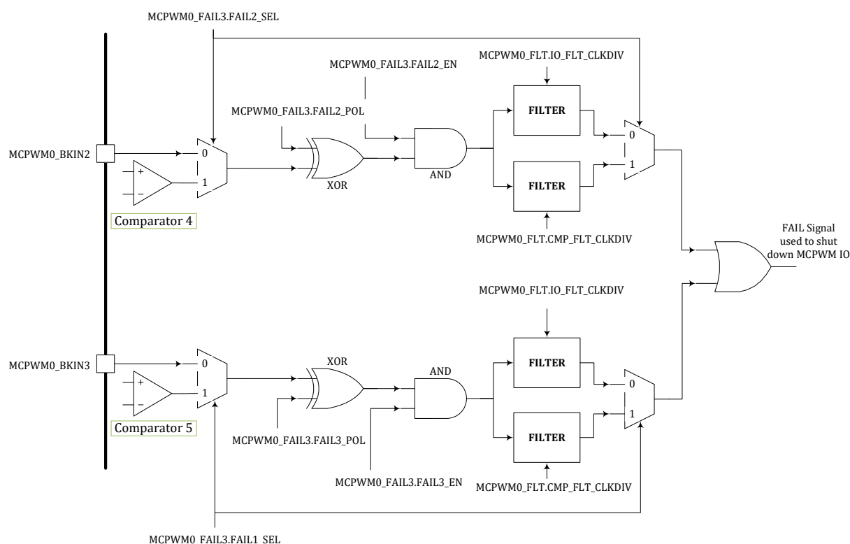
图 16-6 MCPWM0 FAIL2/3 逻辑示意图
