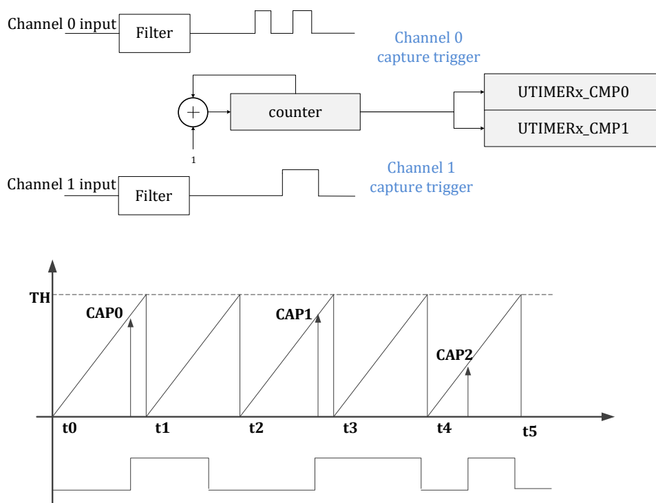
图 14-5 UTimer 捕获模式
