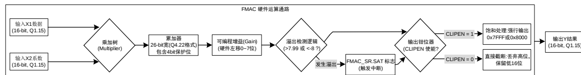
图 12-11 FMAC 硬件乘加运算内核流水线通路
