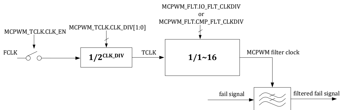
图 16-9 MCPWM Fail 信号滤波时钟生成逻辑
