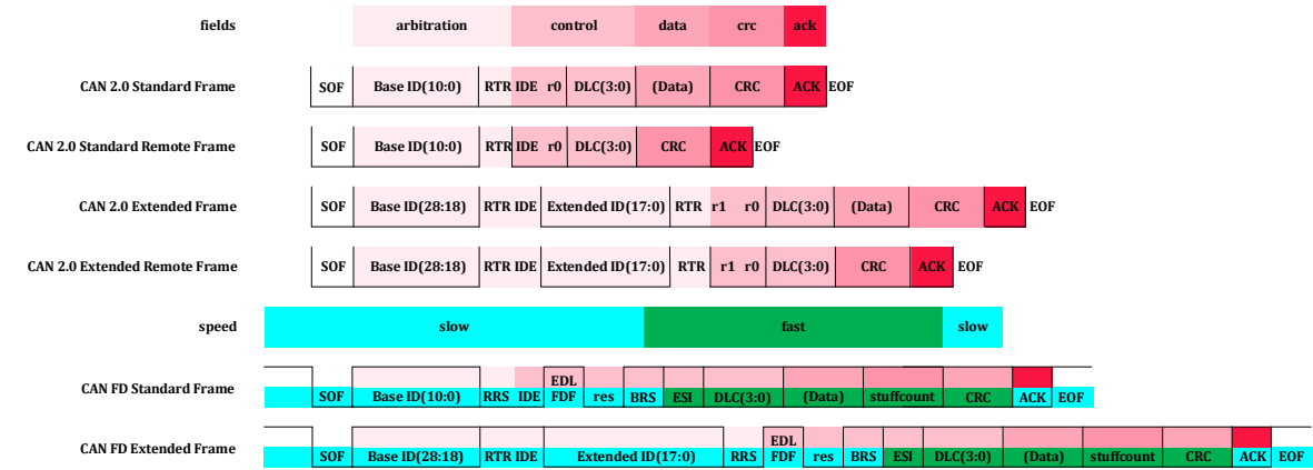
图 21-7 CAN 2.0 和 CAN FD 帧类型
