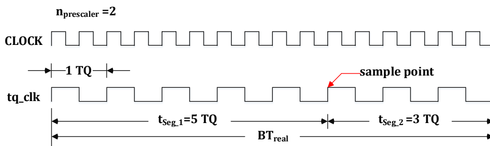
图 21-17 位采样时钟分频示例
