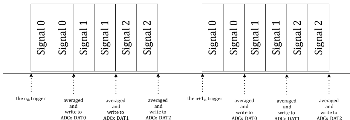
图 13-5 过采样转换时序示例 1
