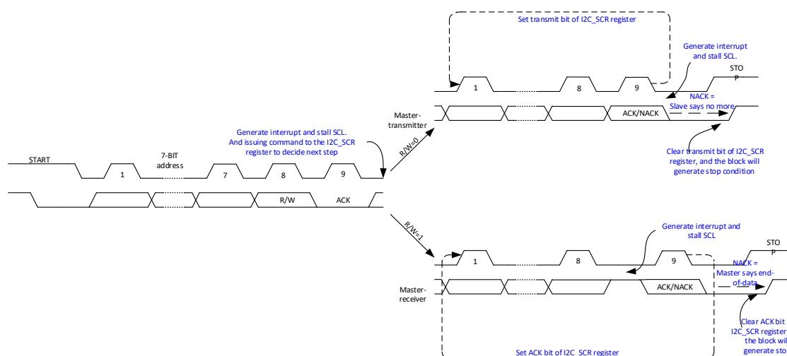
图 18-7 主模式下单字节传输示意图
