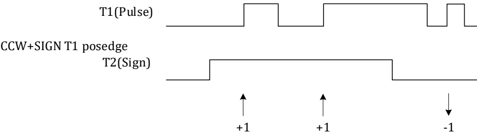
图 14-9 编码器在仅 T1 上升沿计数的符号加脉冲信号计数情况
