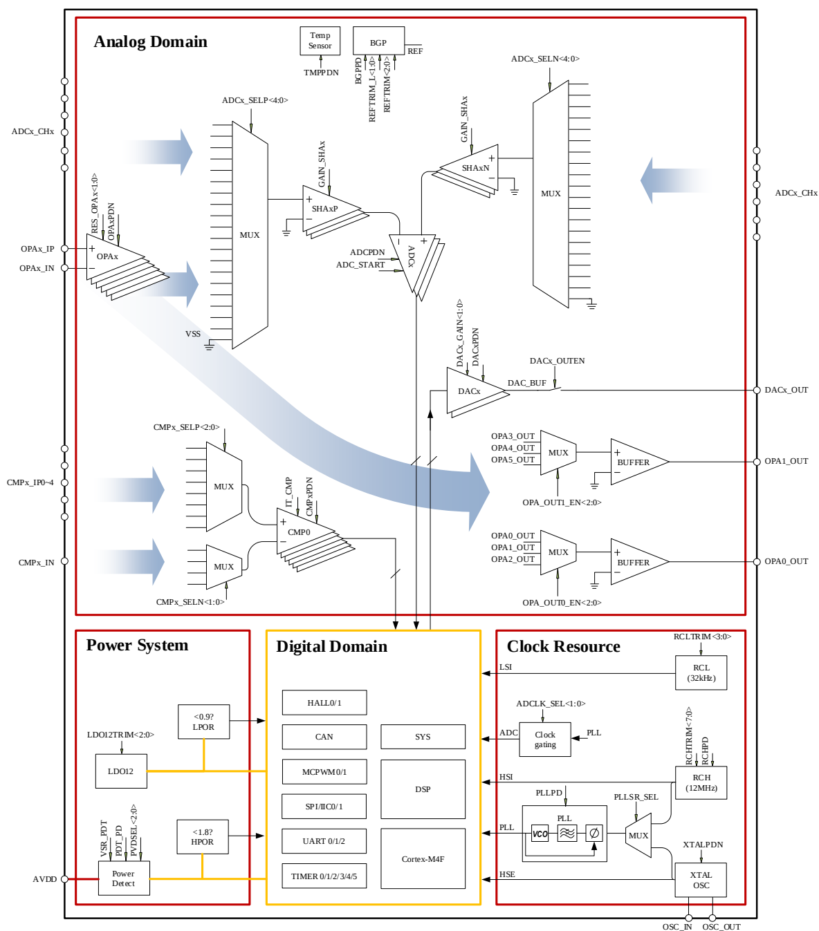
图 5-1 模拟电路功能框图
