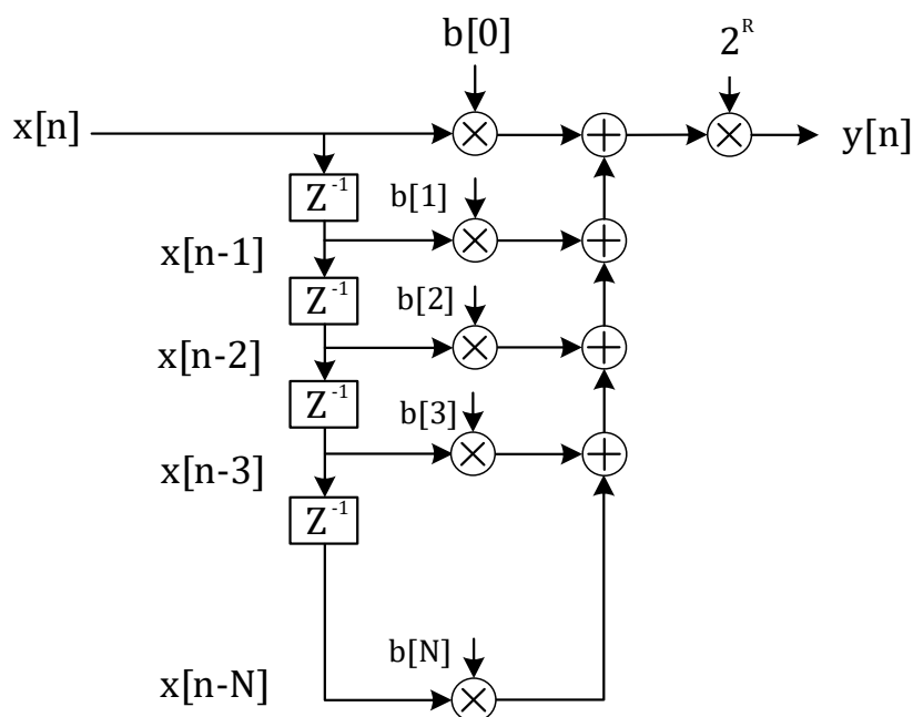
图 12-9 FIR 滤波器结构
