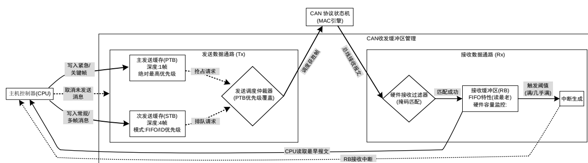
图 21-4 CAN 控制器数据通路架构图
