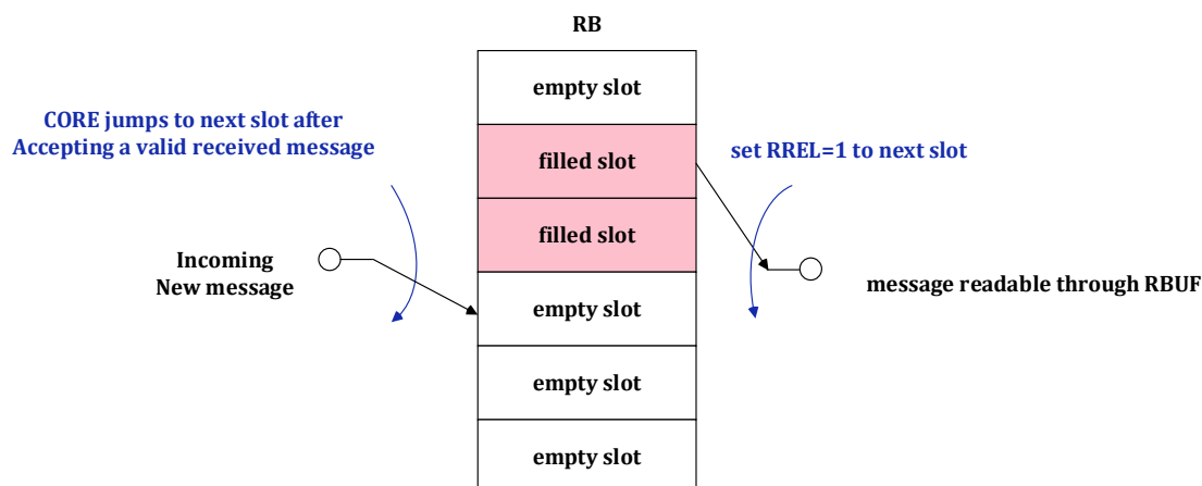
图 21-12 类似 FIFO 的 RB 示意图（6 个消息槽的示例）
