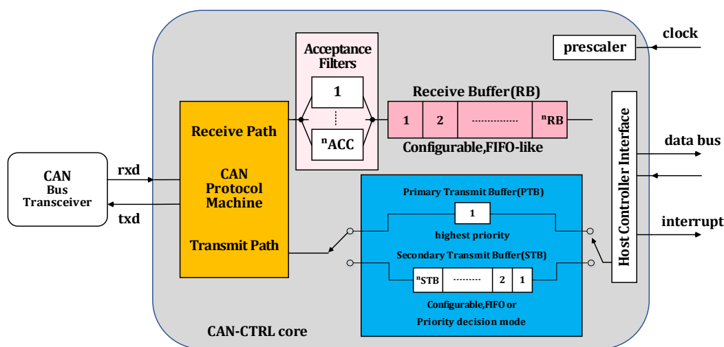
图 21-3 消息缓冲区
