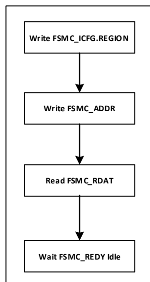
图 7-3 On-Chip FLASH 间接读取操作流程
