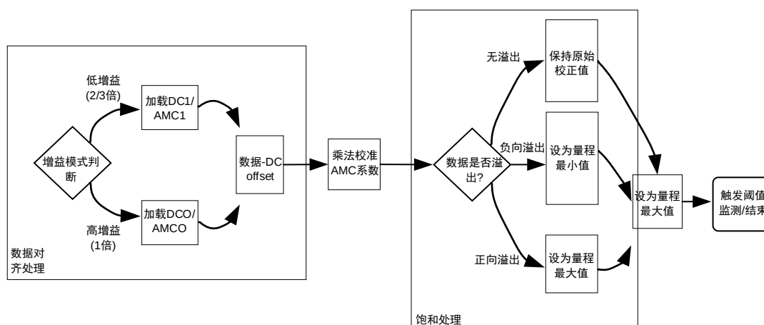
图 13-8 ADC 自动校准逻辑流程图
