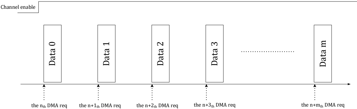
图 8-5 CIRC=1 且 RMODE=1 DMA 传输情况
