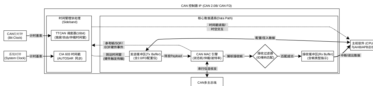
图 21-2 CAN 控制器数据通路与时间管理架构图
