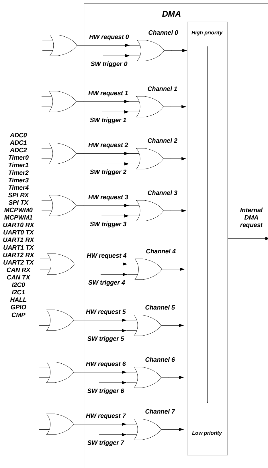
图 8-8 DMA 通道优先级
