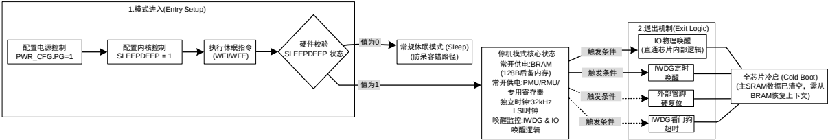
图 24-3 停机/待机模式进入与冷启动退出流程图
