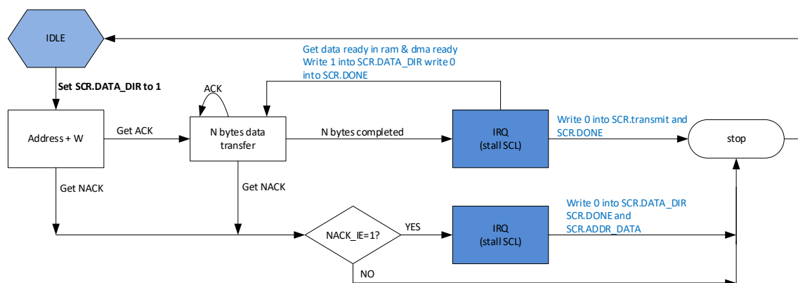
图 18-11 主模式下多字节发送示意图
