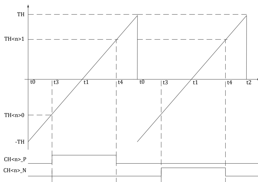
图 16-12 MCPWM 时序 TH_{<n>0} 和 TH_{<n>1} -中心对齐推挽模式
