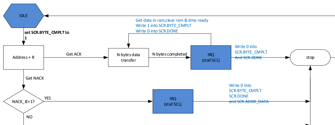
图 18-12 主模式下多字节接收示意图
