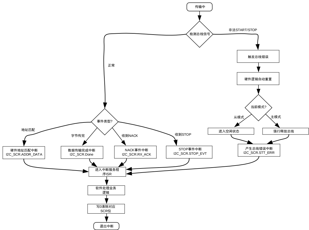
图 18-14 I2C 总线错误处理及中断管理流程图
