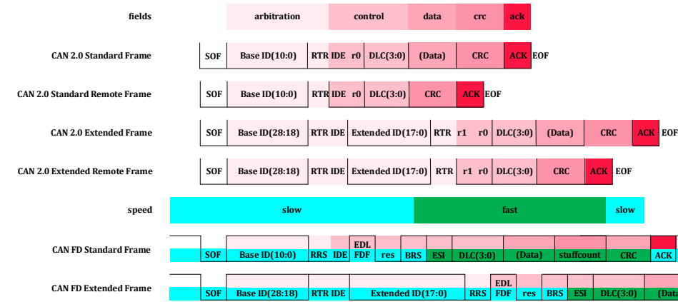
图 21-7 CAN 2.0 和 CAN FD 帧类型
