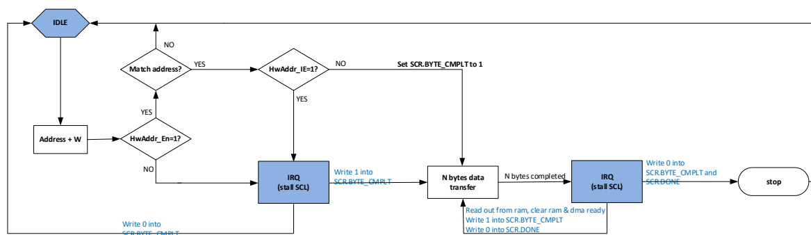
图 18-8 从模式下多字节接收示意图
