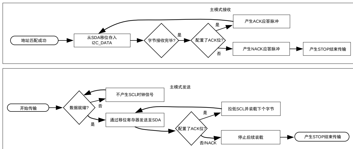
图 18-10 I2C 主模式发送和接收的逻辑流程图
