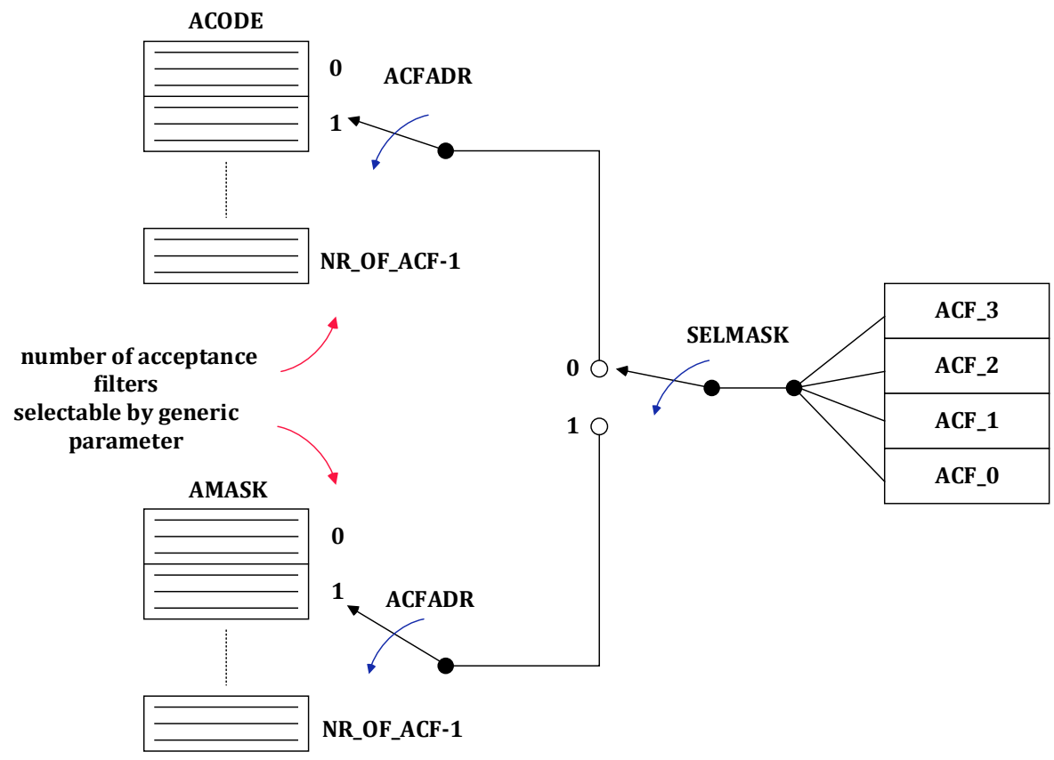
图 21-10 接收过滤器
