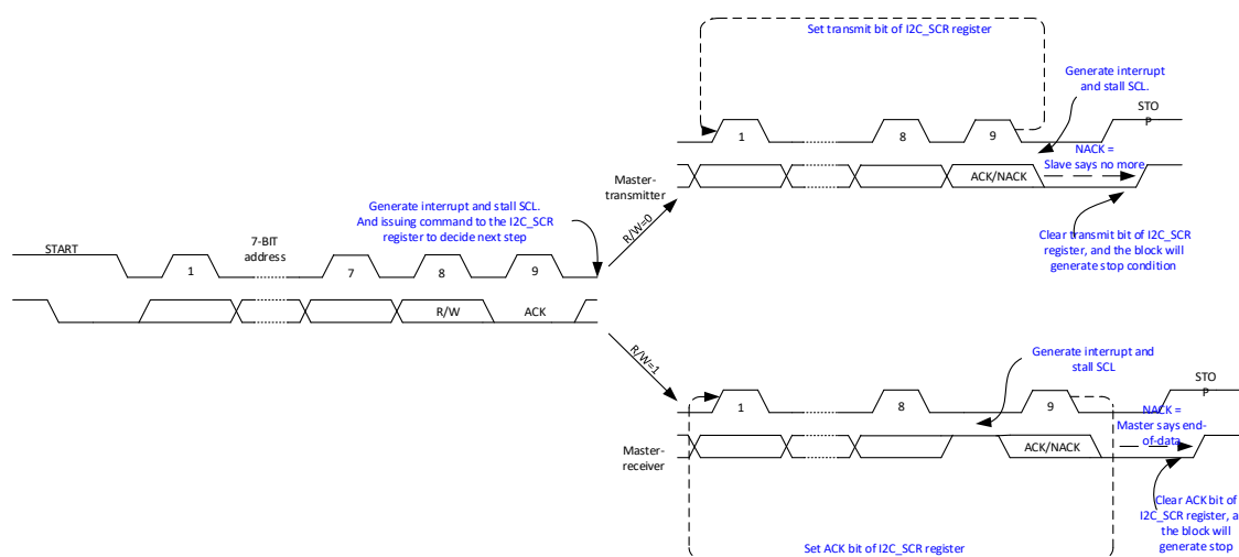
图 18-9 主模式下单字节传输示意图
