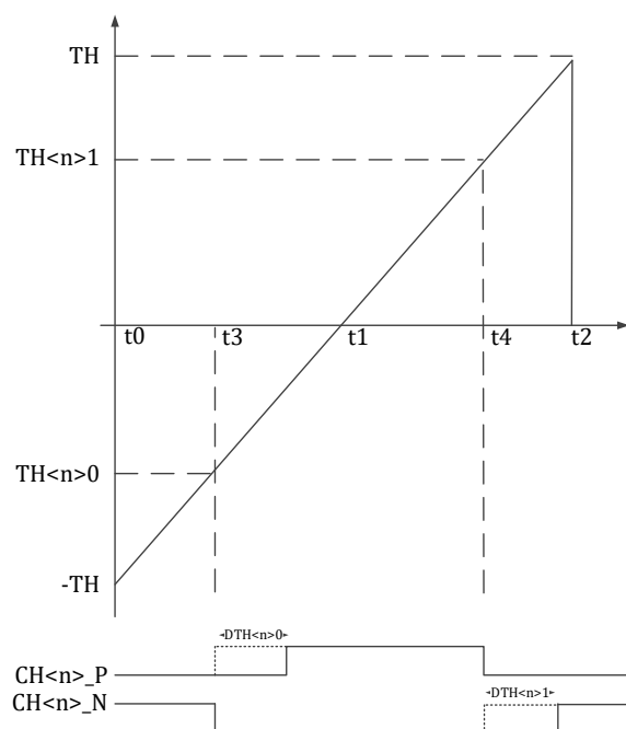
图 16-11 MCPWM 时序 TH_{<n>0} 和 TH_{<n>1} -中心对齐模式
